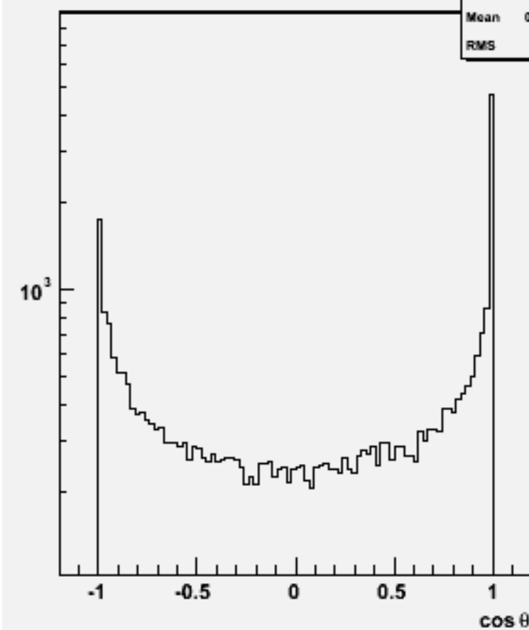
Jet cos \theta (All jets)w102296 n3n3e2e2e2e2_o
