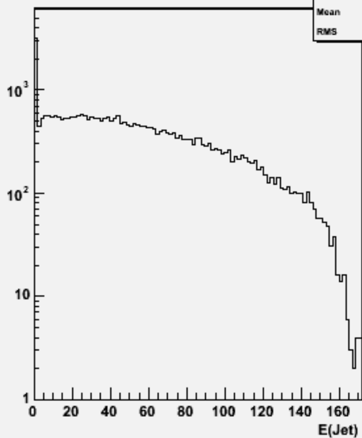
Jet energies(All jets)w102296 n3n3e2e2e2e2_o
