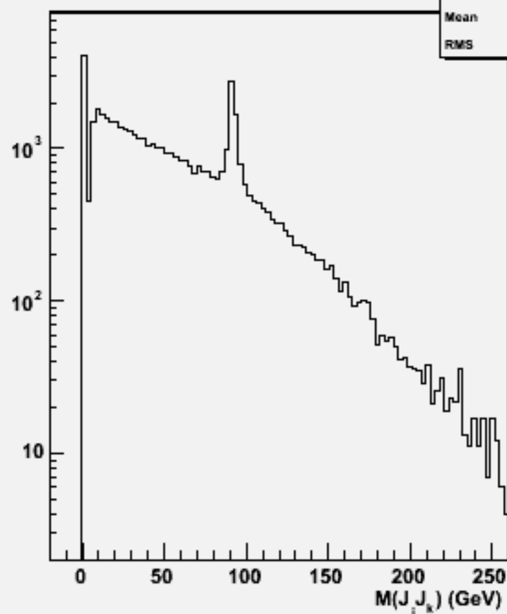
2jets mass(All comb)w102296 n3n3e2e2e2e2_o
