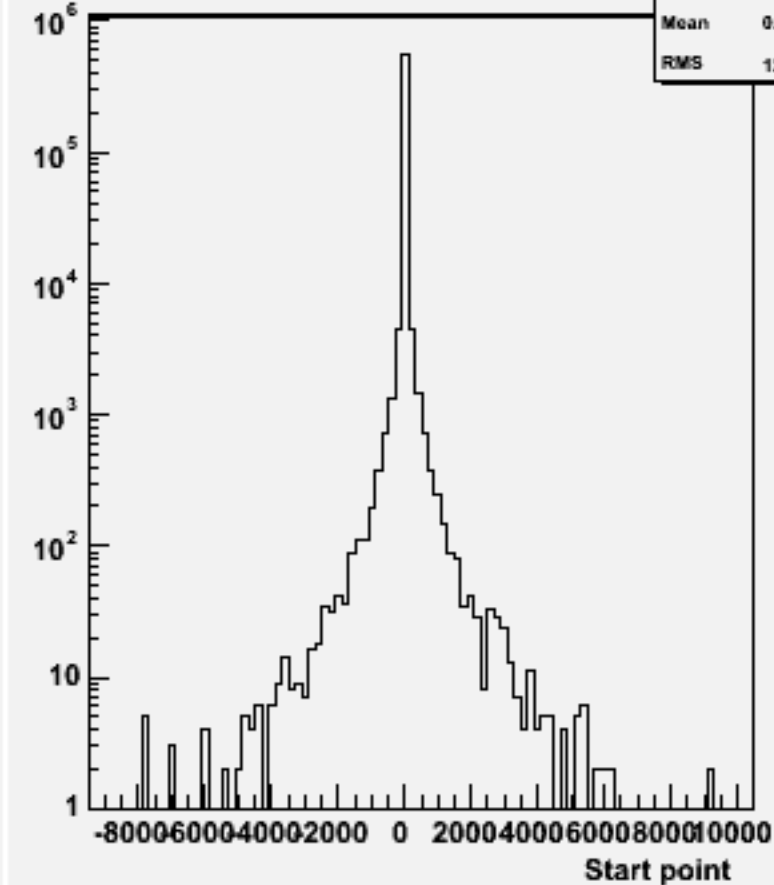
Start point Z : w102293 n3n3e1e1bb_o
