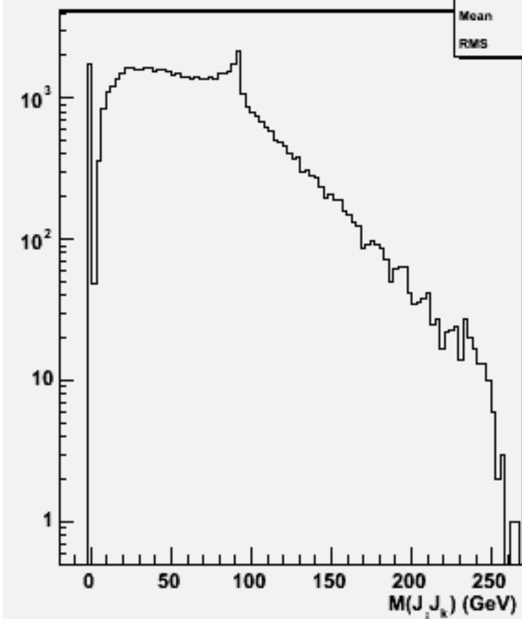
2jets mass(All comb)w102293 n3n3e1e1bb_o
