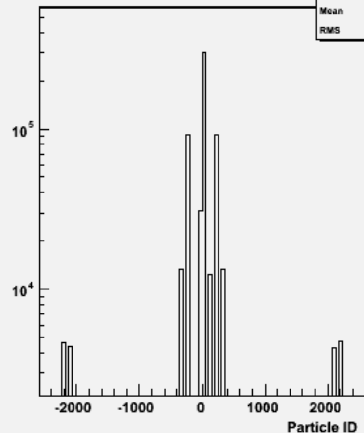
Particle ID : w102293 n3n3e1e1bb_o
