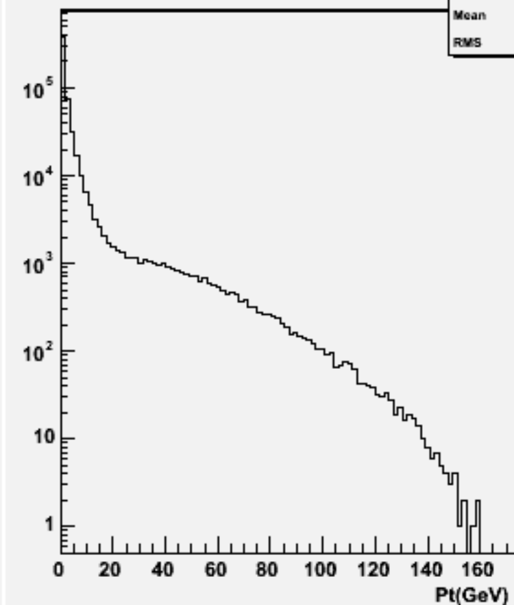
Particle Pt : w102293 n3n3e1e1bb_o
