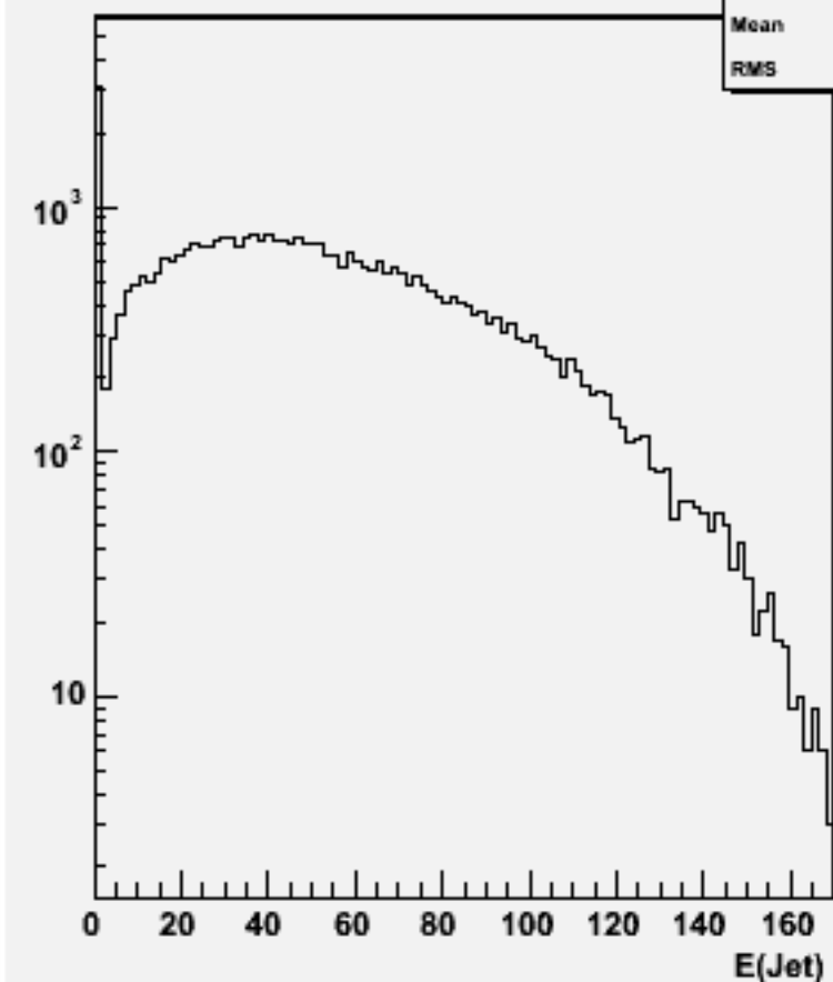
Jet energies(All jets)w102293 n3n3e1e1bb_o
