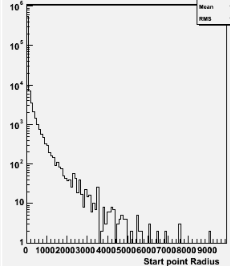
Start point R : w102293 n3n3e1e1bb_o
