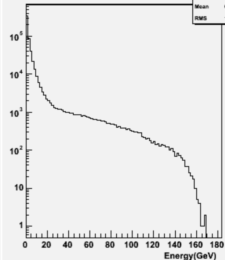
Particle Energy : w102293 n3n3e1e1bb_o
