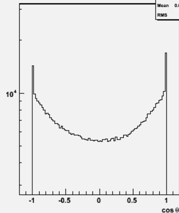
Particle cos \theta : w102293 n3n3e1e1bb_o
