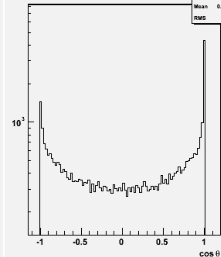
Jet cos \theta (All jets)w102293 n3n3e1e1bb_o
