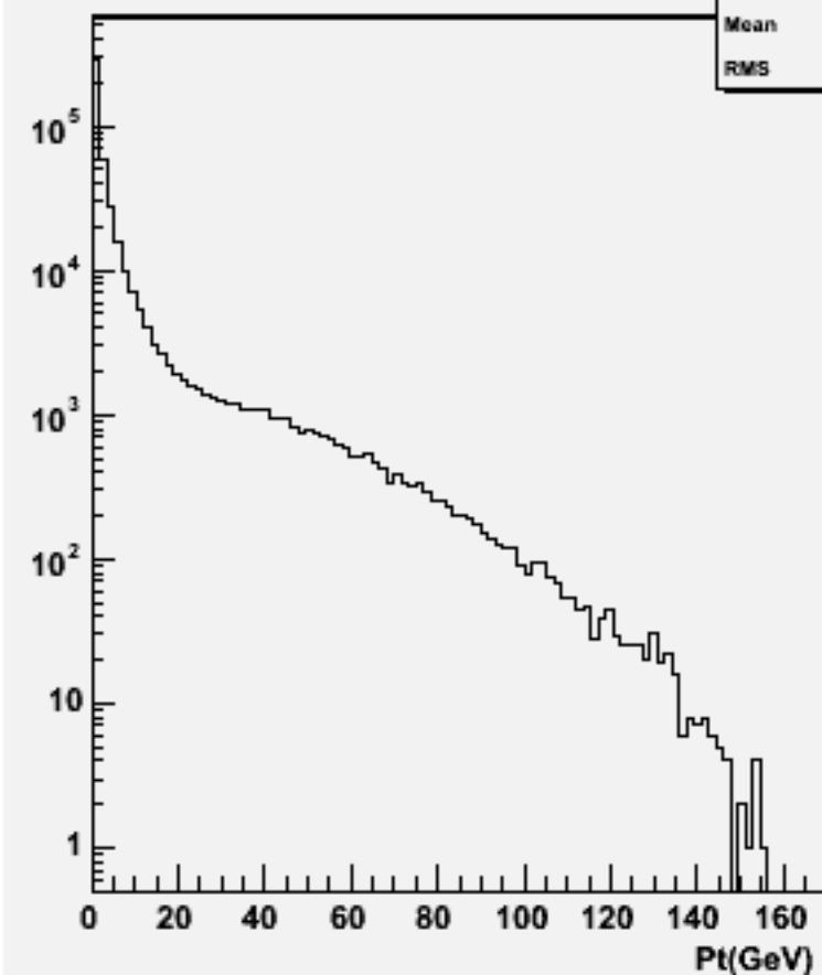
Particle Pt : w102288 n3n3e1e1ss_o
