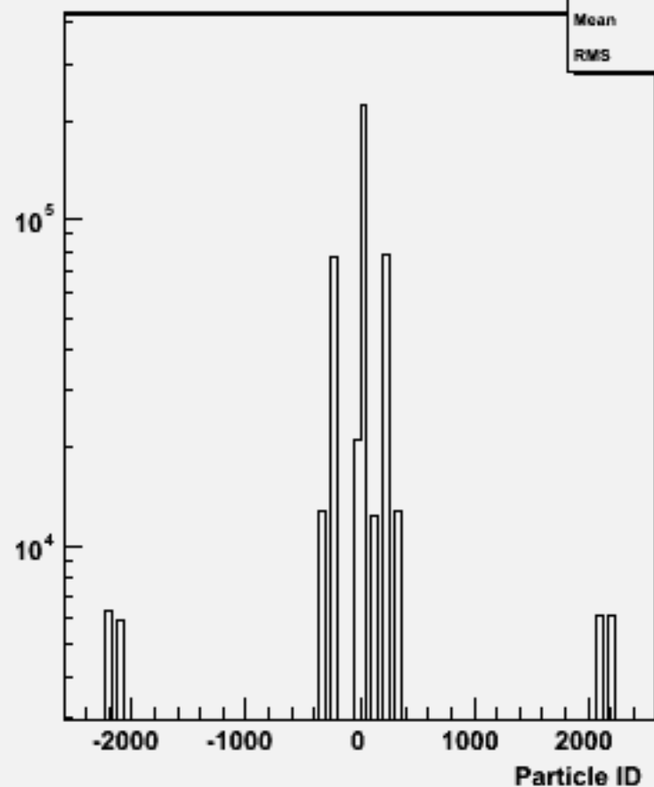
Particle ID : w102288 n3n3e1e1ss_o
