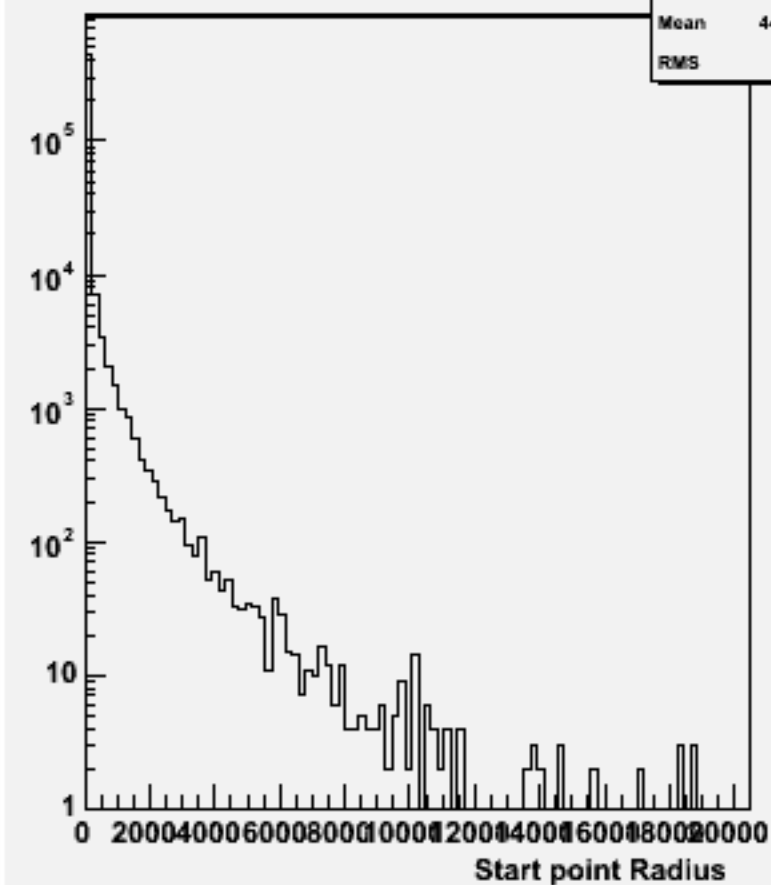
Start point R : w102288 n3n3e1e1ss_o
