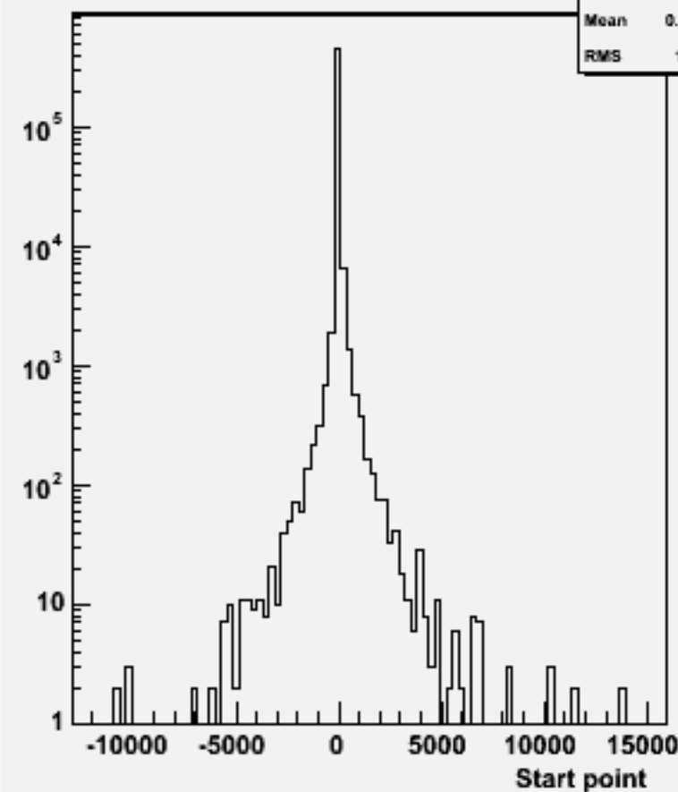
Start point Z : w102285 n3n3e1e1dd_o
