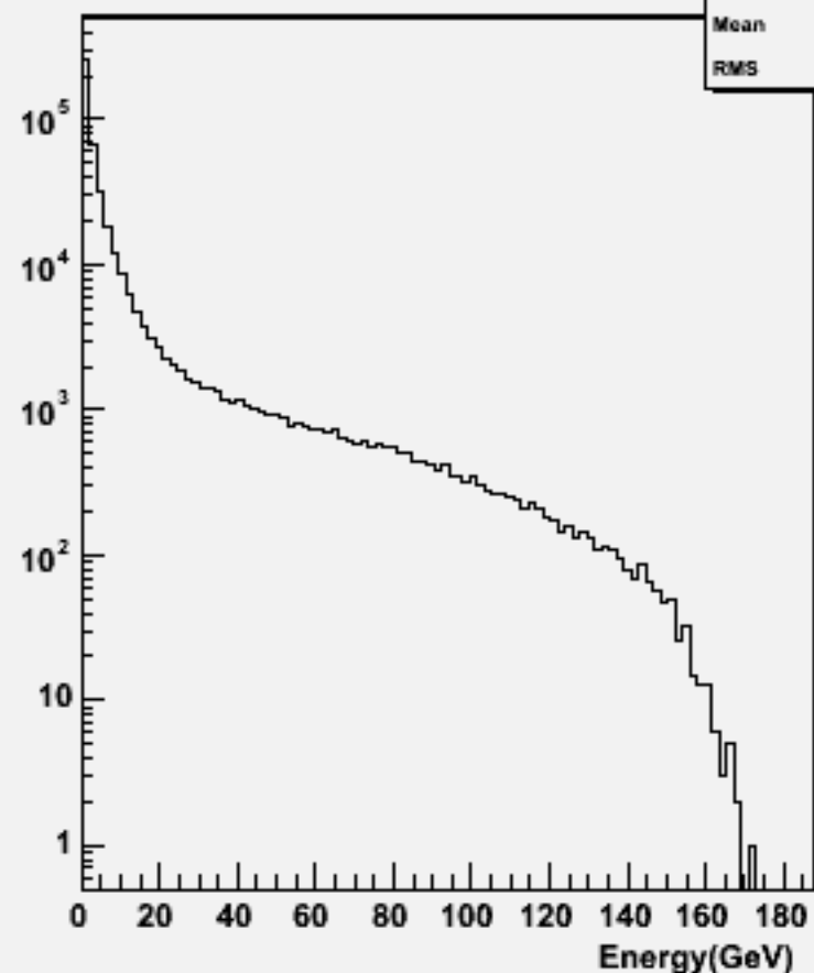
Start point R : w102285 n3n3e1e1dd_o
