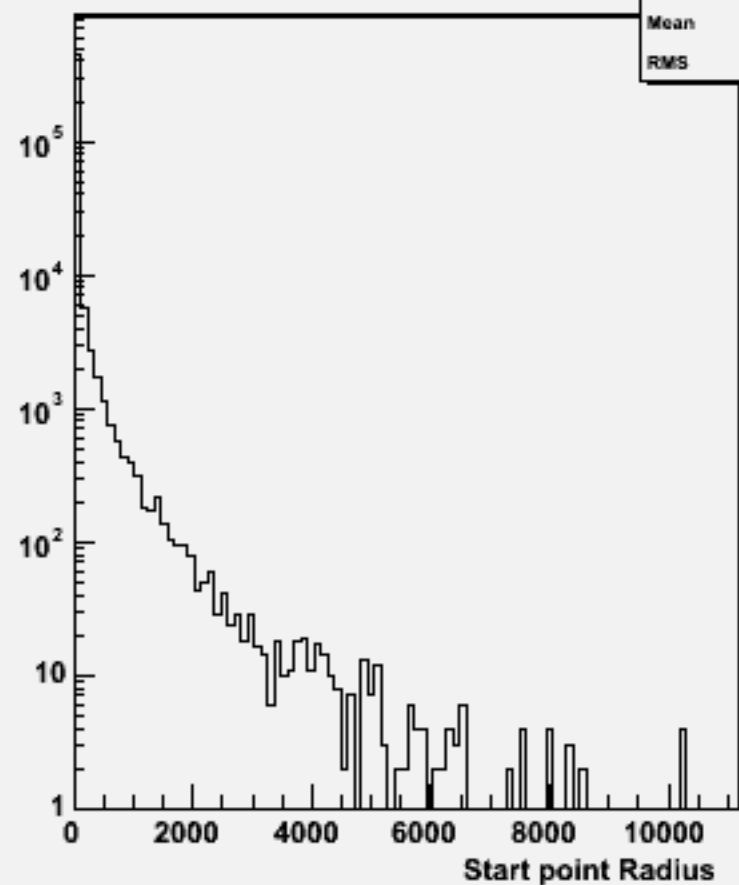
Start point R : w102285 n3n3e1e1dd_o
