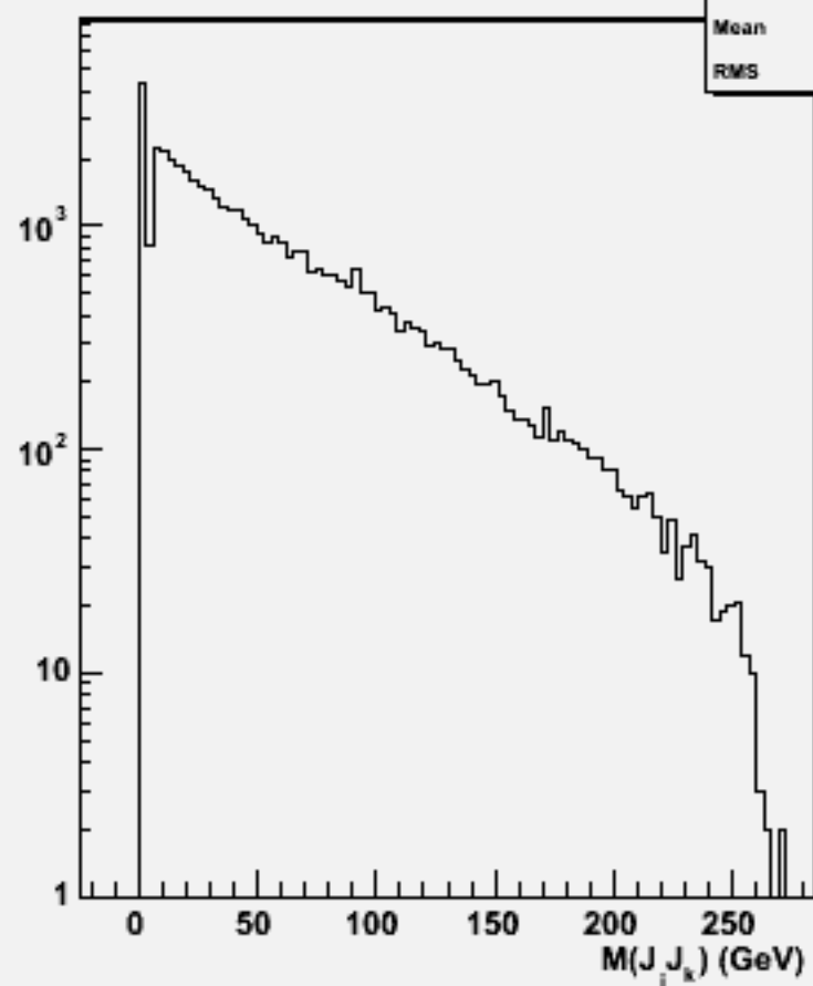
2jets mass(All comb)w102282 n3n3e1e1e2e2_o
