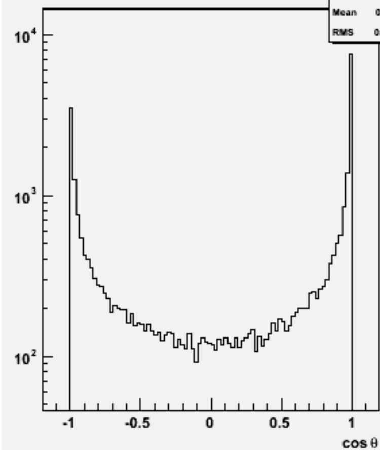
Jet cos \theta (All jets)w102282 n3n3e1e1e2e2_o
