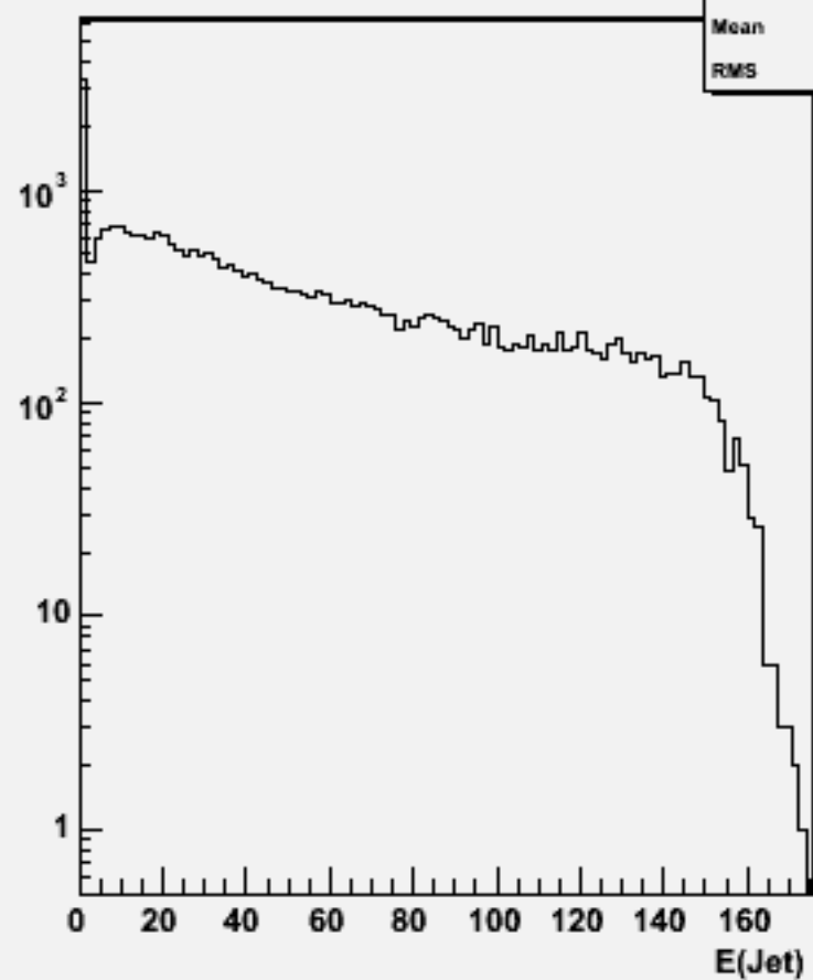
Jet energies(All jets)w102282 n3n3e1e1e2e2_o
