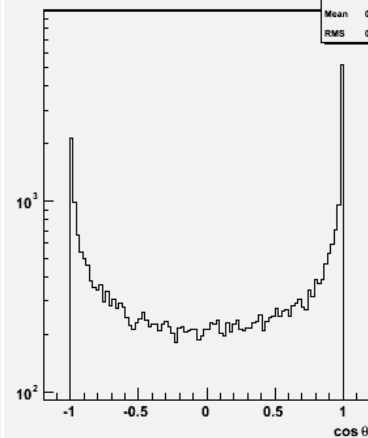
Jet cos \theta (All jets)w102280 n3n3e1e1e2e2_o
