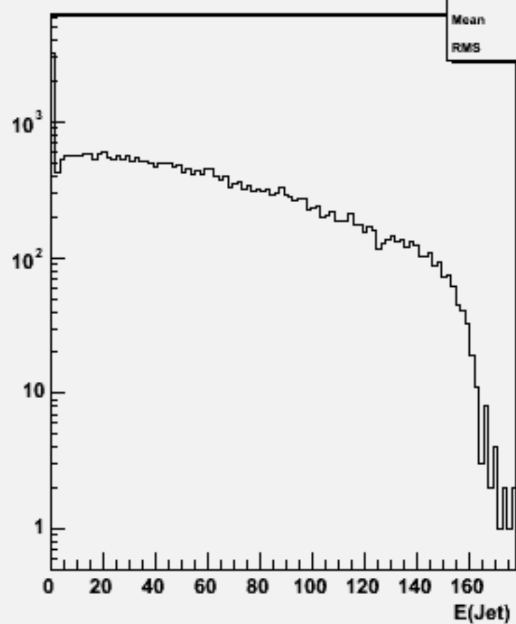
Jet energies(All jets)w102280 n3n3e1e1e2e2_o
