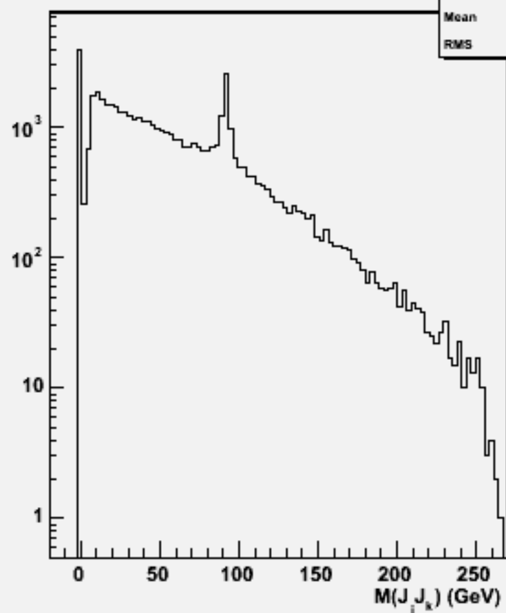
2jets mass(All comb)w102280 n3n3e1e1e2e2_o
