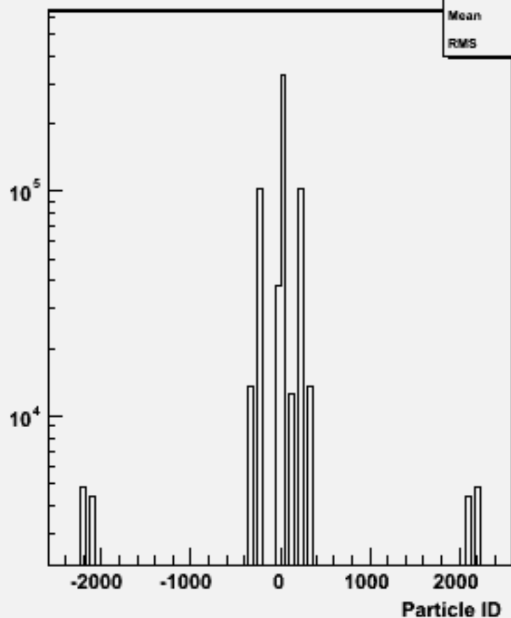
Particle ID : w102249 n2n2e3e3bb_o
