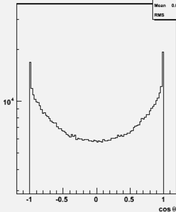
Particle cos \theta : w102249 n2n2e3e3bb_o
