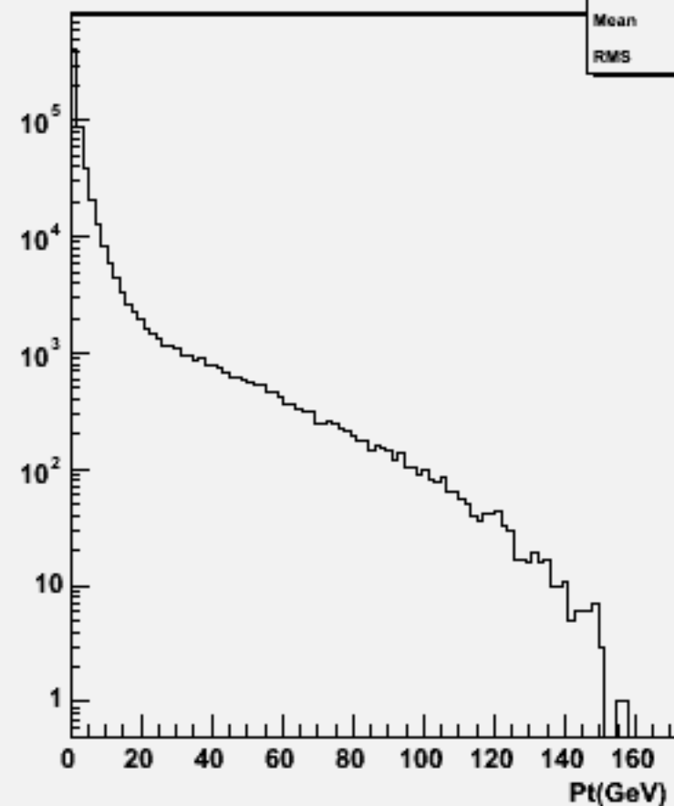
Particle Pt : w102249 n2n2e3e3bb_o
