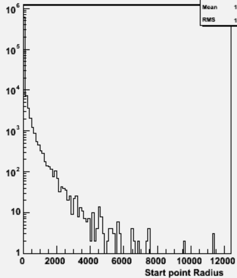
Start point R : w102248 n2n2e3e3bb_o
