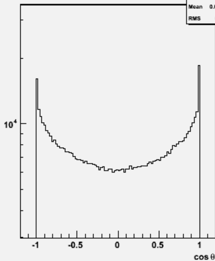
Particle cos \theta : w102248 n2n2e3e3bb_o
