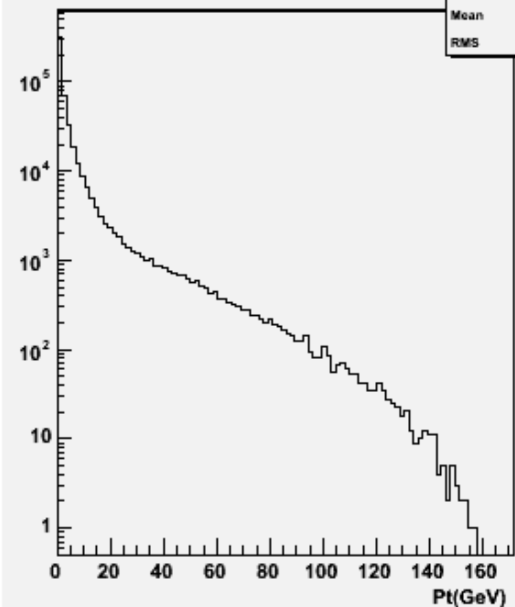
Particle Pt : w102245 n2n2e3e3ss_o
