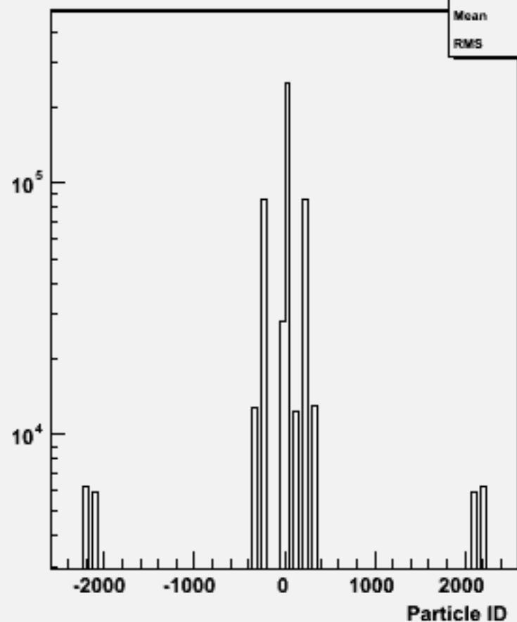
Particle ID : w102245 n2n2e3e3ss_o
