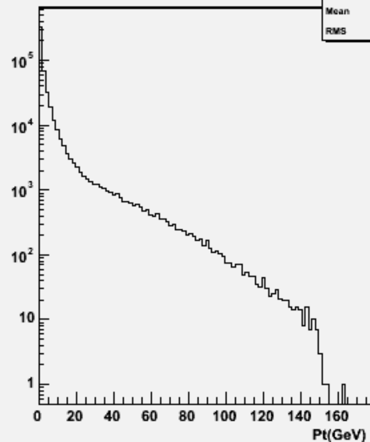
Particle Pt : w102241 n2n2e3e3dd_o
