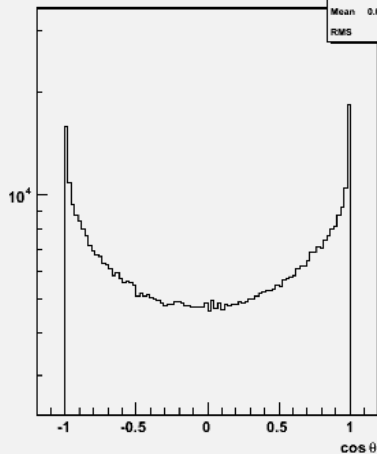
Particle cosθ : w102241 n2n2e3e3dd_o
