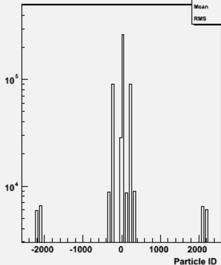
Particle ID : w102241 n2n2e3e3dd_o
