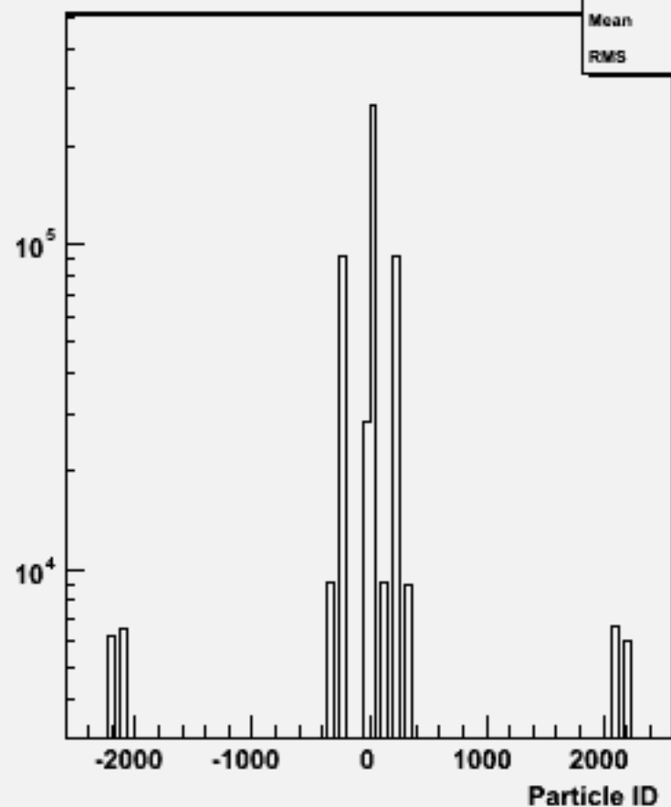
Particle ID : w102240 n2n2e3e3dd_o
