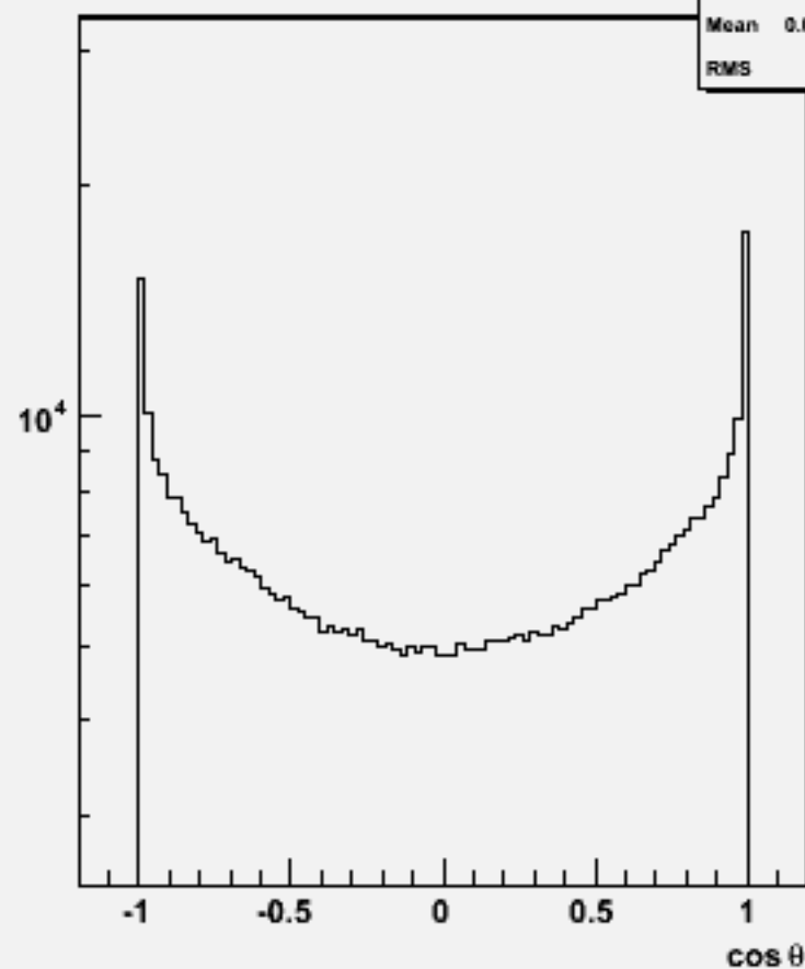
Particle cosθ : w102240 n2n2e3e3dd_o
