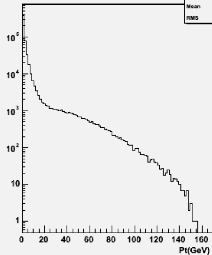
Particle Pt : w102233 n2n2e1e1bb_o
