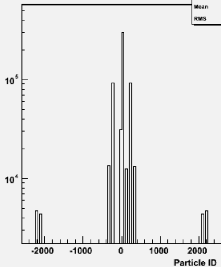
Particle ID : w102233 n2n2e1e1bb_o
