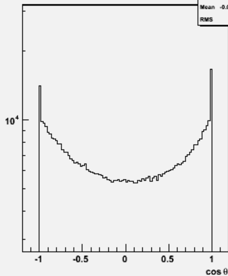
Particle cos \theta : w102233 n2n2e1e1bb_o
