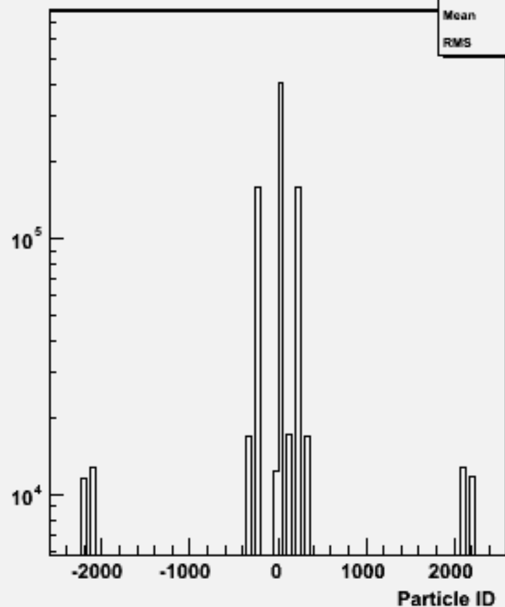
Particle ID : w102193 n1n1dddd_o
