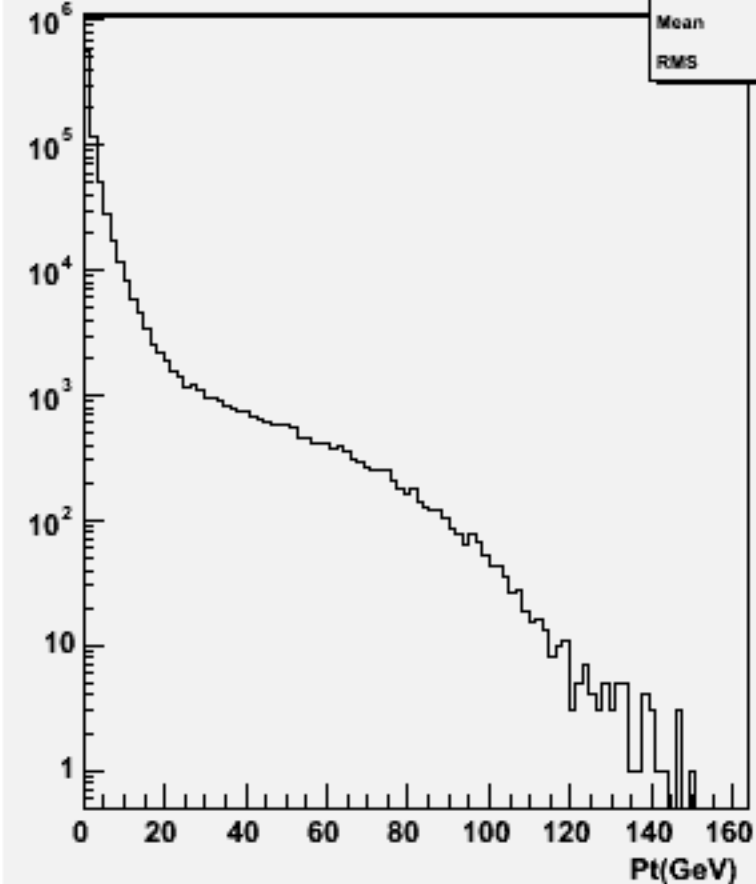
Particle Pt : w102193 n1n1dddd_o
