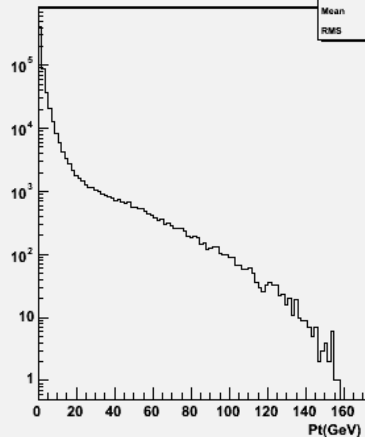
Particle Pt : w102189 n1n1e3e3bb_o
