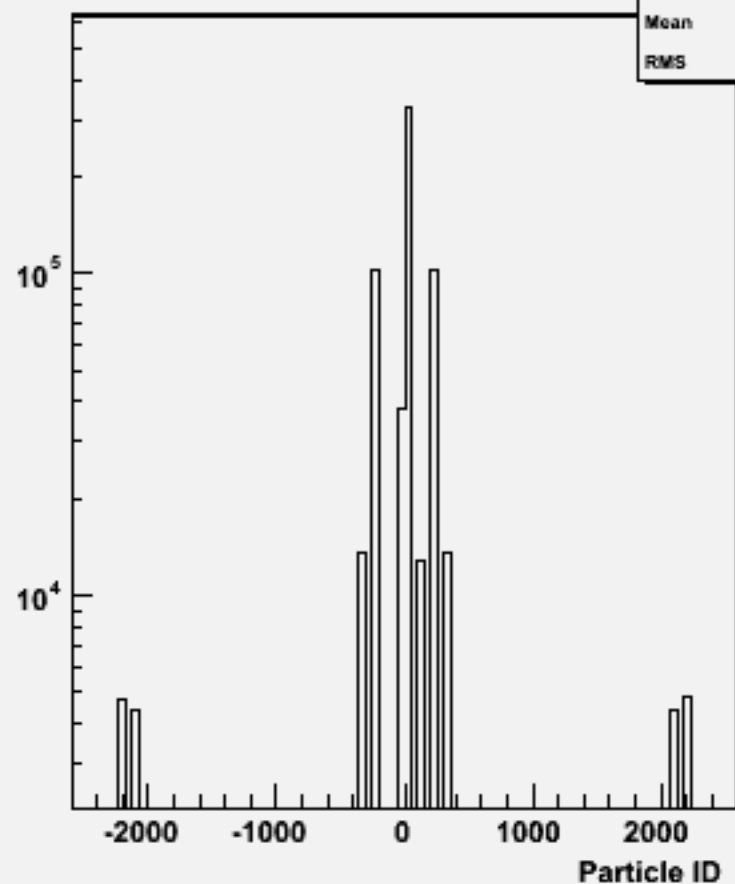
Particle ID : w102189 n1n1e3e3bb_o
