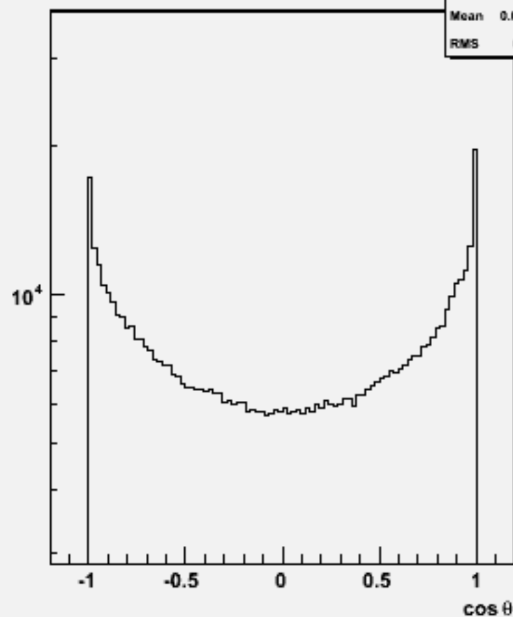
Particle cosθ : w102189 n1n1e3e3bb_o
