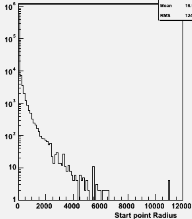
Start point R : w102189 n1n1e3e3bb_o
