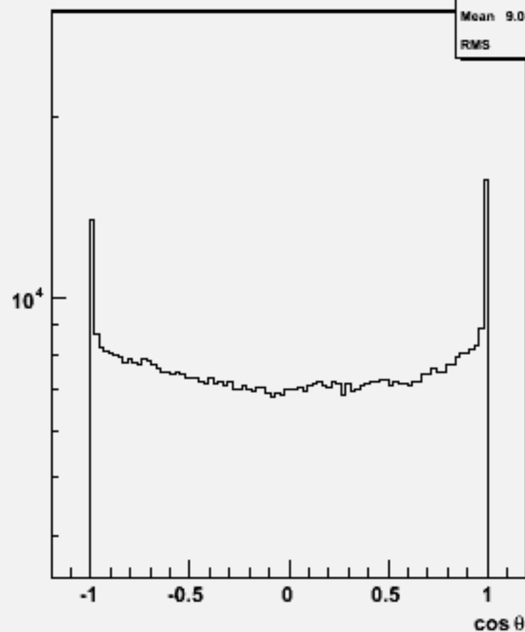
Particle cosθ : w102188 n1n1e3e3bb_o
