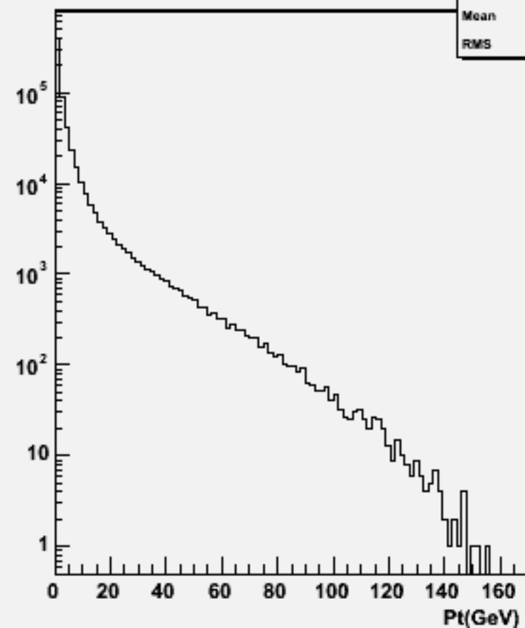
Particle Pt : w102188 n1n1e3e3bb_o
