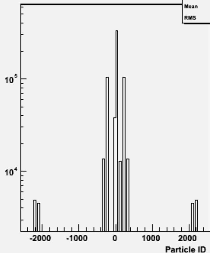
Particle ID : w102188 n1n1e3e3bb_o
