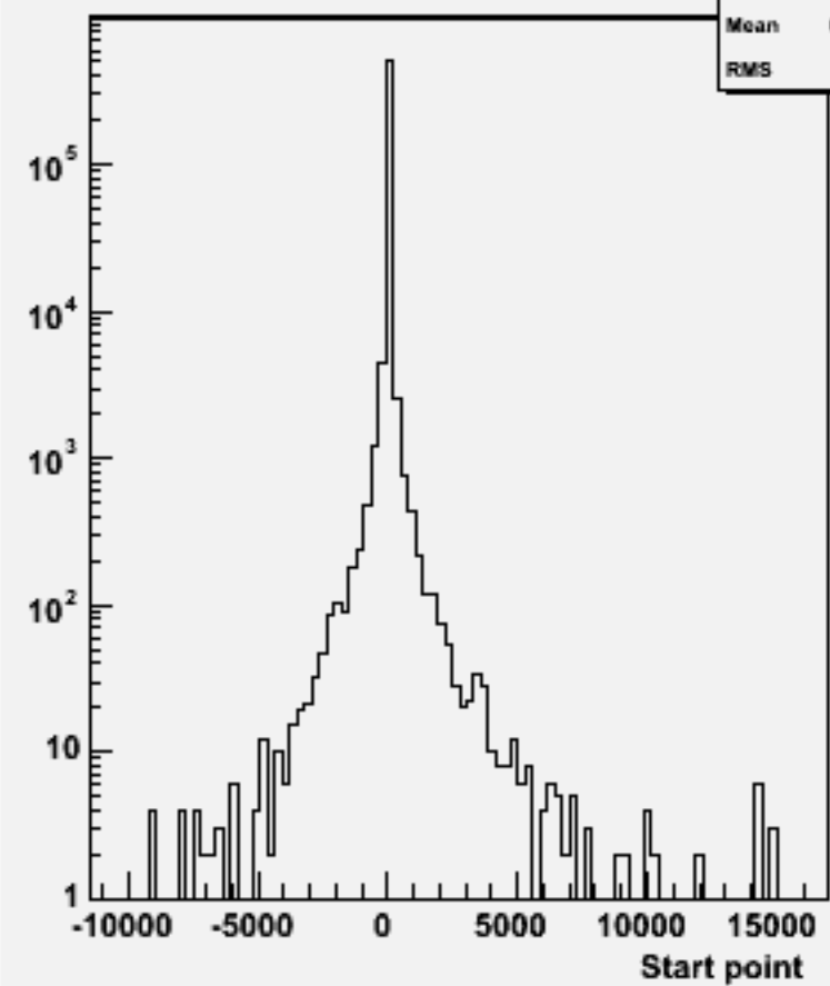
Start point Z : w102181 n1n1e3e3dd_o
