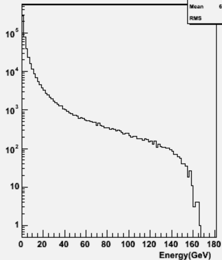
Start point R : w102181 n1n1e3e3dd_o
