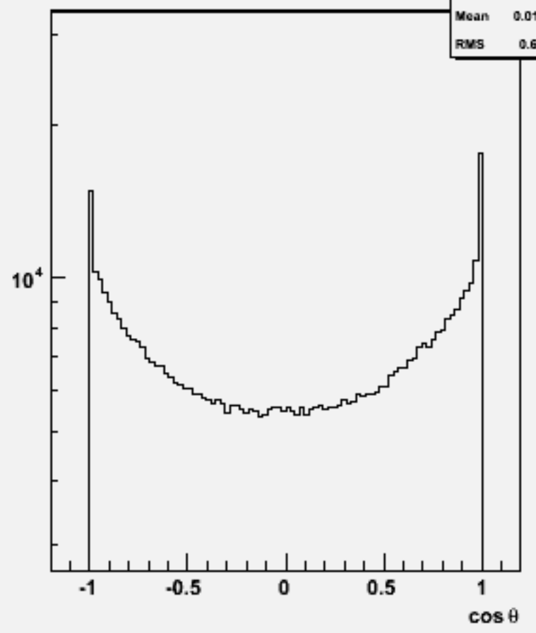
Particle cosθ : w102173 n1n1e2e2bb_o
