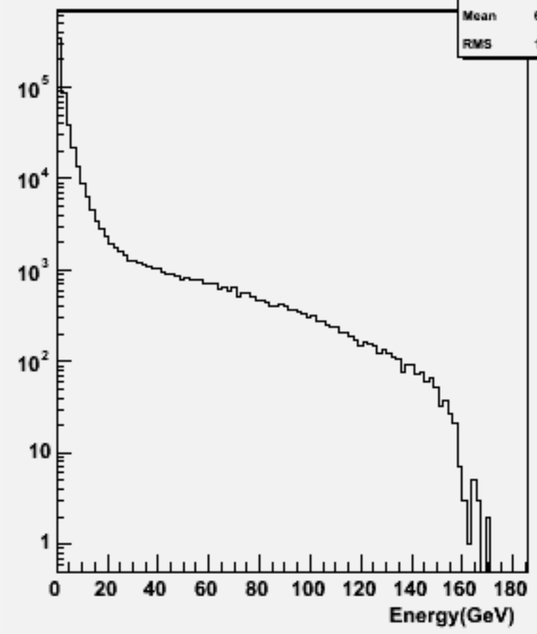
Start point R : w102173 n1n1e2e2bb_o
