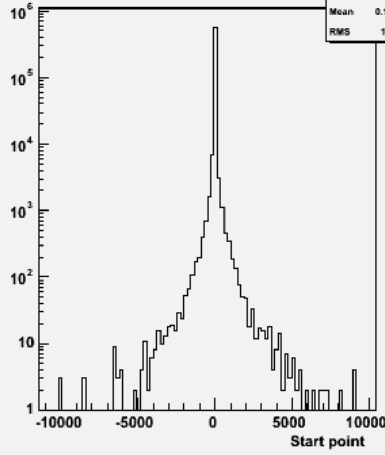
Start point Z : w102173 n1n1e2e2bb_o
