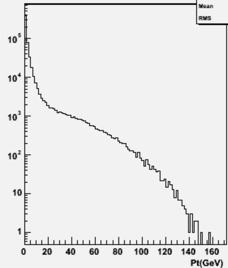
Particle Pt : w102172 n1n1e2e2bb_o
