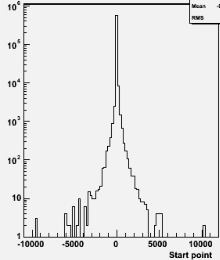
Start point Z : w102172 n1n1e2e2bb_o
