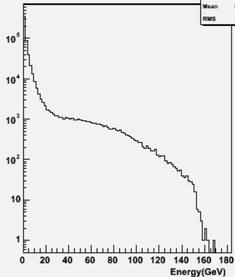
Particle Energy : w102172 n1n1e2e2bb_o
