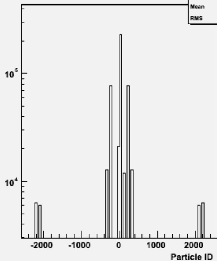
Particle ID : w102169 n1n1e2e2ss_o
