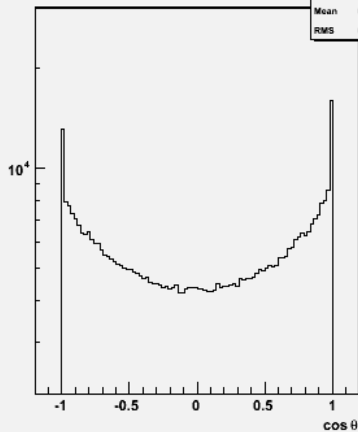
Particle cosθ : w102169 n1n1e2e2ss_o
