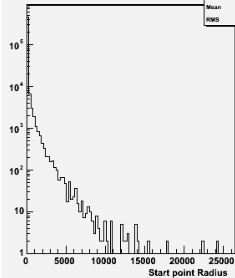
Start point R : w102169 n1n1e2e2ss_o
