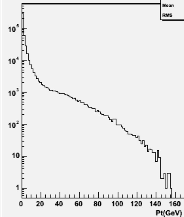
Particle Pt : w102169 n1n1e2e2ss_o
