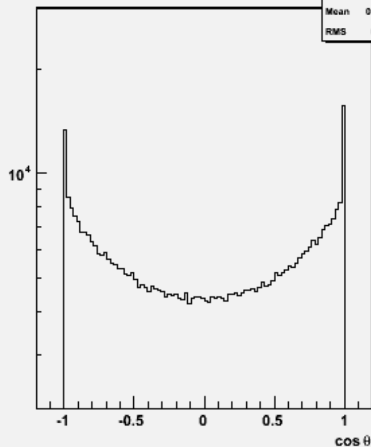
Particle cosθ : w102165 n1n1e2e2dd_o
