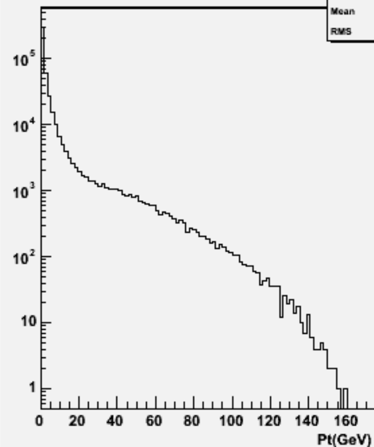
Start point Z : w102165 n1n1e2e2dd_o
