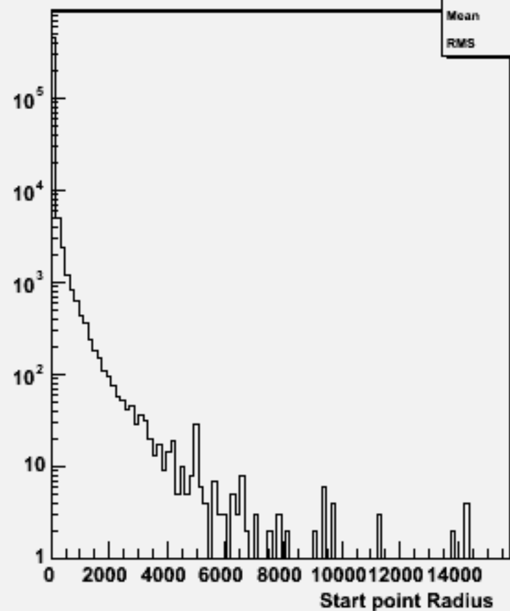
Start point R : w102165 n1n1e2e2dd_o
