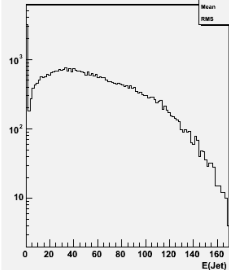
Jet energies(All jets)w102165 n1n1e2e2dd_o
