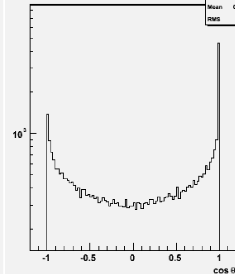
Jet cos \theta (All jets)w102165 n1n1e2e2dd_o
