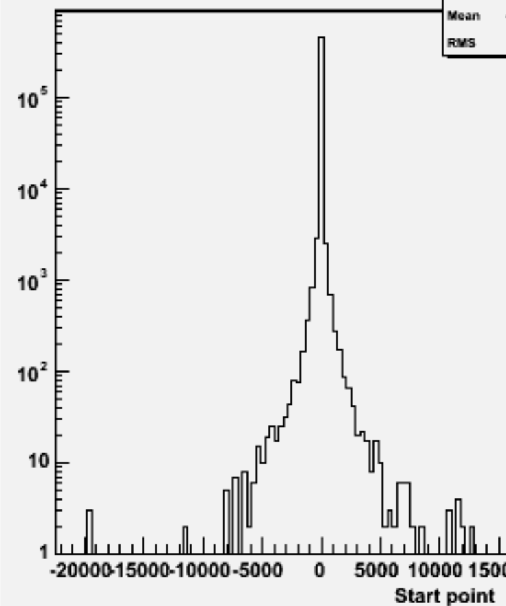
Start point Z : w102165 n1n1e2e2dd_o
