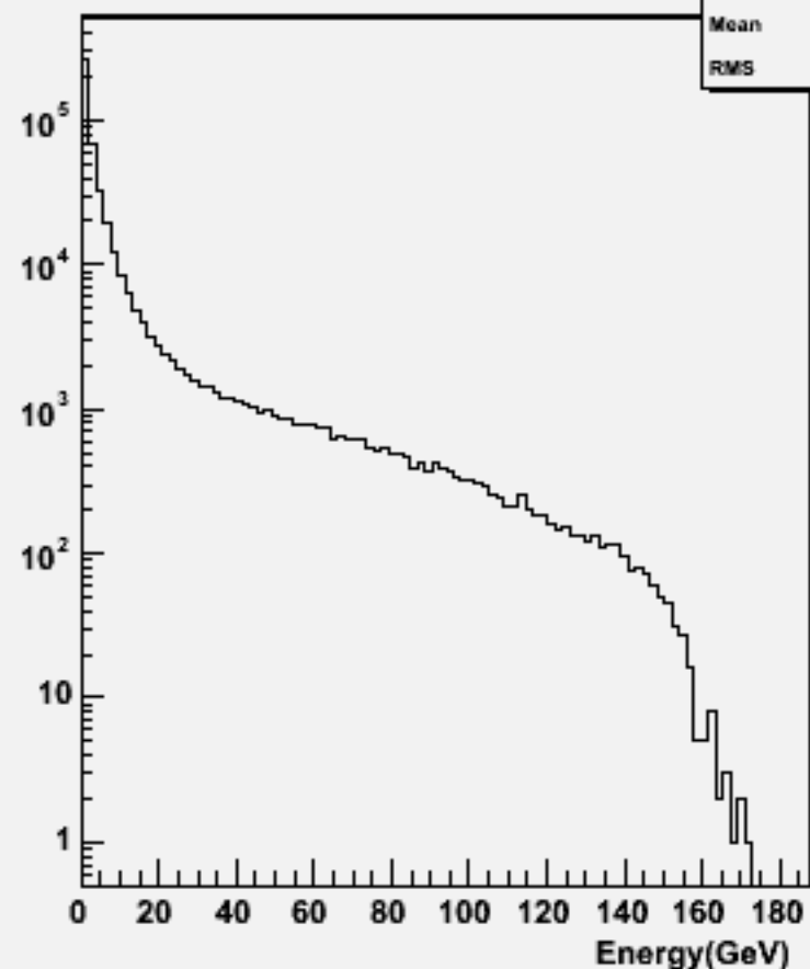
Start point R : w102165 n1n1e2e2dd_o
