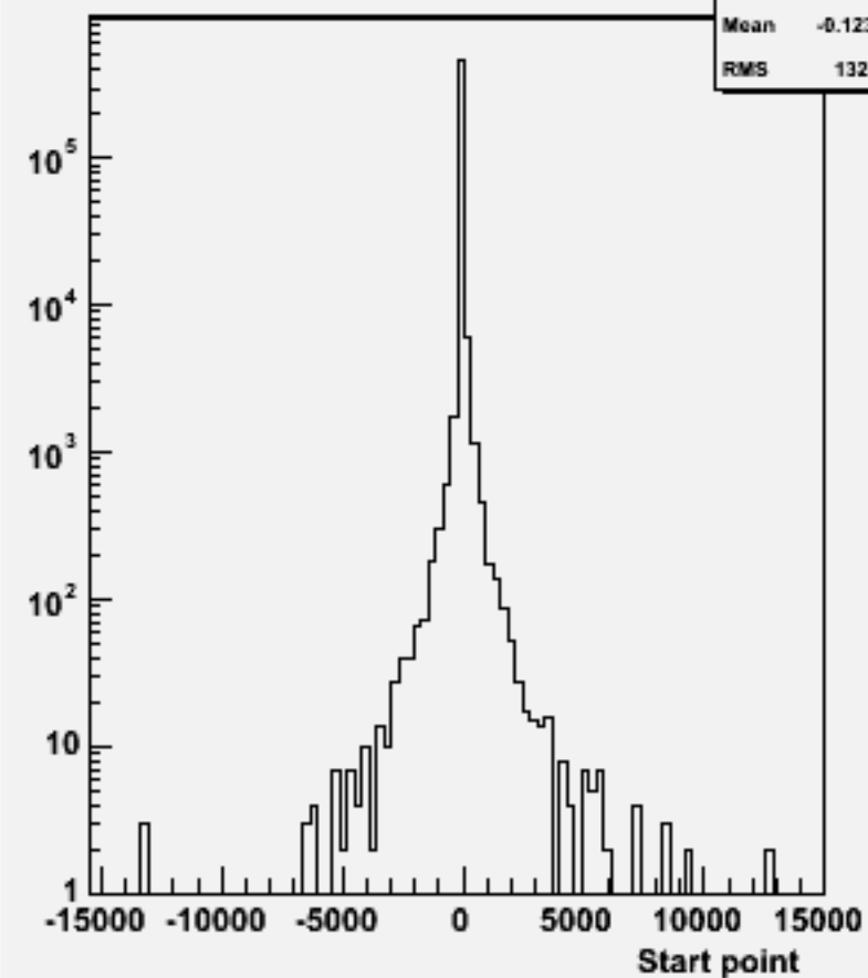
Start point Z : w102164 n1n1e2e2dd_o
