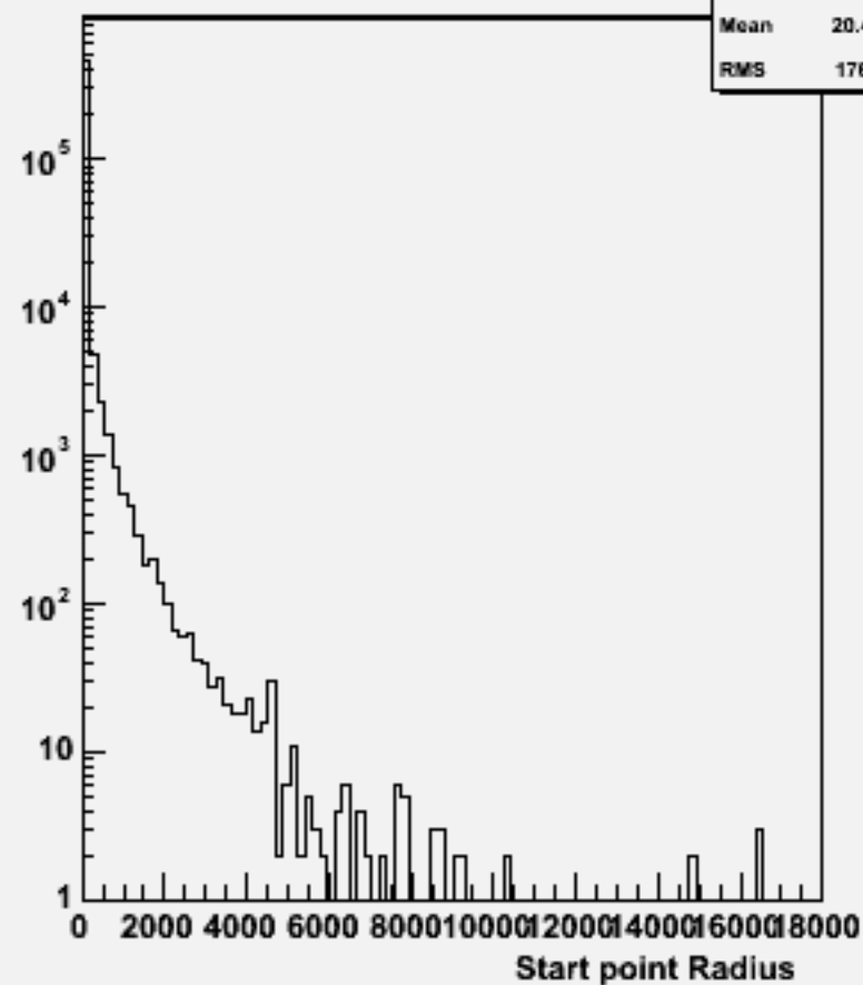
Start point R : w102164 n1n1e2e2dd_o
