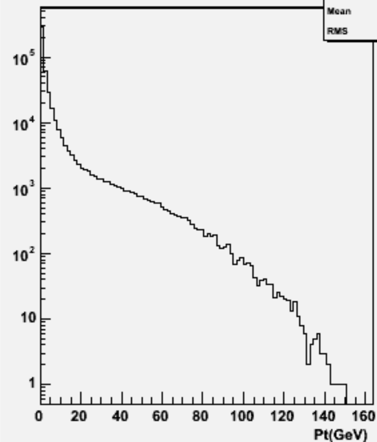
Start point Z : w102164 n1n1e2e2dd_o
