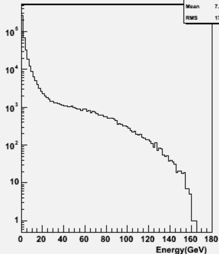
Start point R : w102164 n1n1e2e2dd_o
