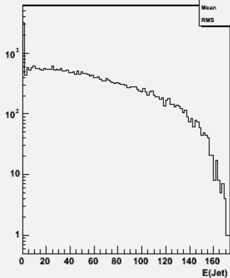
Jet energies(All jets)w102157 n1n1e2e2e2e2_o
