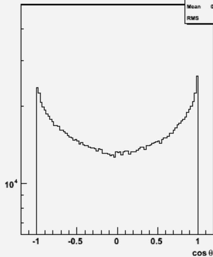
Particle cosθ : w102153 cccbb_o
