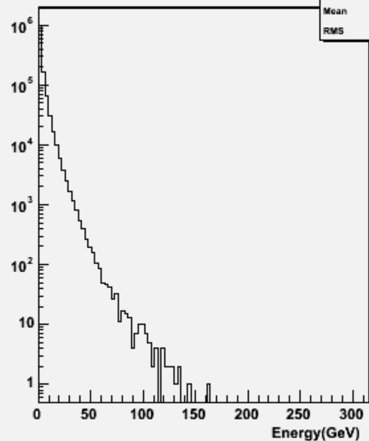
Start point R : w102153 cccbb_o
