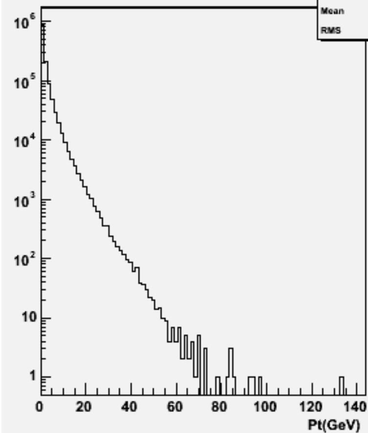
Start point Z : w102153 cccbb_o
