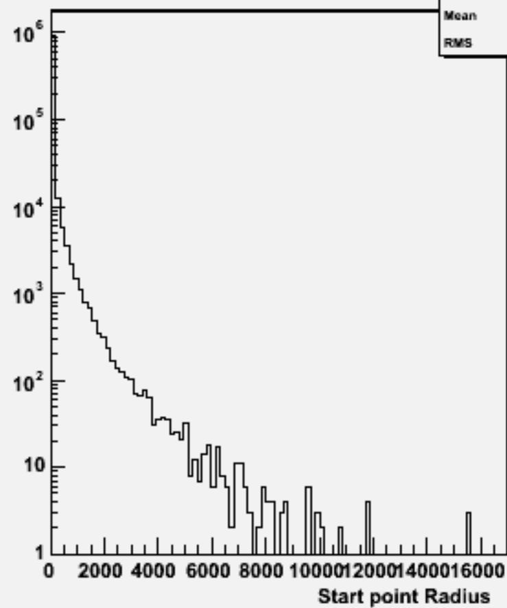
Start point R : w102144 cccce3e3_o
