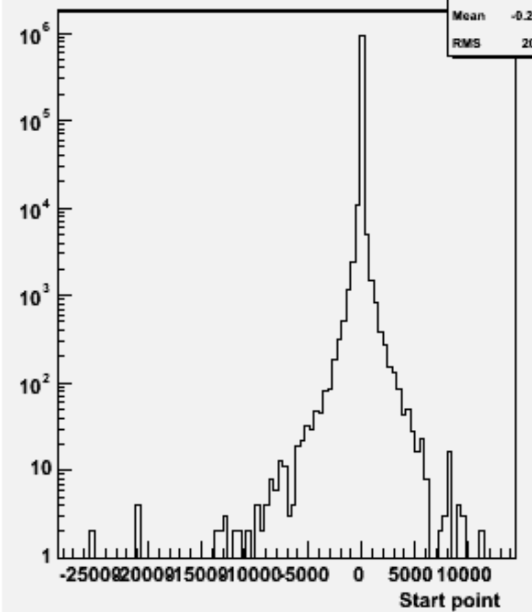
Start point Z : w102144 cccce3e3_o
