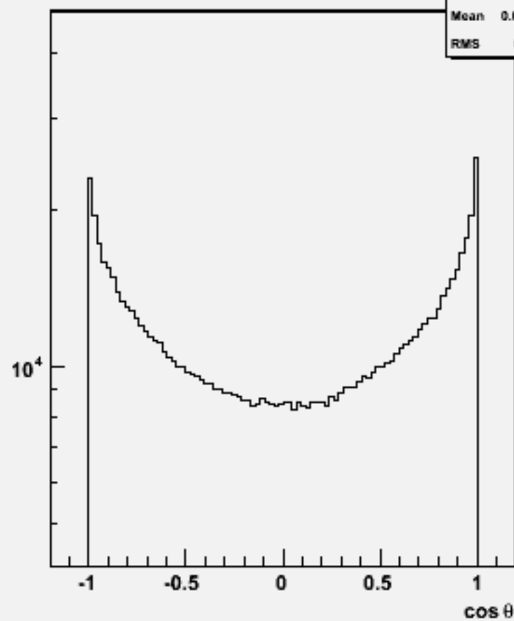
Particle cos \theta : w102144 cccce3e3_o
