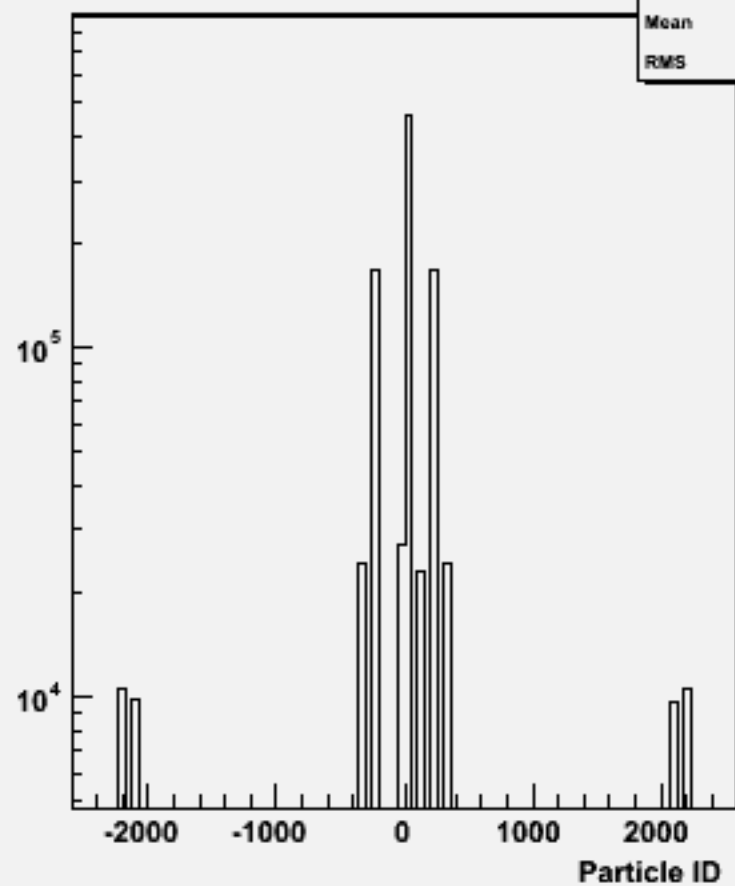
Particle ID : w102144 cccce3e3_o
