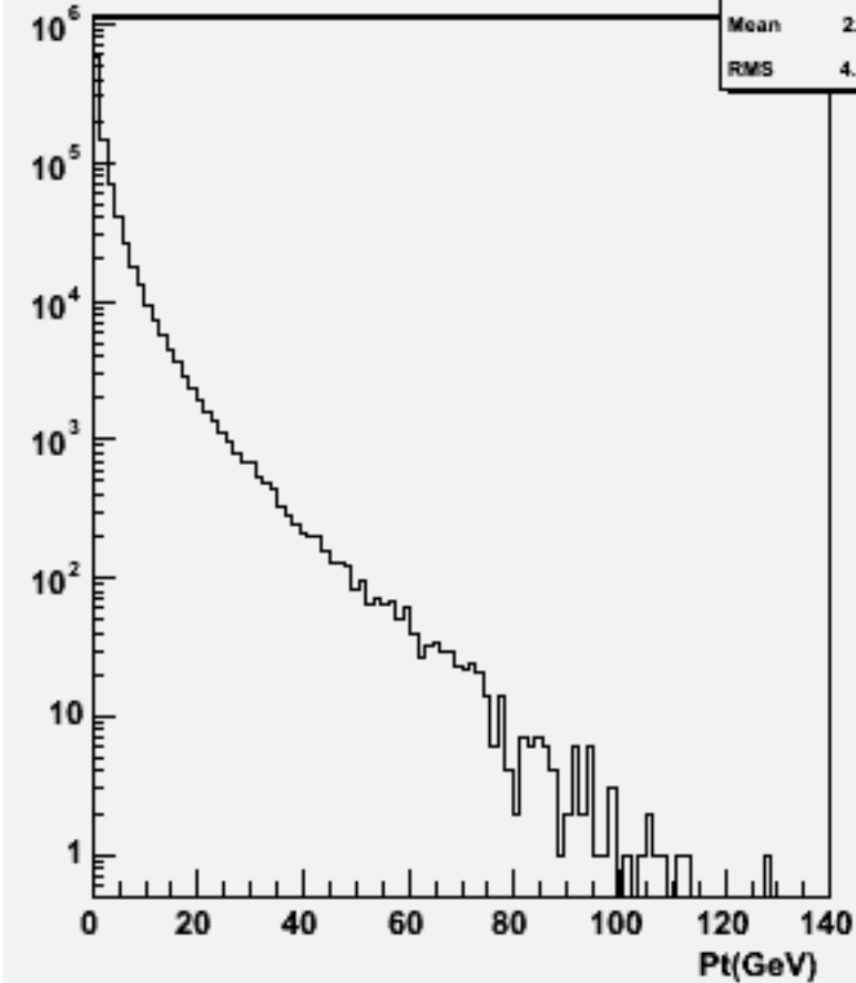
Particle Pt : w102144 cccce3e3_o
