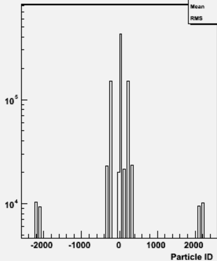
Particle ID : w102141 cccce2e2_o
