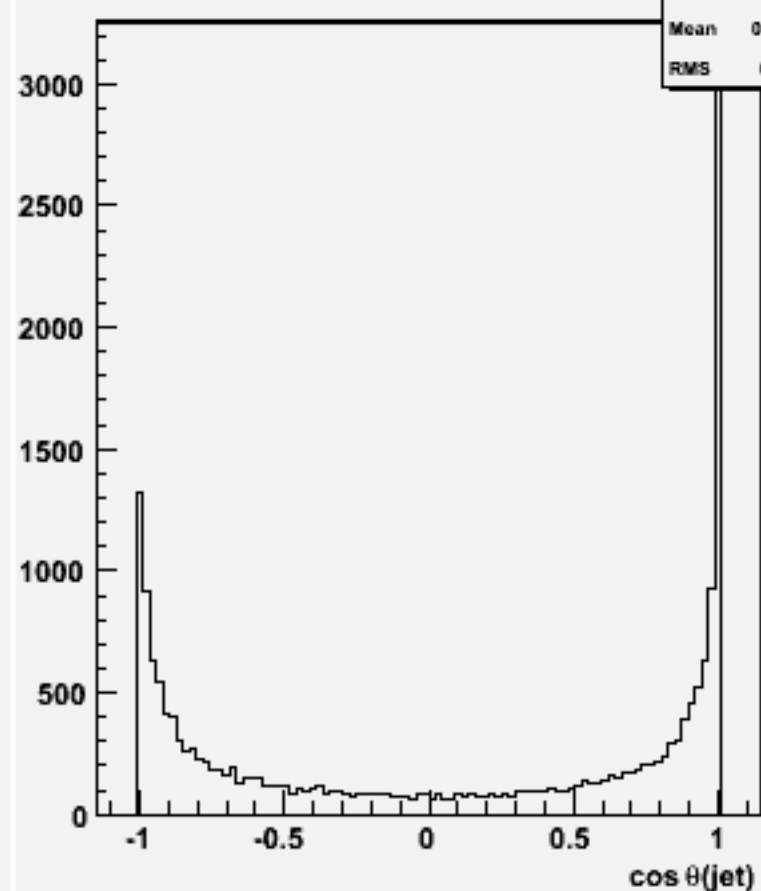
cos \theta for 2-jets :w102141 cccce2e2_o
