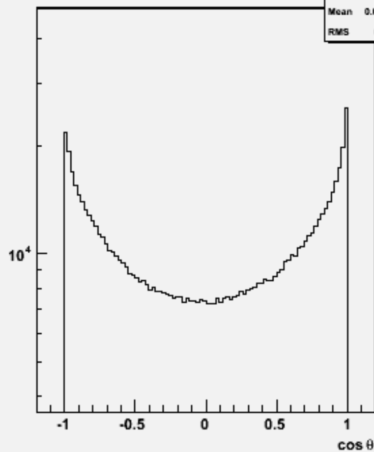
Particle cos \theta : w102141 cccce2e2_o
