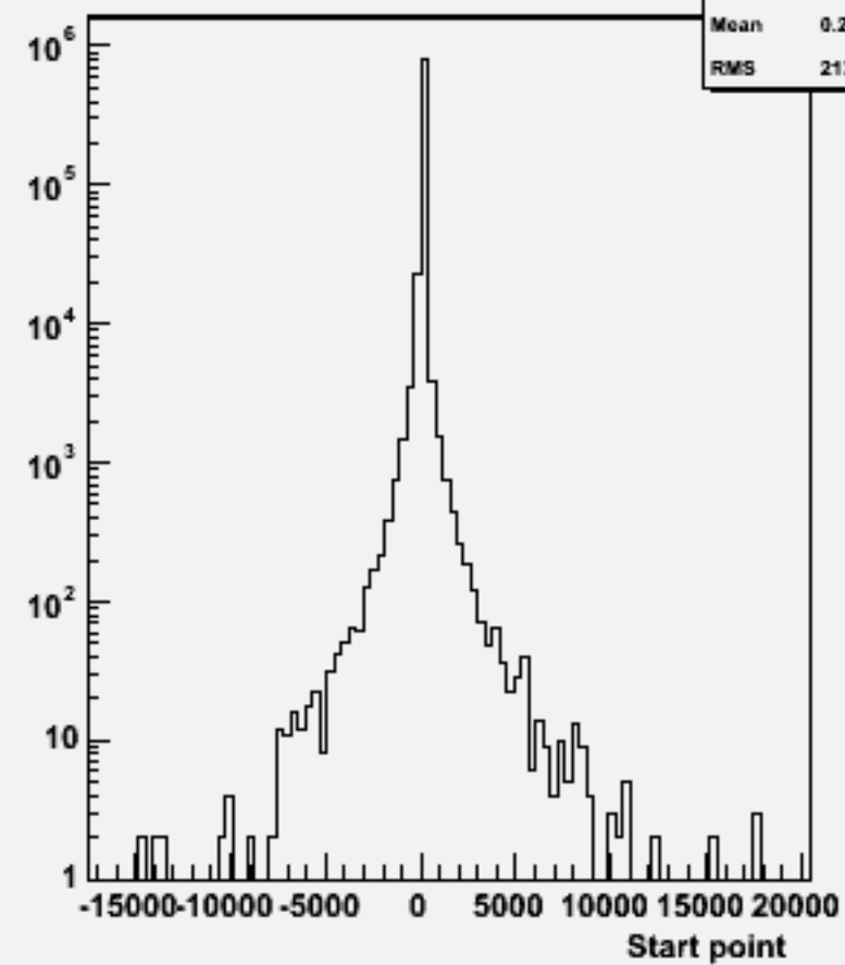
Start point Z : w102141 cccce2e2_o
