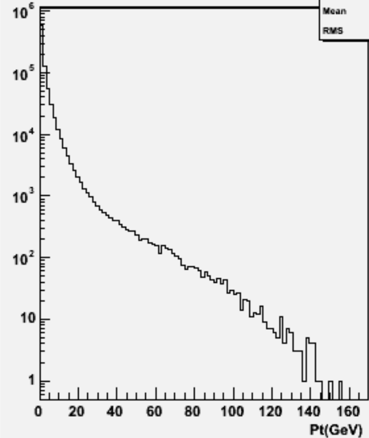
Particle Pt : w102141 cccce2e2_o
