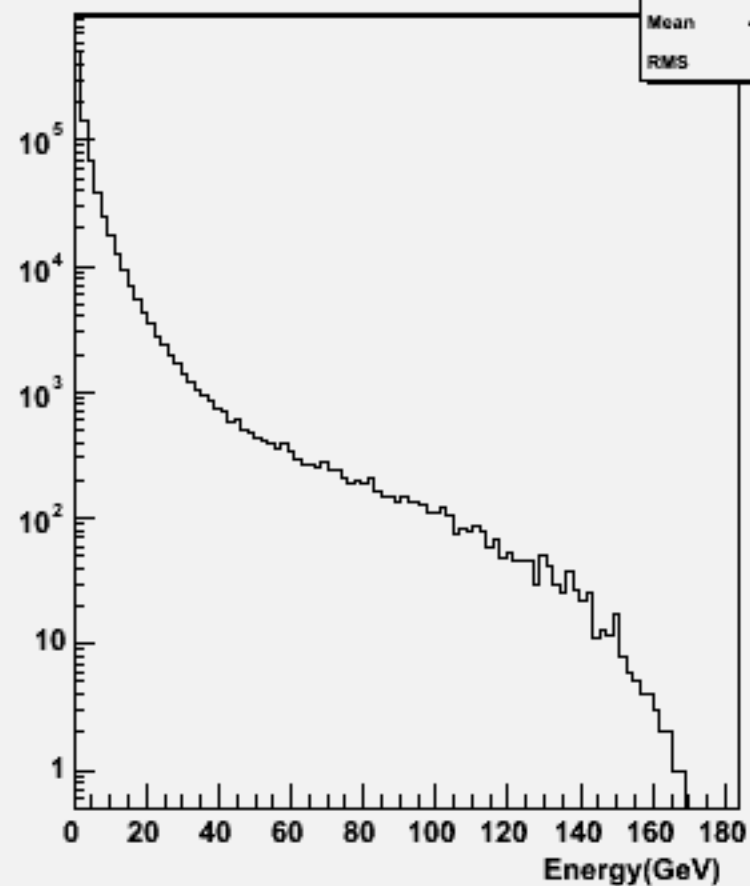
Particle Energy : w102141 cccce2e2_o
