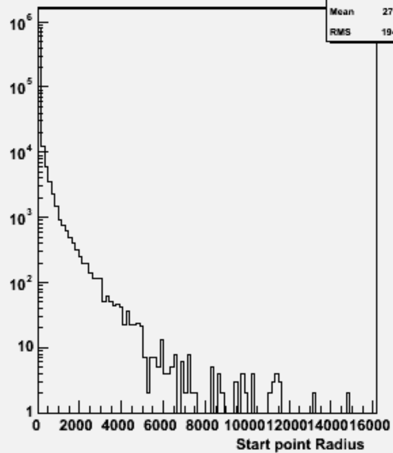
Start point R : w102141 cccce2e2_o
