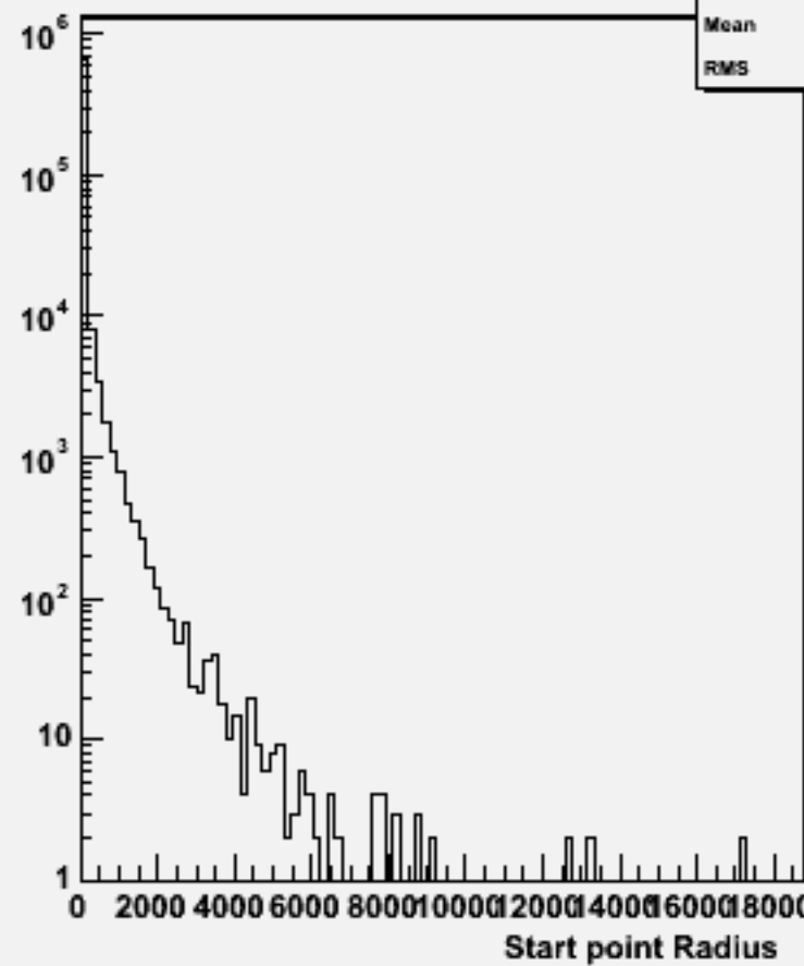
Start point R : w102138 cccce1e1_o
