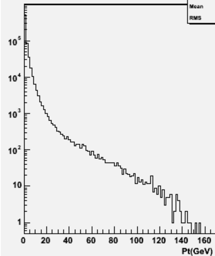
Particle Pt : w102138 cccce1e1_o
