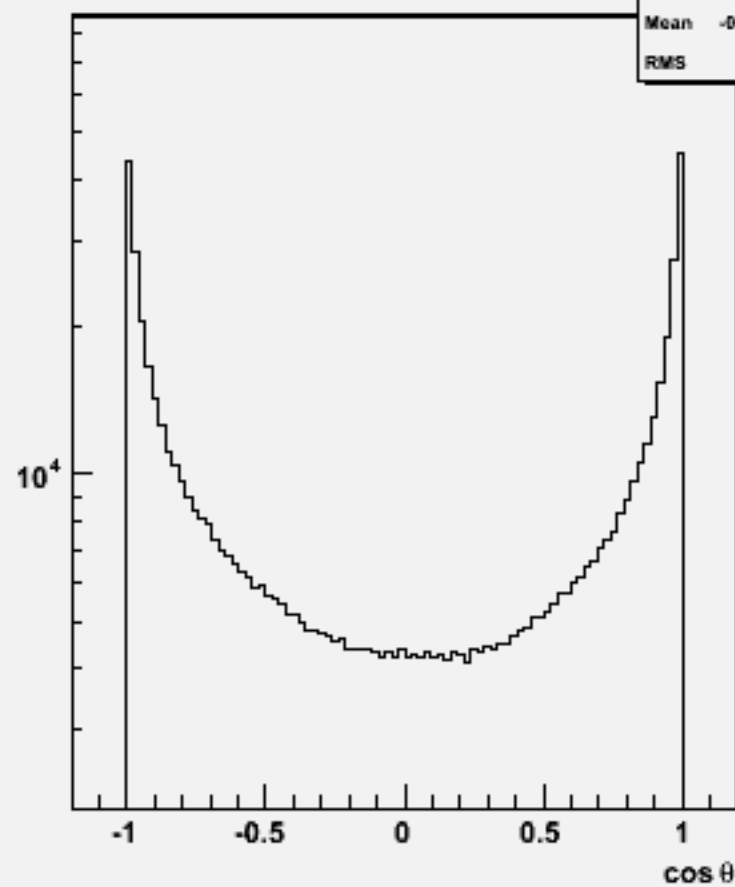
Particle cos \theta : w102138 cccce1e1_o
