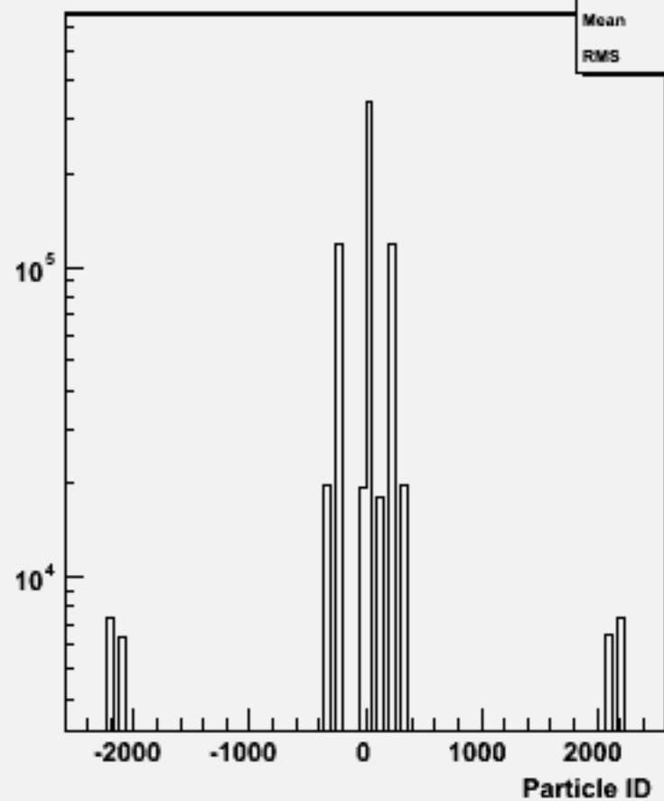
Particle ID : w102138 cccce1e1_o
