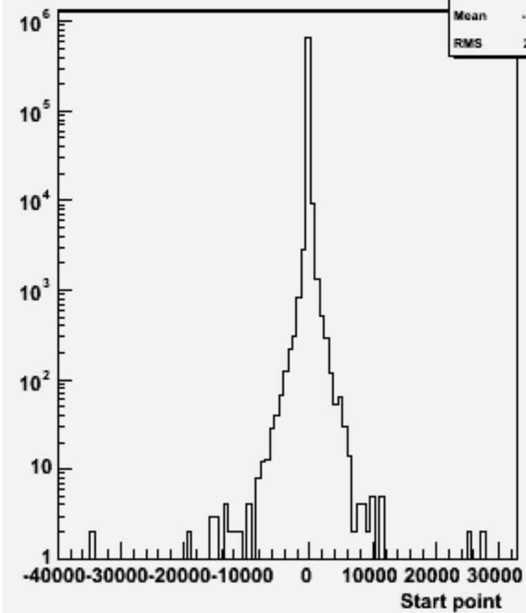
Start point Z : w102138 cccce1e1_o
