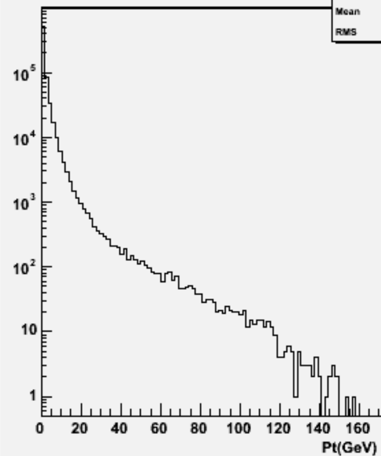
Particle Pt : w102135 cccce1e1_o
