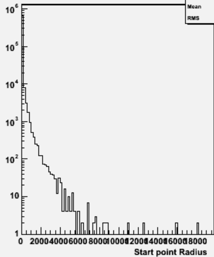
Start point R : w102135 cccce1e1_o
