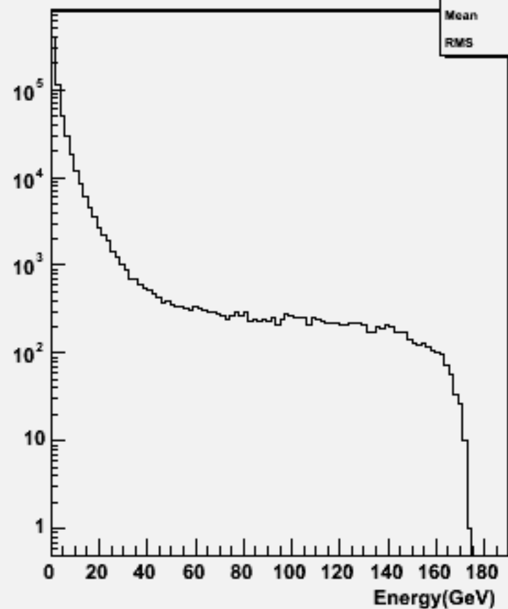
Particle Energy : w102135 cccce1e1_o
