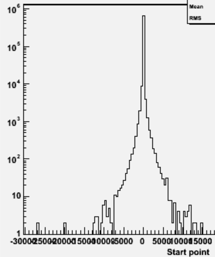
Start point Z : w102135 cccce1e1_o
