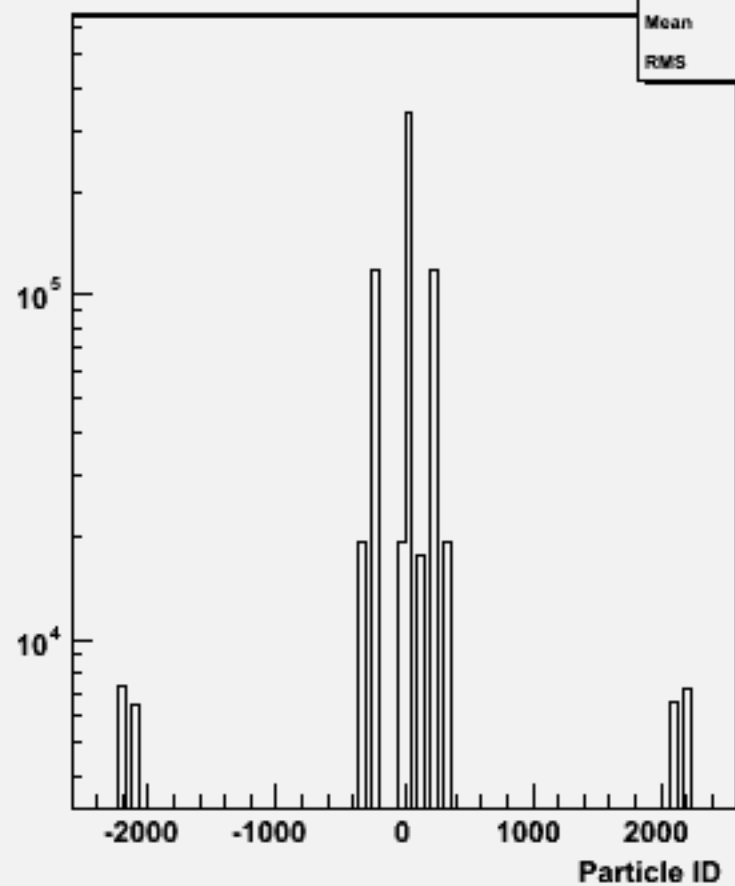
Particle ID : w102135 cccce1e1_o
