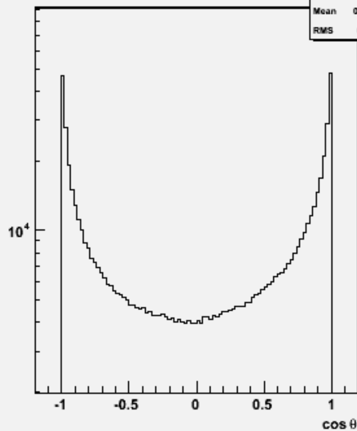
Particle cosθ : w102135 cccce1e1_o
