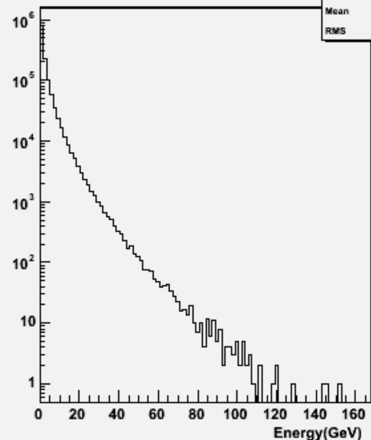
Start point R : w102132 uuccbb_o
