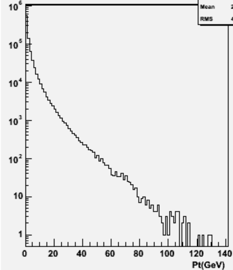
Particle Pt : w102129 uucce3e3_o
