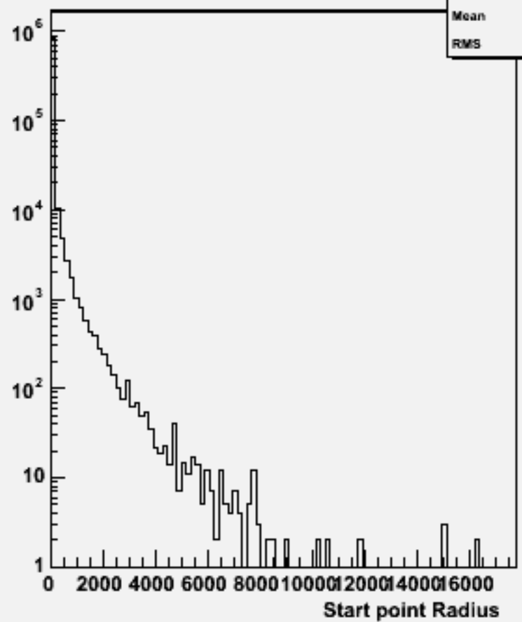
Start point R : w102129 uucce3e3_o
