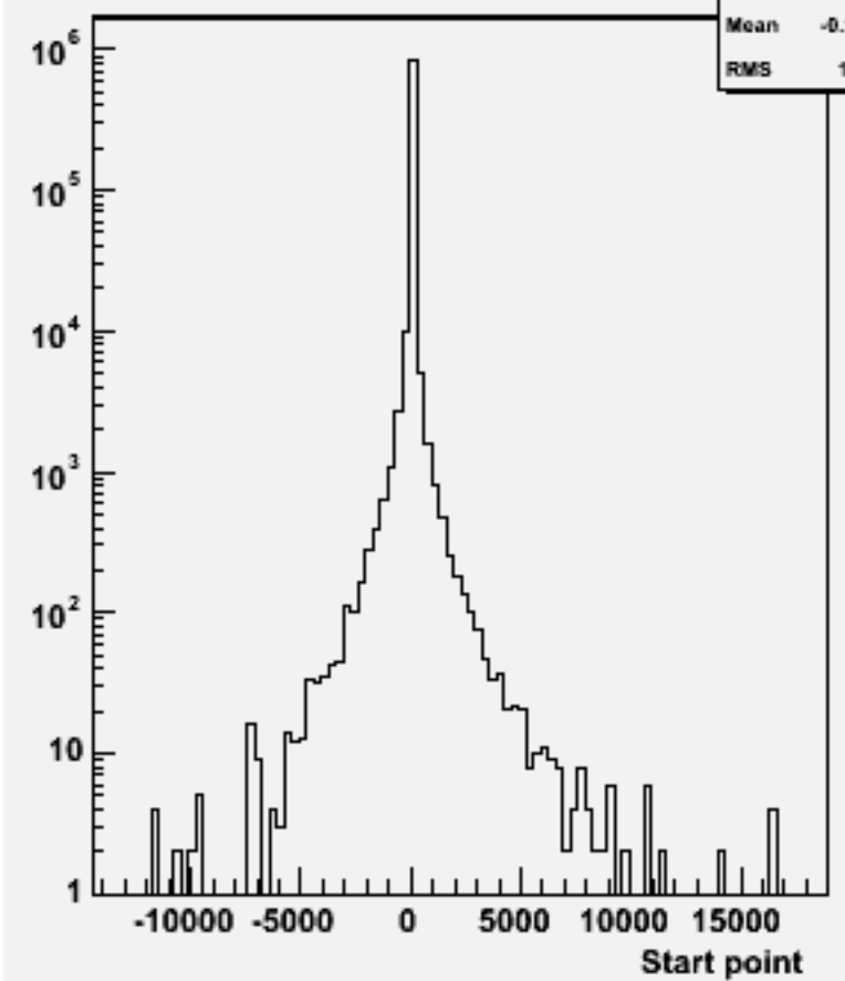
Start point Z : w102129 uucce3e3_o
