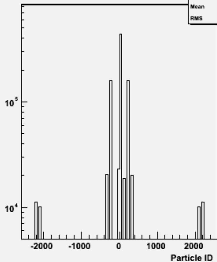
Particle ID : w102129 uucce3e3_o
