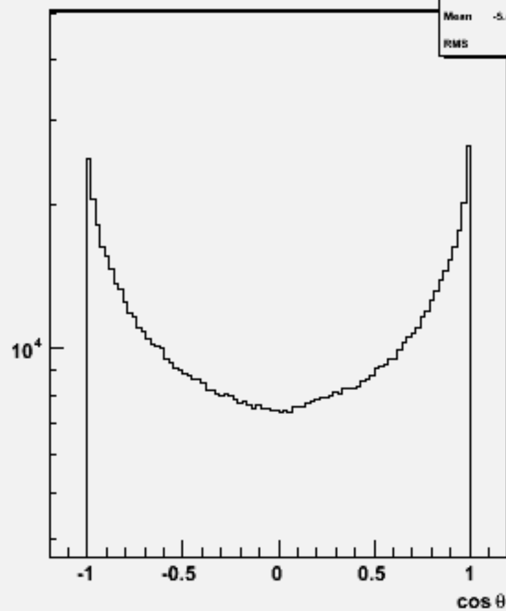
Particle cos \theta : w102129 uucce3e3_o
