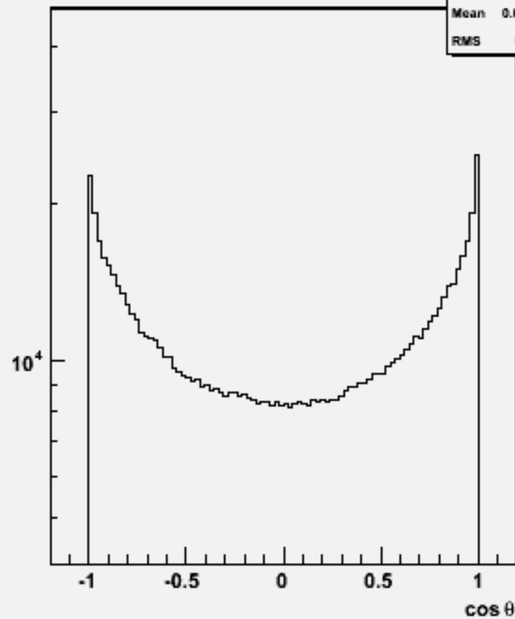
Particle cos \theta : w102128 uucce3e3_o
