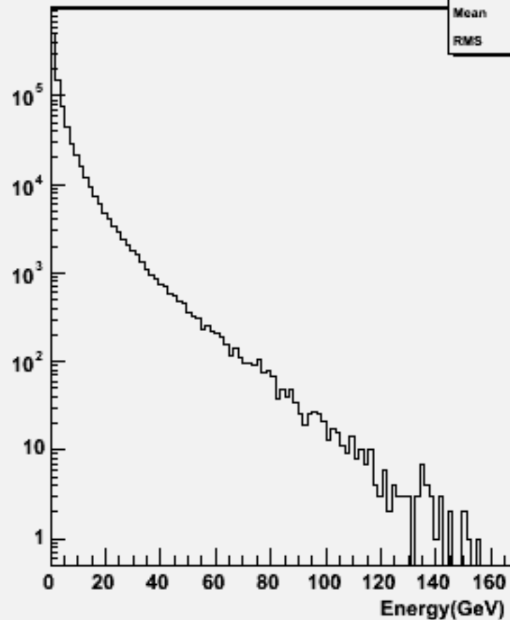
Start point R : w102128 uucce3e3_o
