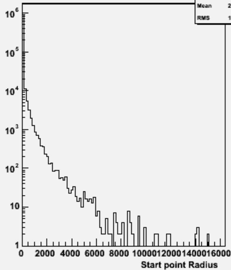
Start point R : w102128 uucce3e3_o
