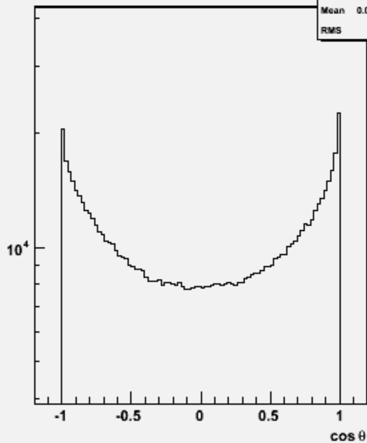
Particle cos \theta : w102124 uucce2e2_o
