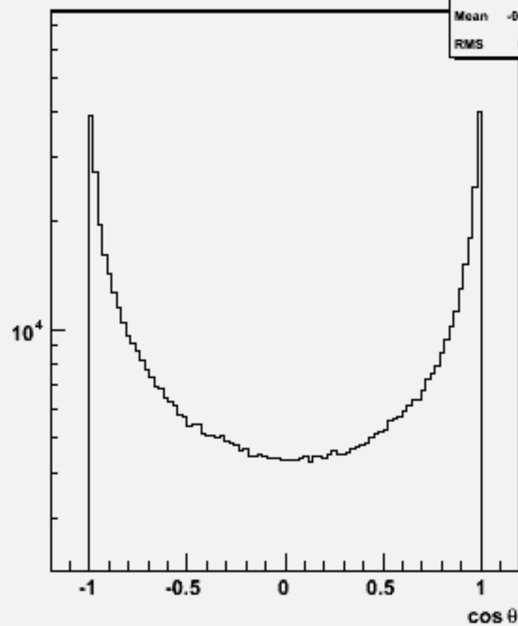
Particle cos \theta : w102122 uucce1e1_o
