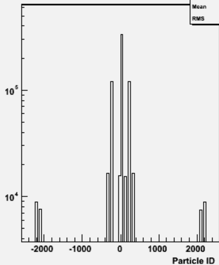
Particle ID : w102122 uucce1e1_o
