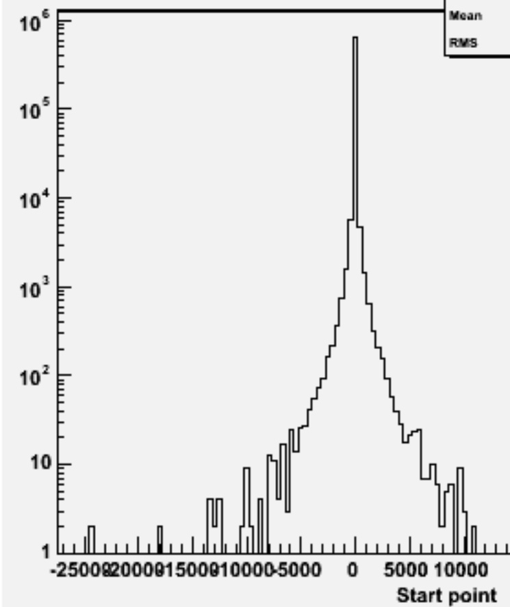
Start point Z : w102122 uucce1e1_o
