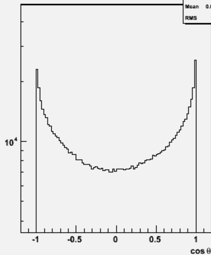
Particle cos \theta : w102120 uucce1e1_o
