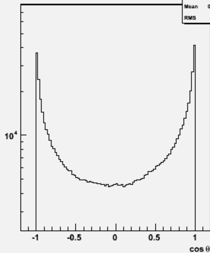
Particle cos \theta : w102119 uucce1e1_o
