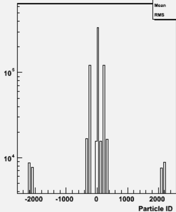
Particle ID : w102119 uucce1e1_o
