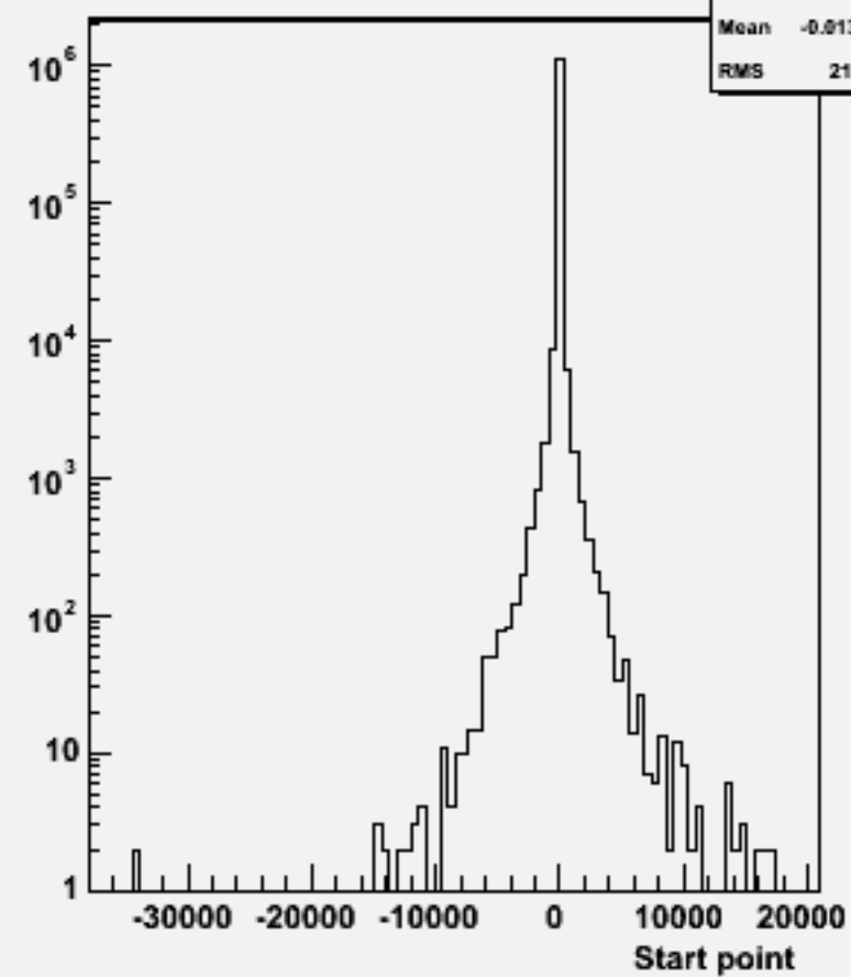
Start point Z : w102113 uuuuss_o
