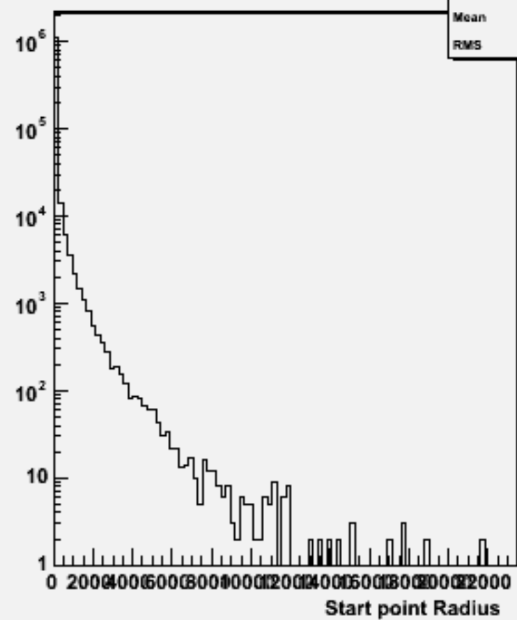
Start point R : w102113 uuuuss_o
