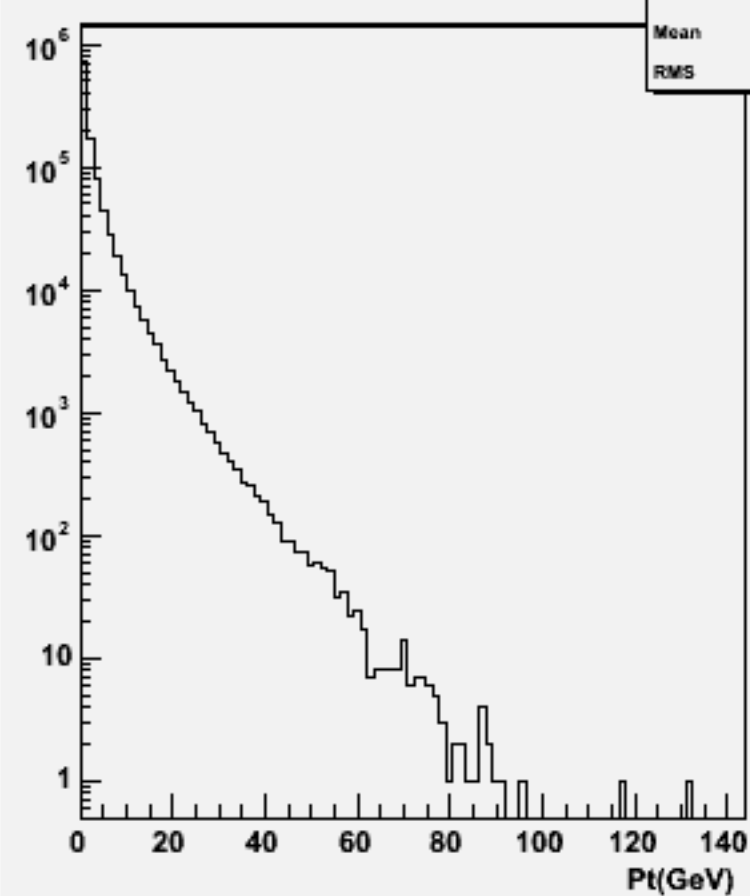
Particle Pt : w102113 uuuuss_o
