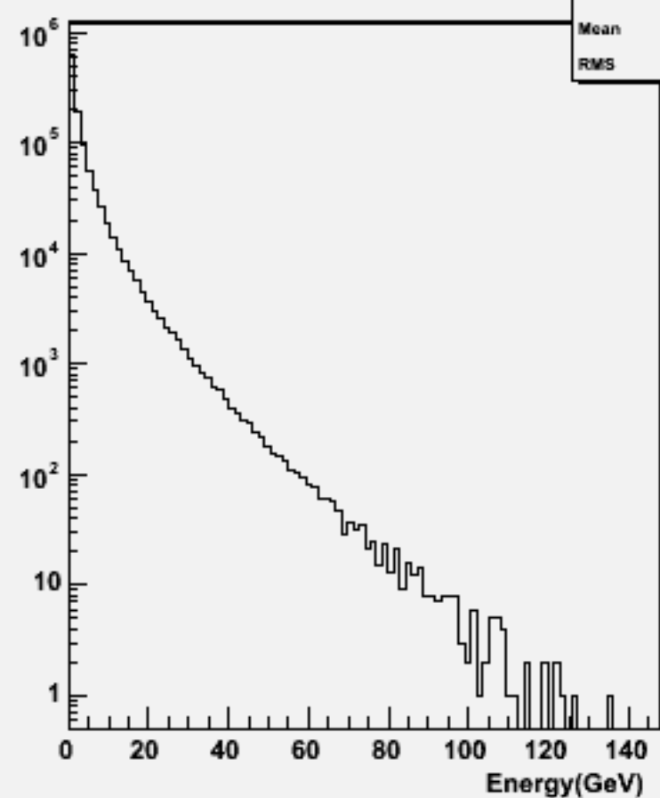
Particle Energy : w102113 uuuuss_o
