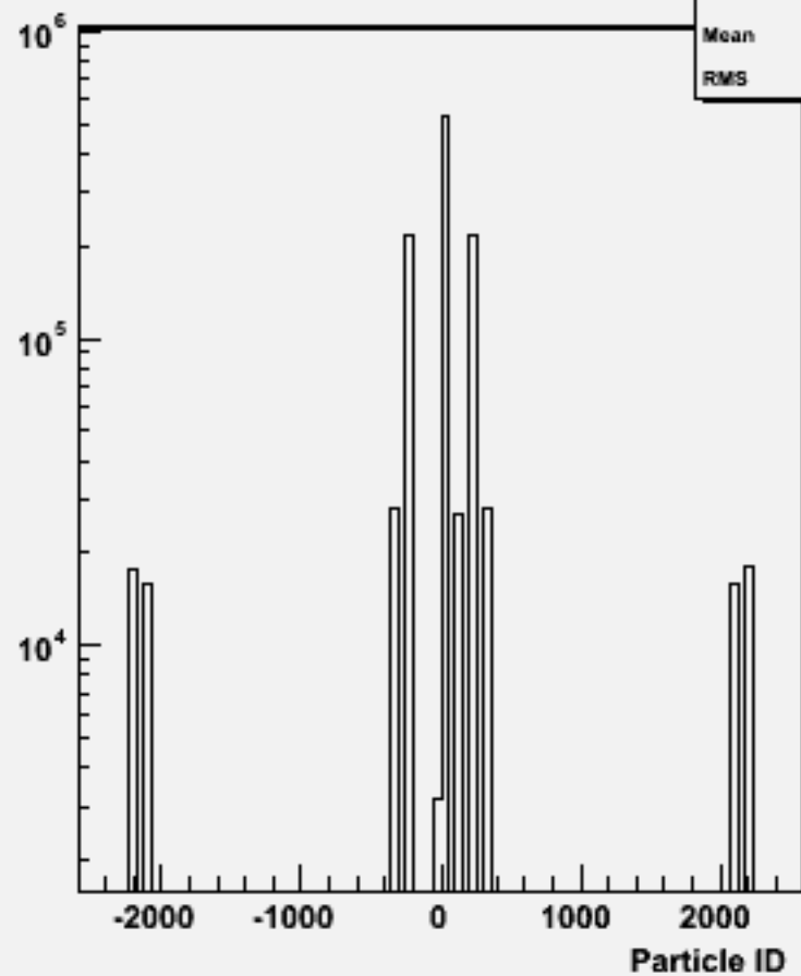
Particle ID : w102113 uuuuss_o
