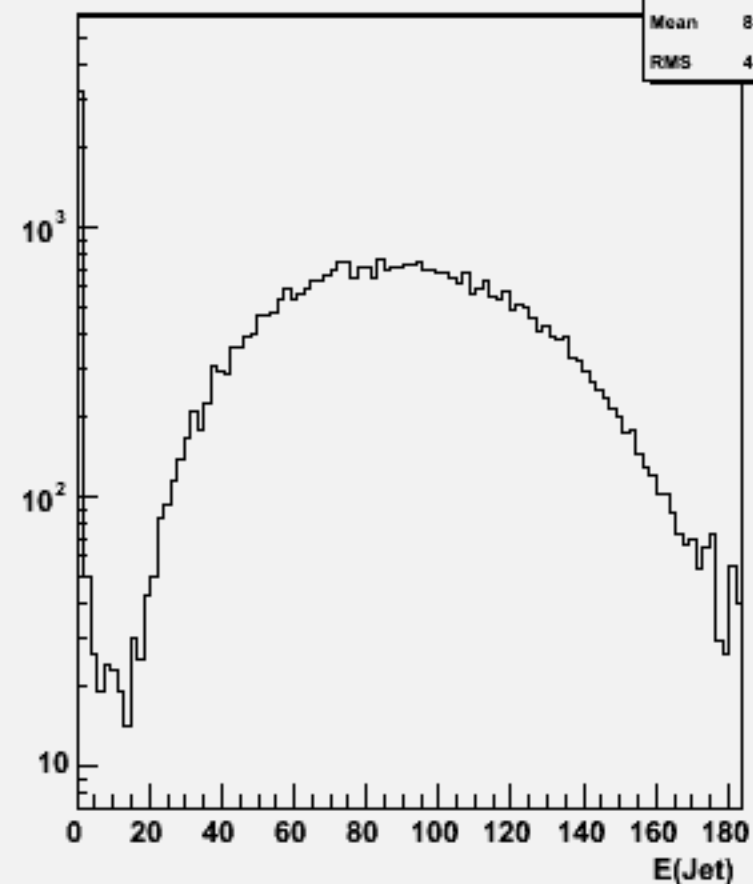
Jet energies(All jets)w102113 uuuuss_o
