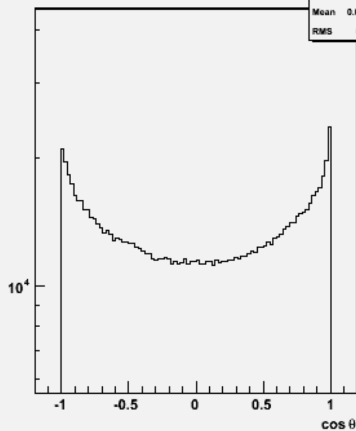
Particle cosθ : w102113 uuuuss_o
