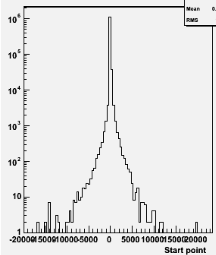
Start point Z : w102112 uuuuss_o
