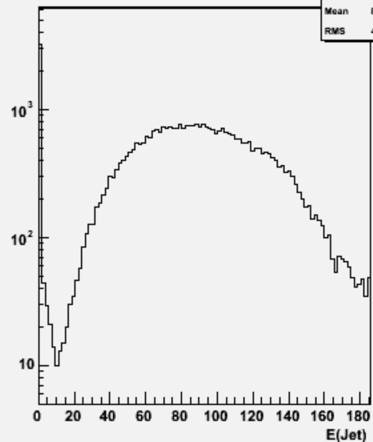
Jet energies(All jets)w102112 uuuuss_o
