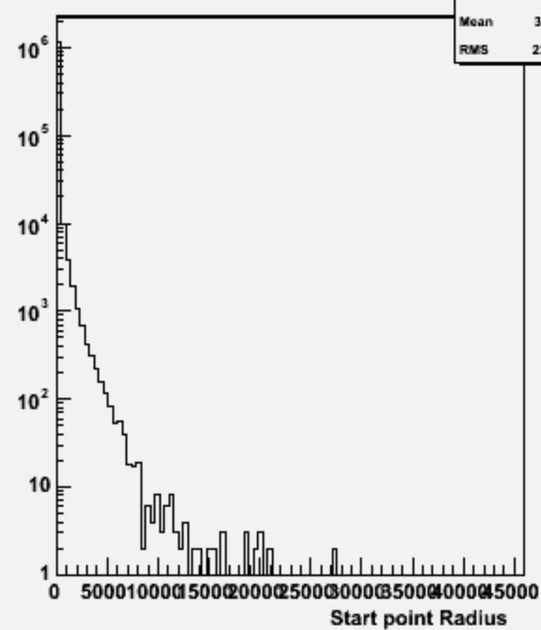
Start point R : w102112 uuuuss_o
