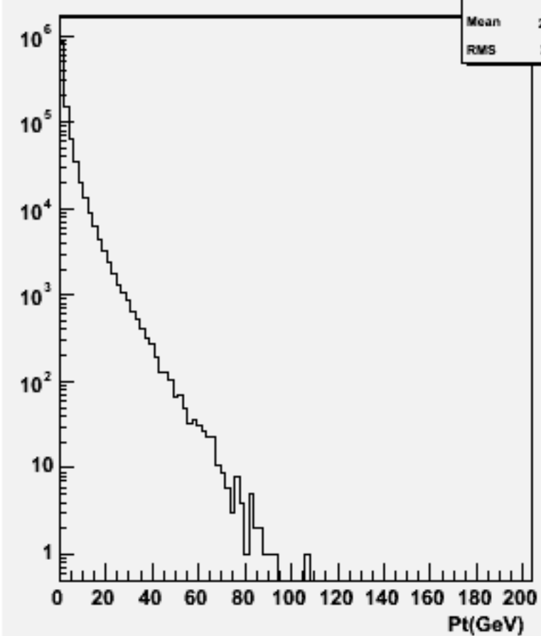
Particle Pt : w102112 uuuuss_o
