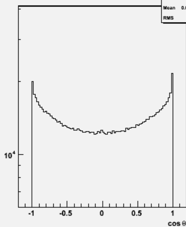
Particle cosθ : w102112 uuuuss_o
