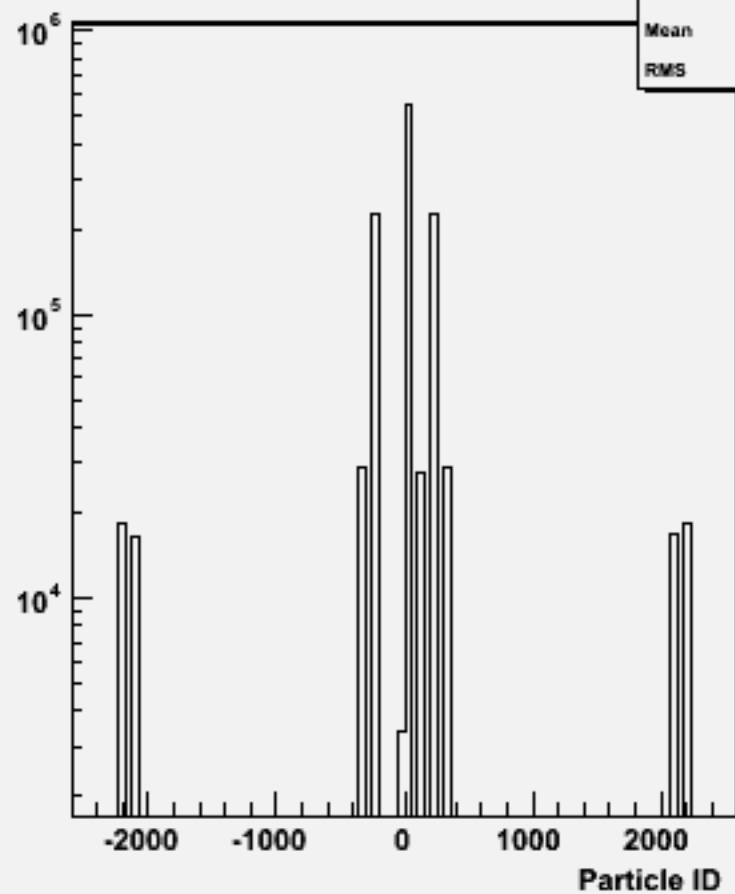
Particle ID : w102112 uuuuss_o
