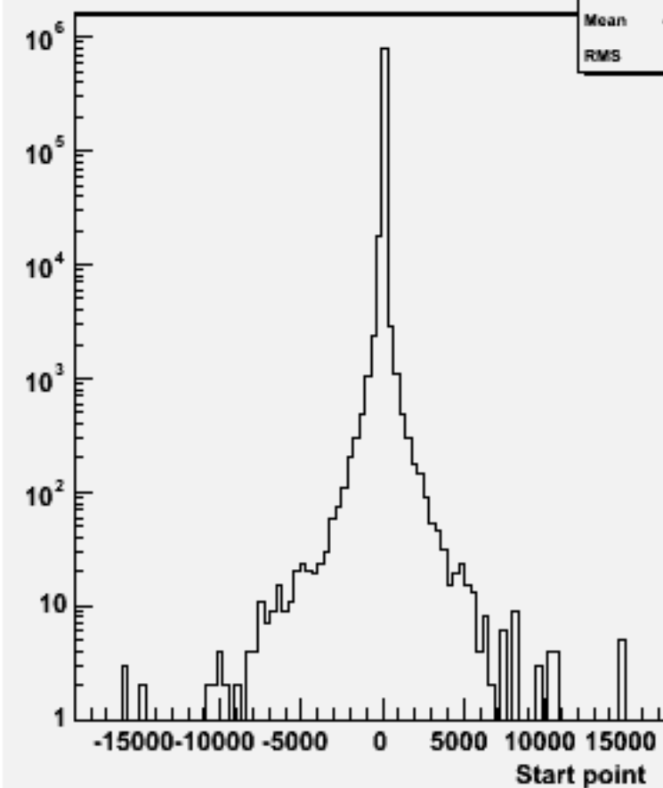
Start point Z : w102109 uuuue3e3_o
