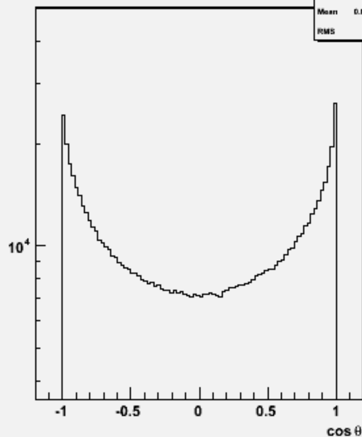
Particle cos \theta : w102109 uuuue3e3_o
