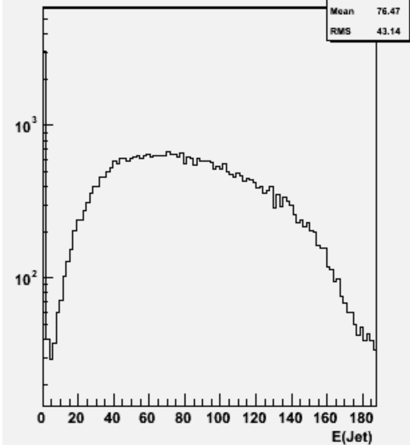
Jet energies(All jets)w102109 uuuue3e3_o
