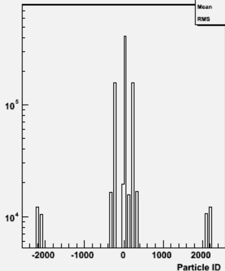
Particle ID : w102109 uuuue3e3_o
