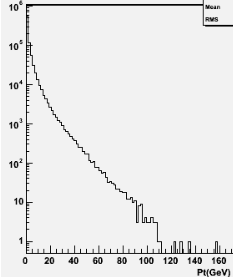
Particle Pt : w102109 uuuue3e3_o
