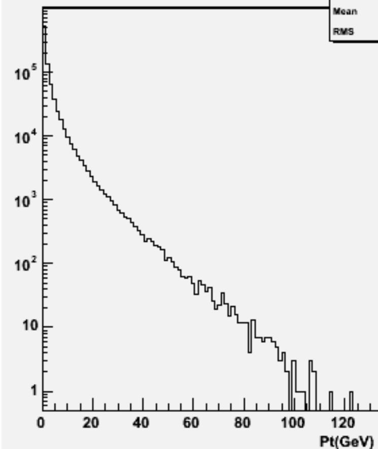
Particle Pt : w102108 uuuue3e3_o
