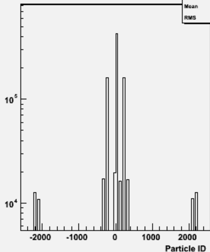
Particle ID : w102108 uuuue3e3_o
