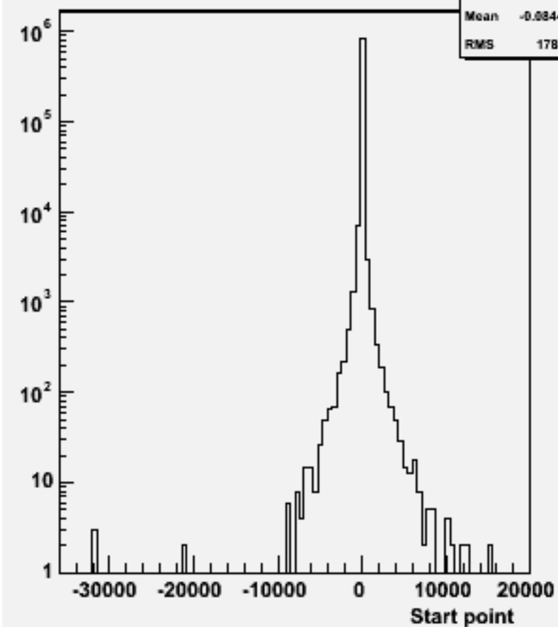
Start point Z : w102108 uuuue3e3_o
