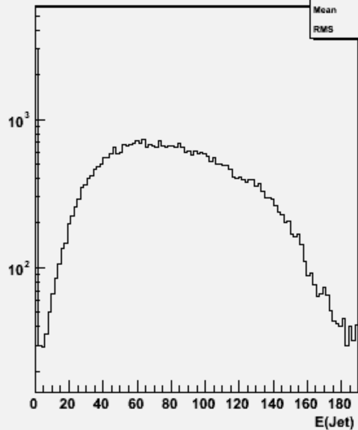
Jet energies(All jets)w102108 uuuue3e3_o
