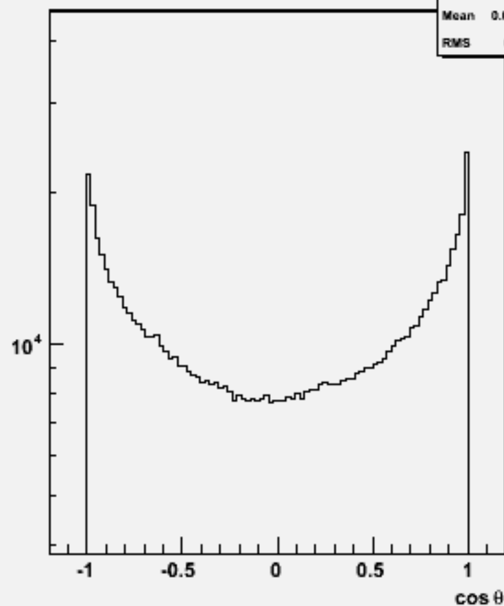
Particle cos \theta : w102108 uuuue3e3_o
