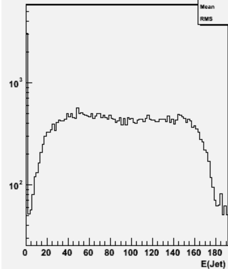
Jet energies(All jets)w102102 uuuue1e1_o
