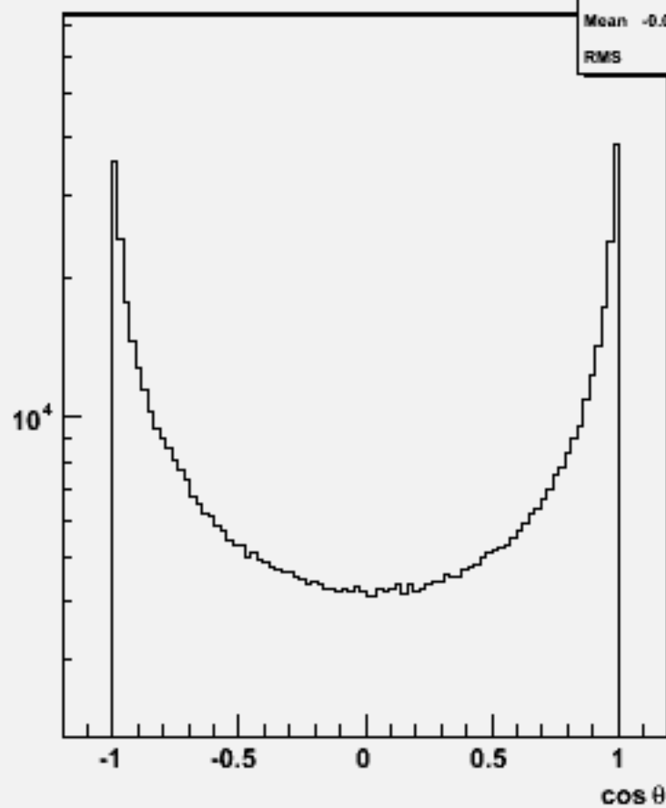
Particle cos \theta : w102102 uuuue1e1_o
