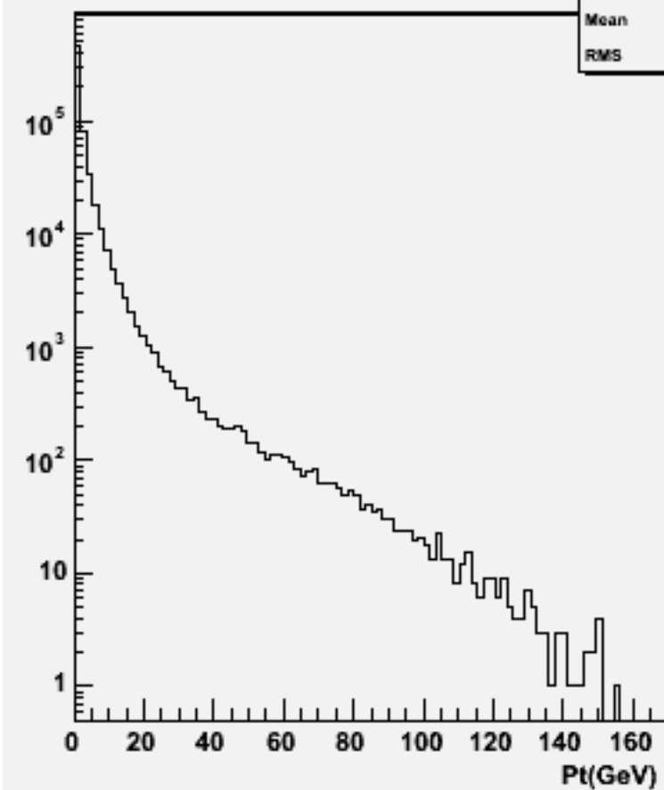
Particle Pt : w102102 uuuue1e1_o
