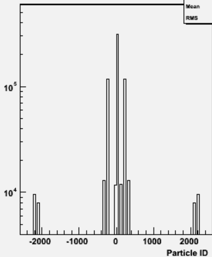
Particle ID : w102102 uuuue1e1_o
