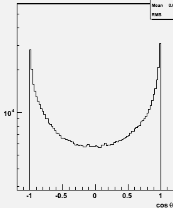
Particle cos \theta : w102101 uuuue1e1_o
