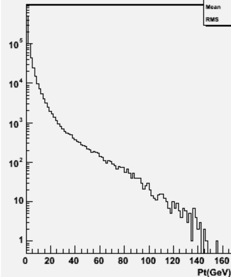
Particle Pt : w102101 uuuue1e1_o
