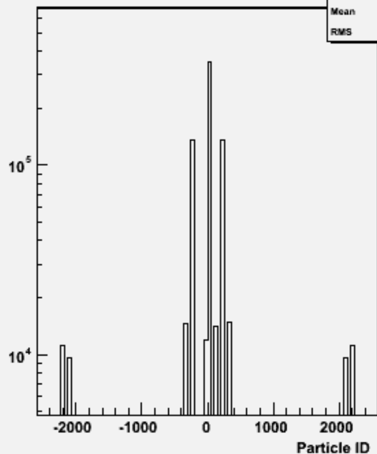
Particle ID : w102101 uuuue1e1_o
