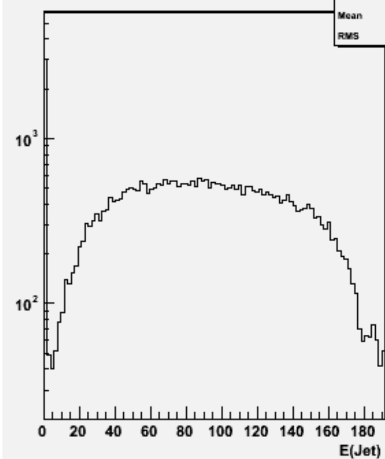
Jet energies(All jets)w102101 uuuue1e1_o
