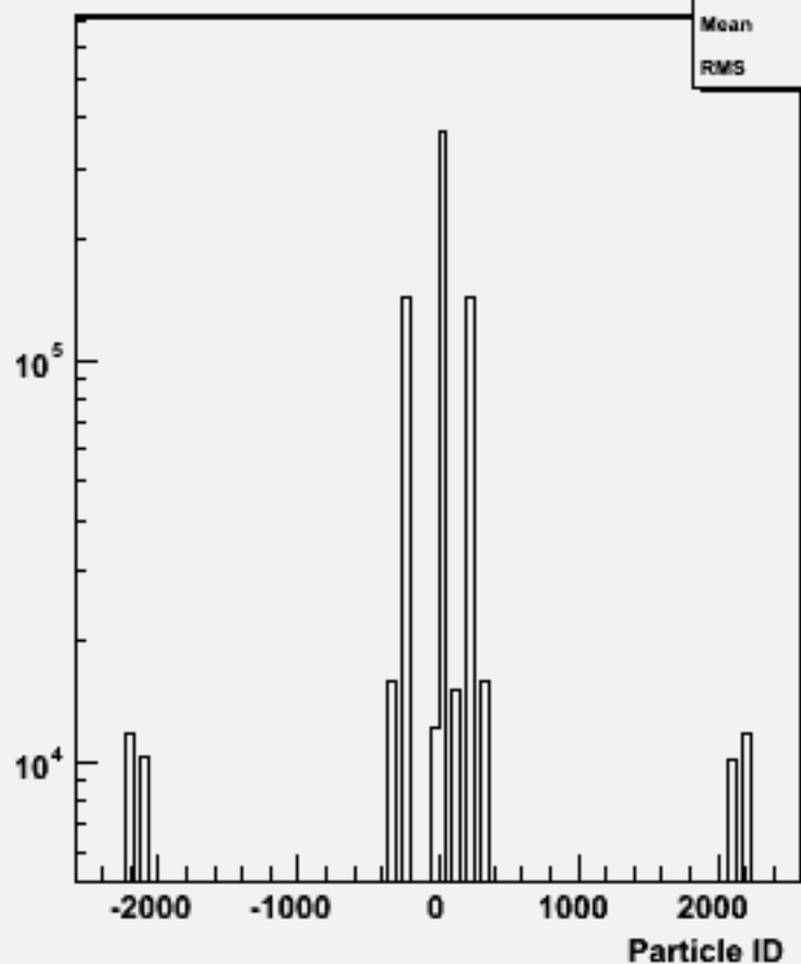
Particle ID : w102100 uuuue1e1_o
