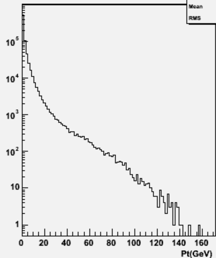
Particle Pt : w102100 uuuue1e1_o
