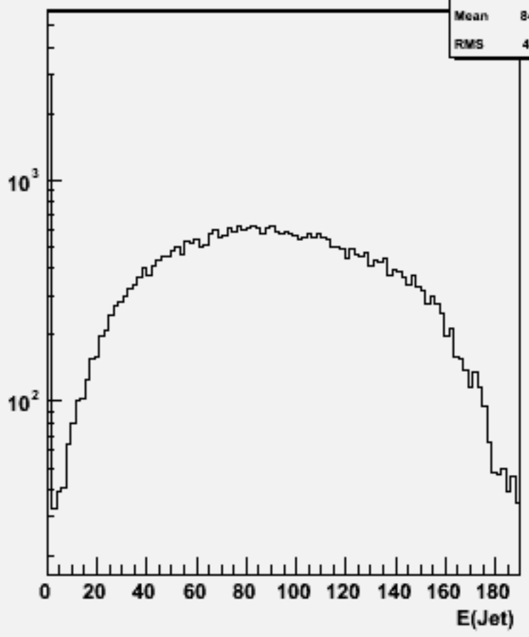
Jet energies(All jets)w102100 uuuue1e1_o
