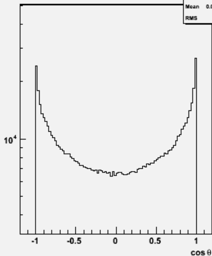
Particle cos \theta : w102100 uuuue1e1_o
