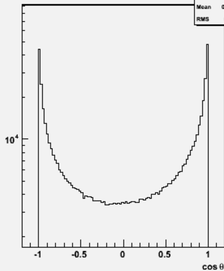
Particle cos \theta : w102099 uuuue1e1_o
