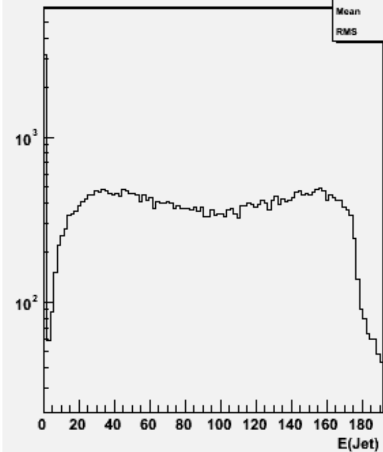
Jet energies(All jets)w102099 uuuue1e1_o
