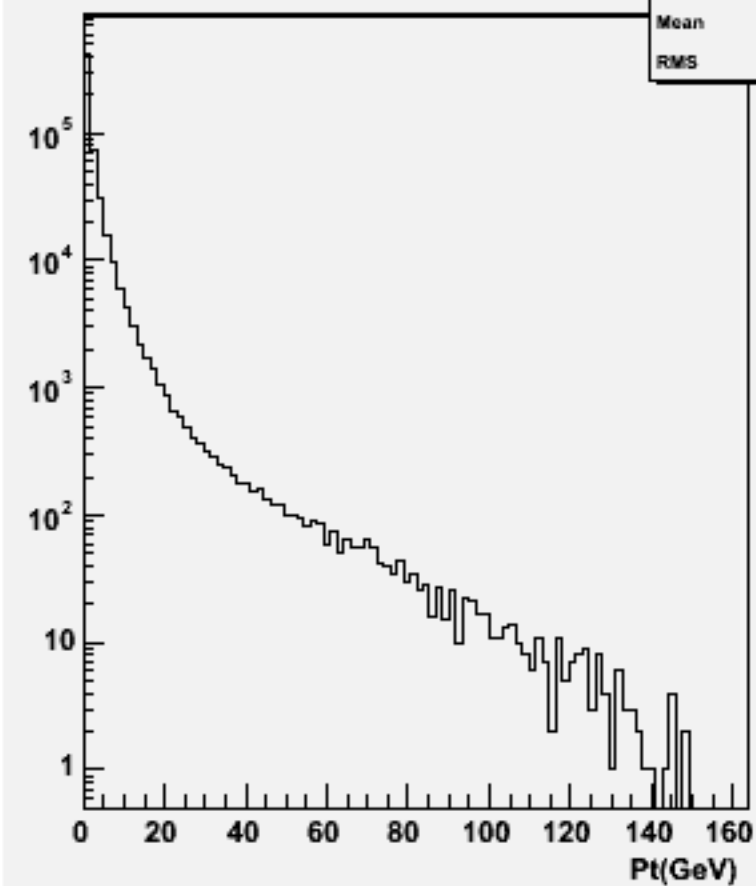
Particle Pt : w102099 uuuue1e1_o
