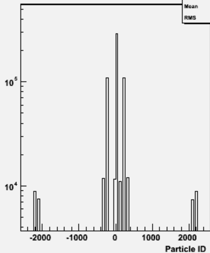
Particle ID : w102099 uuuue1e1_o
