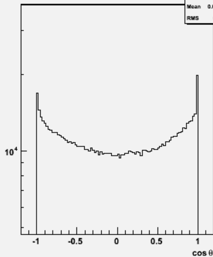
Particle cos \theta : w102097 n3n3ccbb_o
