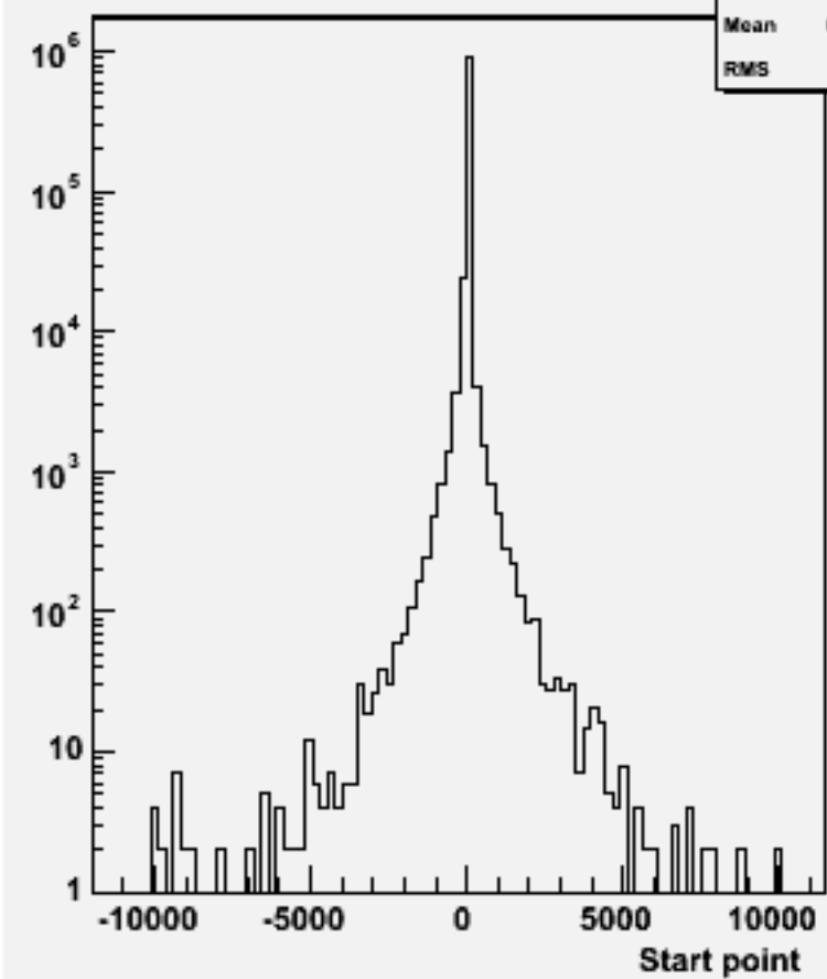
Start point Z : w102097 n3n3ccbb_o
