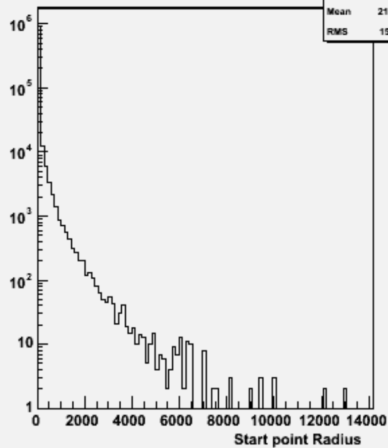
Start point R : w102097 n3n3ccbb_o
