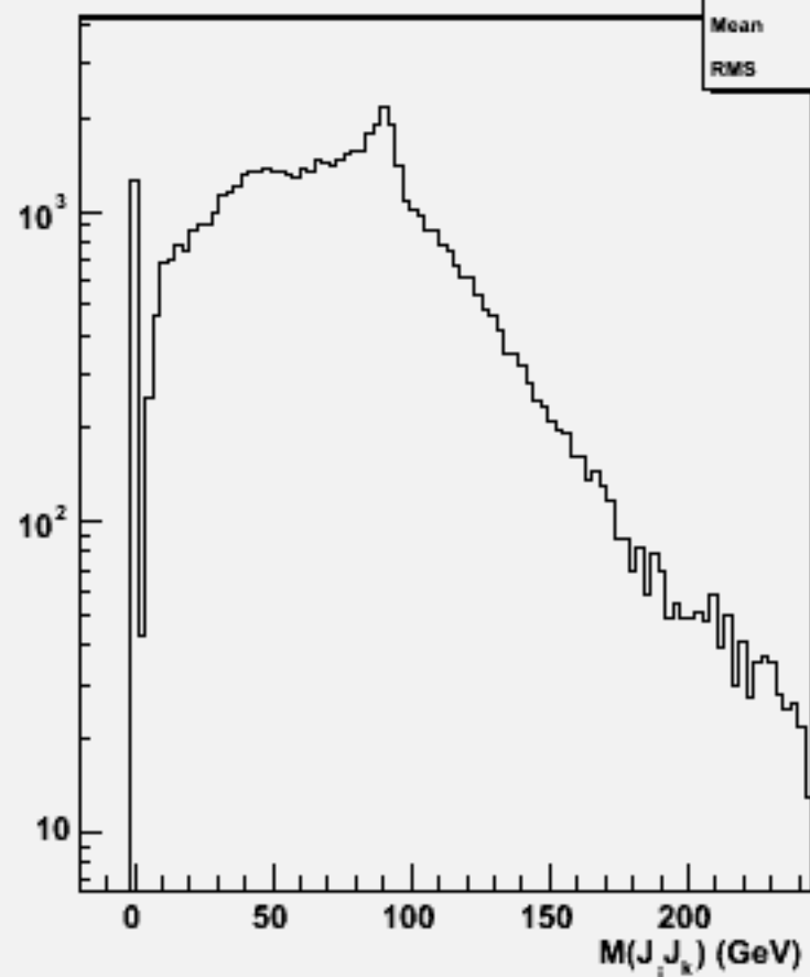
2jets mass(All comb)w102097 n3n3ccbb_o
