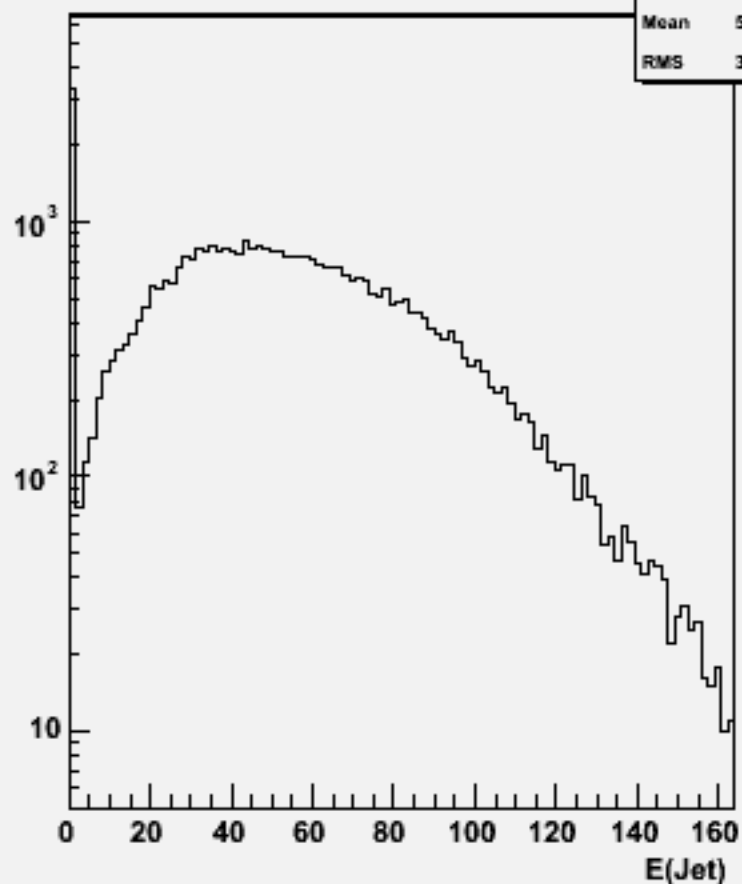
Jet energies(All jets)w102097 n3n3ccbb_o
