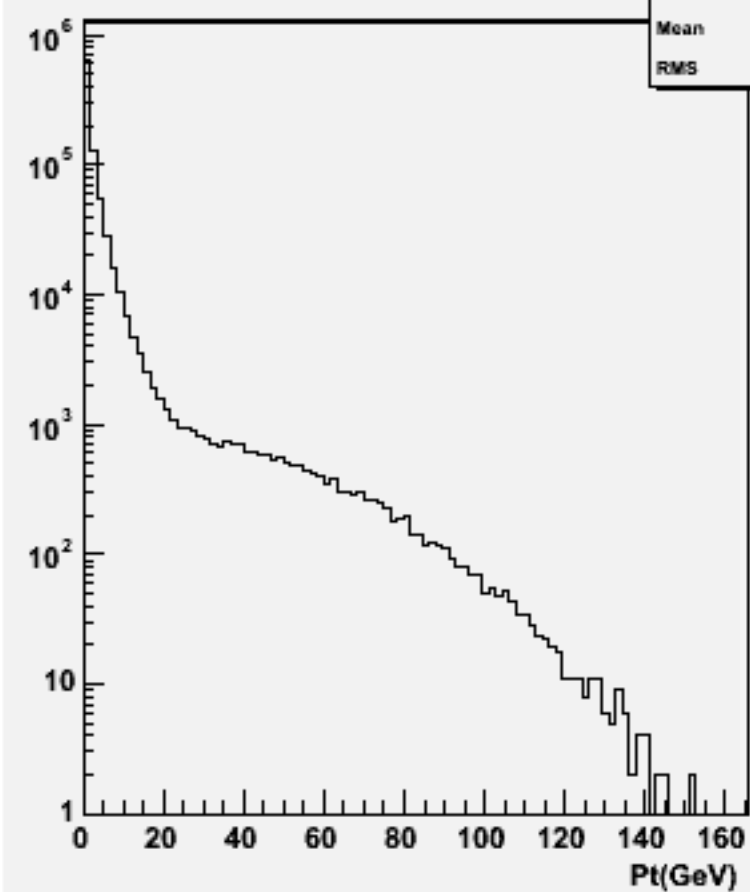
Particle Pt : w102097 n3n3ccbb_o
