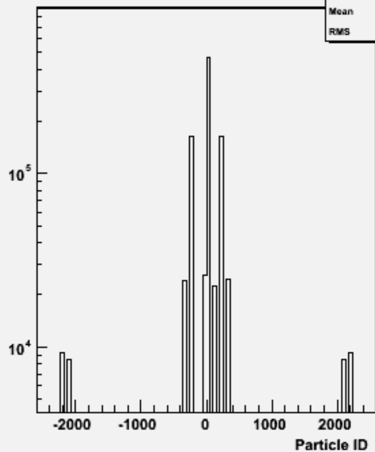
Particle ID : w102097 n3n3ccbb_o
