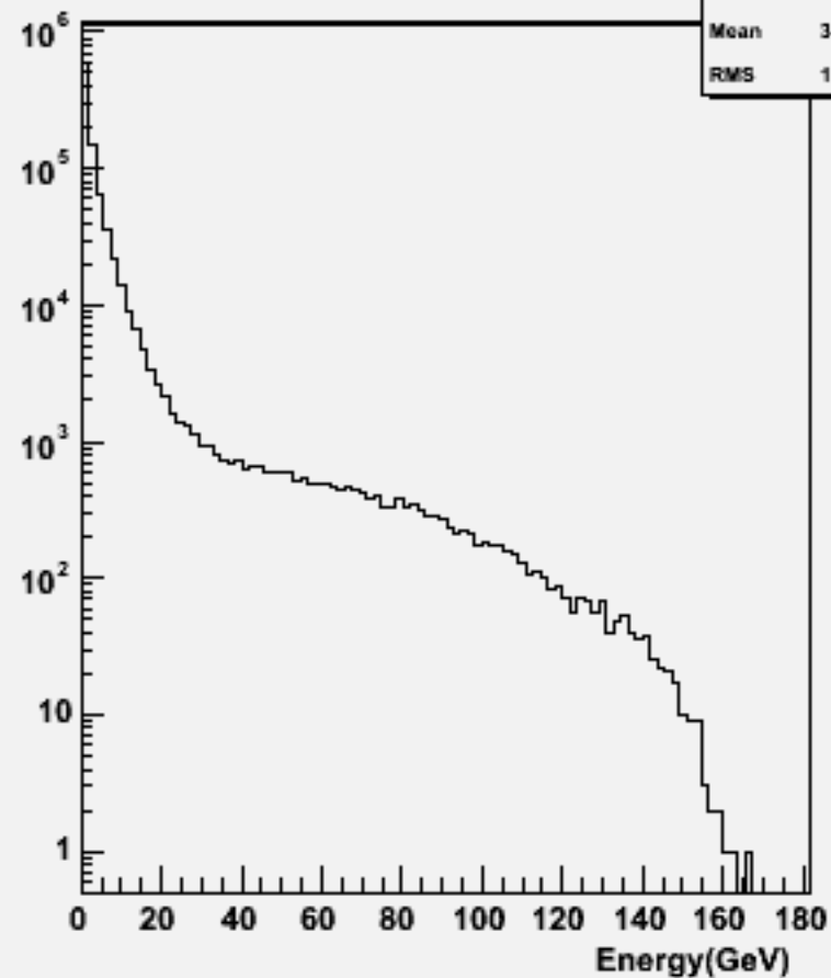
Particle Energy : w102097 n3n3ccbb_o
