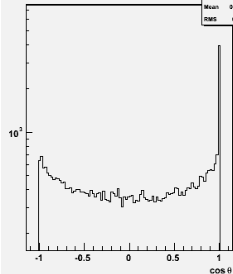
Jet cos \theta (All jets)w102097 n3n3ccbb_o
