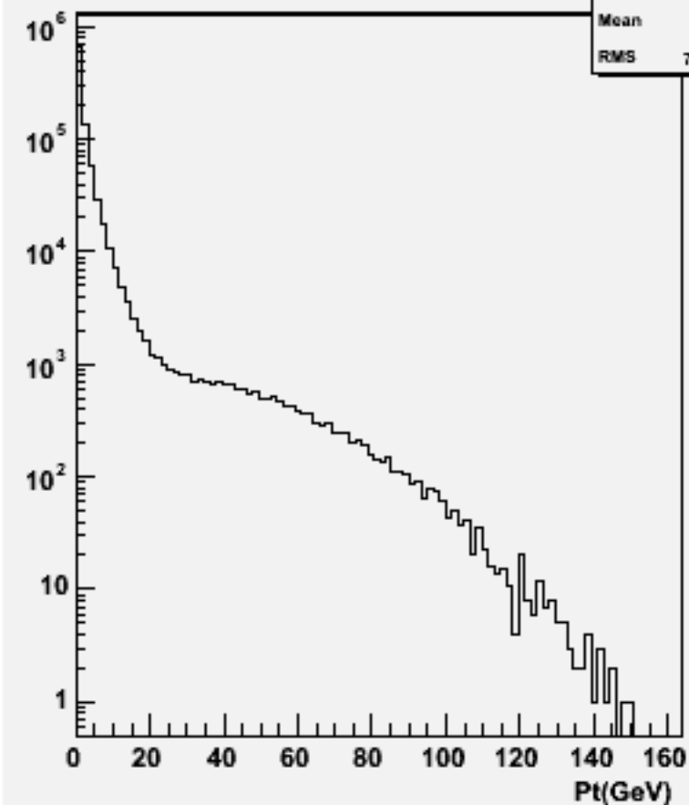
Particle Pt : w102096 n3n3ccbb_o
