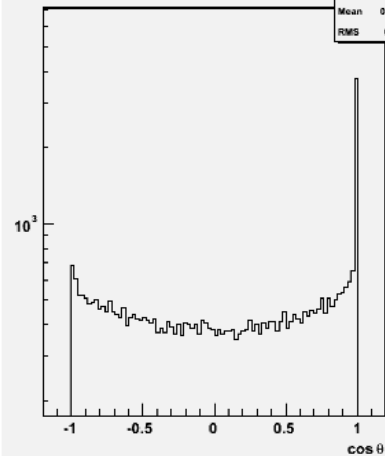
Jet cosθ (All jets)w102096 n3n3ccbb_o
