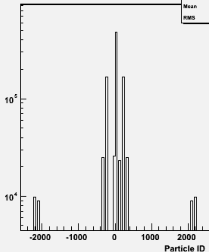
Particle ID : w102096 n3n3ccbb_o
