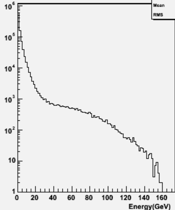
Particle Energy : w102096 n3n3ccbb_o
