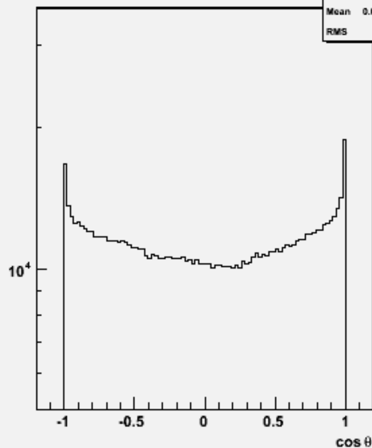
Particle cos \theta : w102096 n3n3ccbb_o
