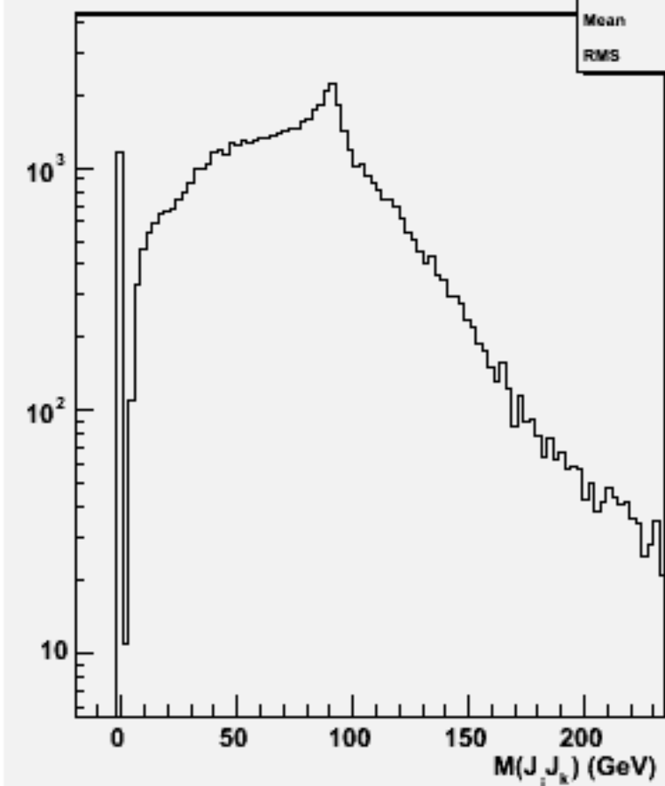
2jets mass(All comb)w102096 n3n3ccbb_o
