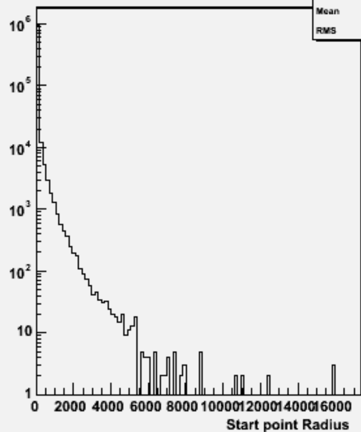
Start point R : w102096 n3n3ccbb_o
