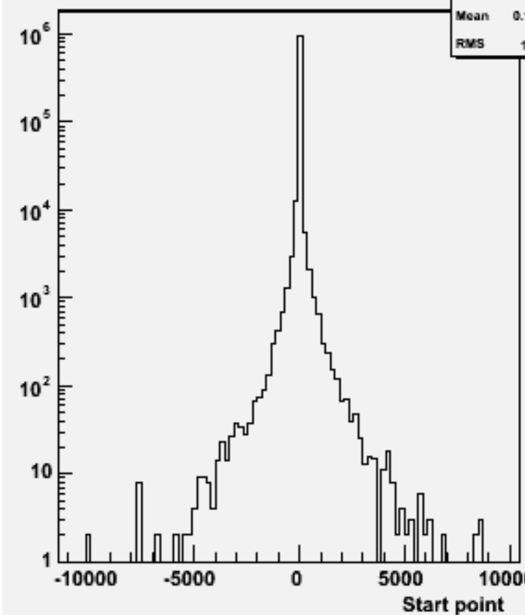
Start point Z : w102096 n3n3ccbb_o
