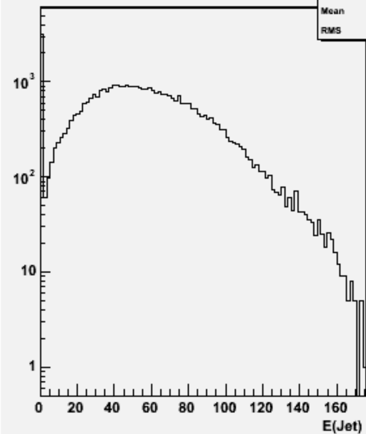
Jet energies(All jets)w102096 n3n3ccbb_o
