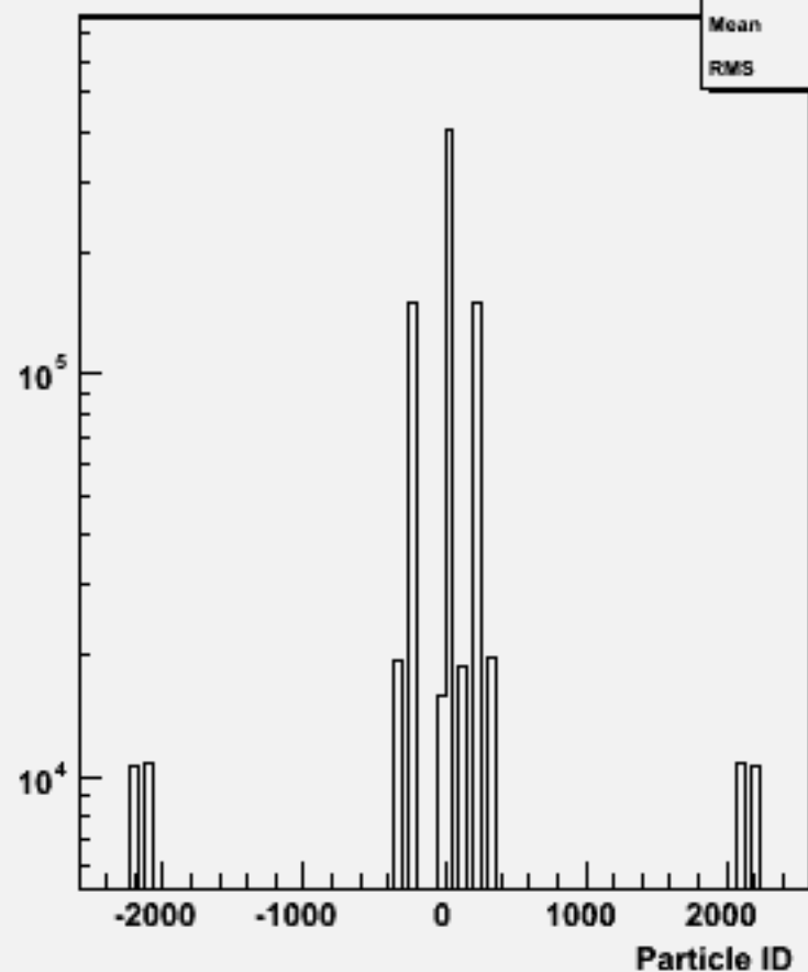
Particle ID : w102093 n3n3ccdd_o
