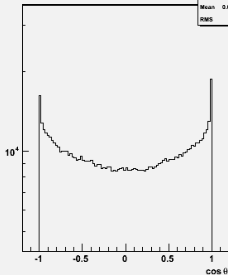
Particle cos \theta : w102093 n3n3ccdd_o
