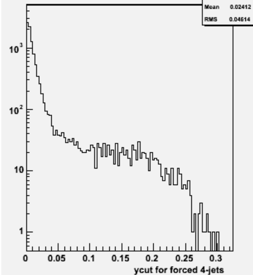
Ycut for 4-jets :w102093 n3n3ccdd_o
