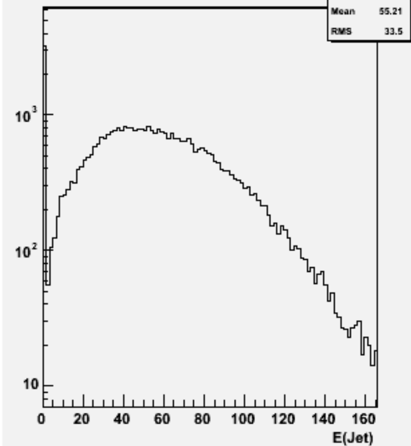
Jet energies(All jets)w102093 n3n3ccdd_o
