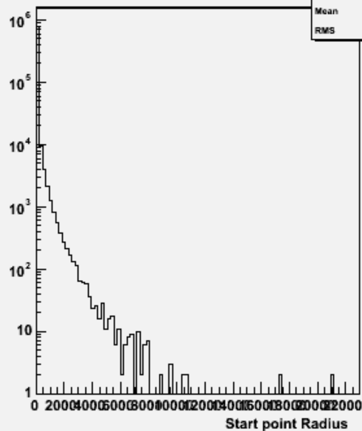
Start point R : w102093 n3n3ccdd_o
