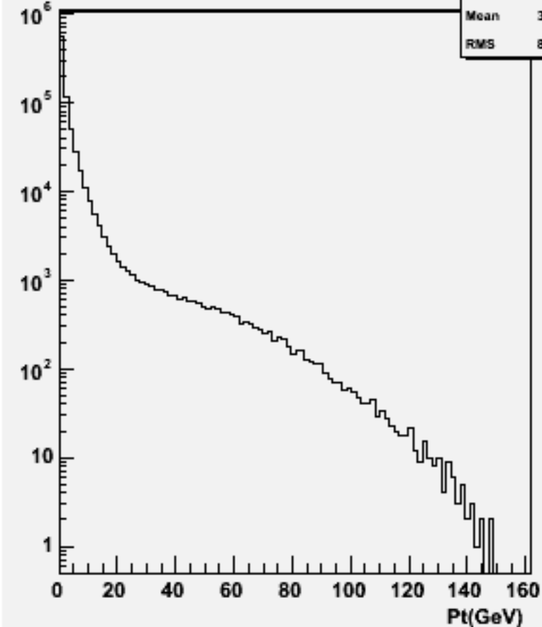
Particle Pt : w102093 n3n3ccdd_o
