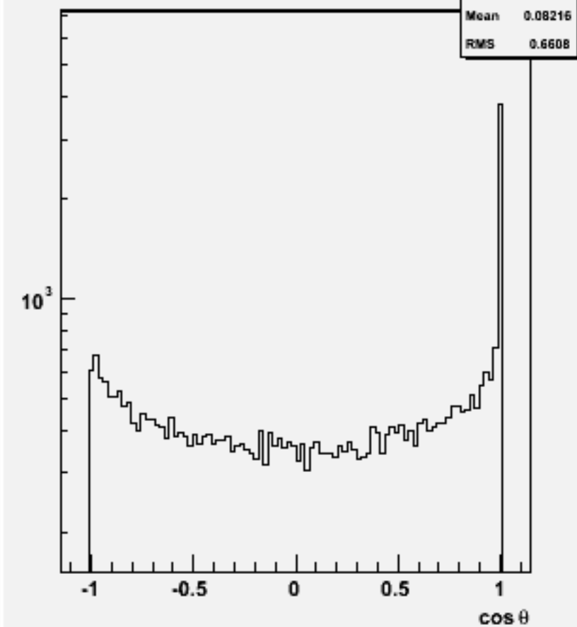
Jet cosθ (All jets)w102093 n3n3ccdd_o
