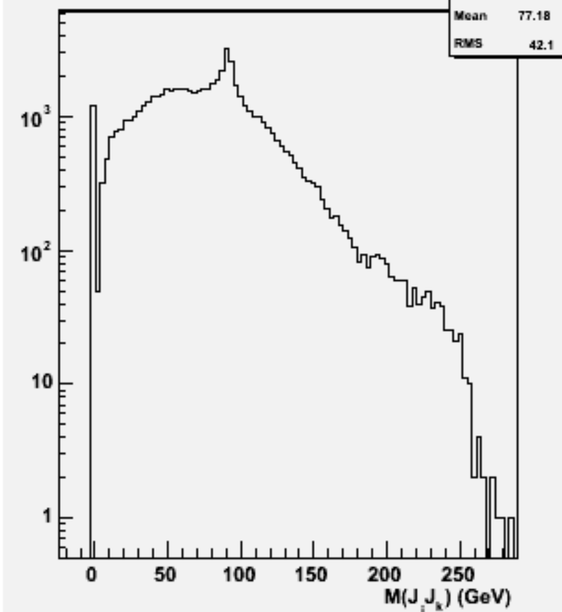
2jets mass(All comb)w102093 n3n3ccdd_o
