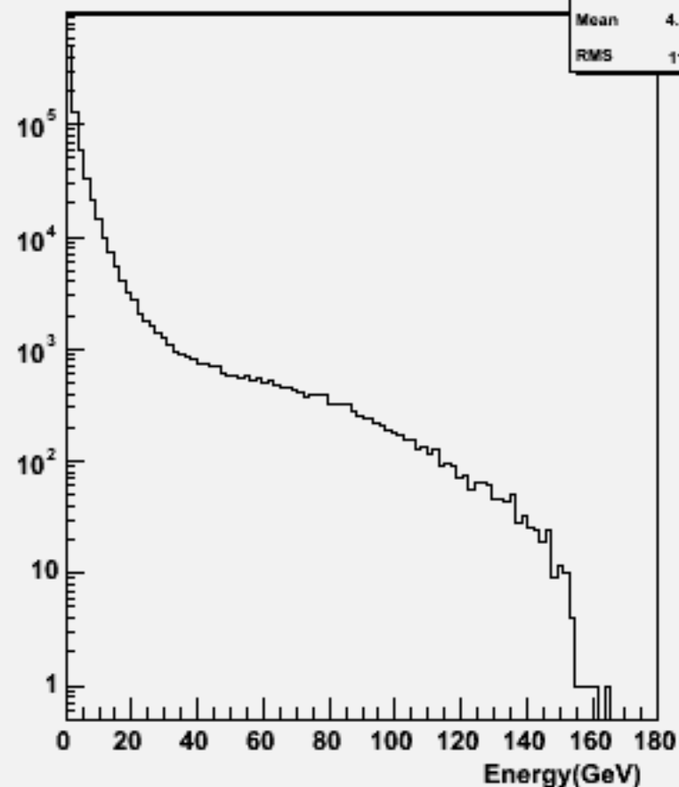
Particle Energy : w102093 n3n3ccdd_o
