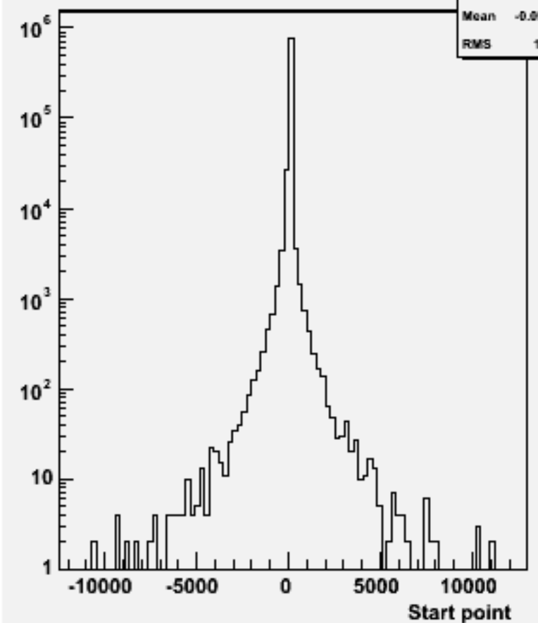
Start point Z : w102093 n3n3ccdd_o
