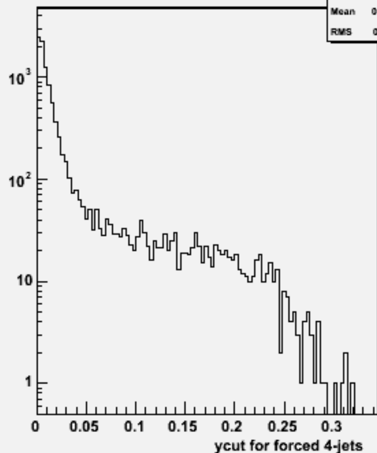
Ycut for 4-jets :w102092 n3n3ccdd_o
