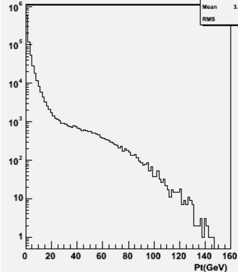
Particle Pt : w102092 n3n3ccdd_o
