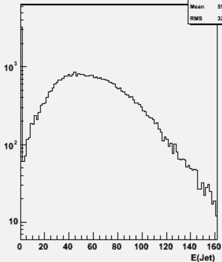
Jet energies(All jets)w102092 n3n3ccdd_o
