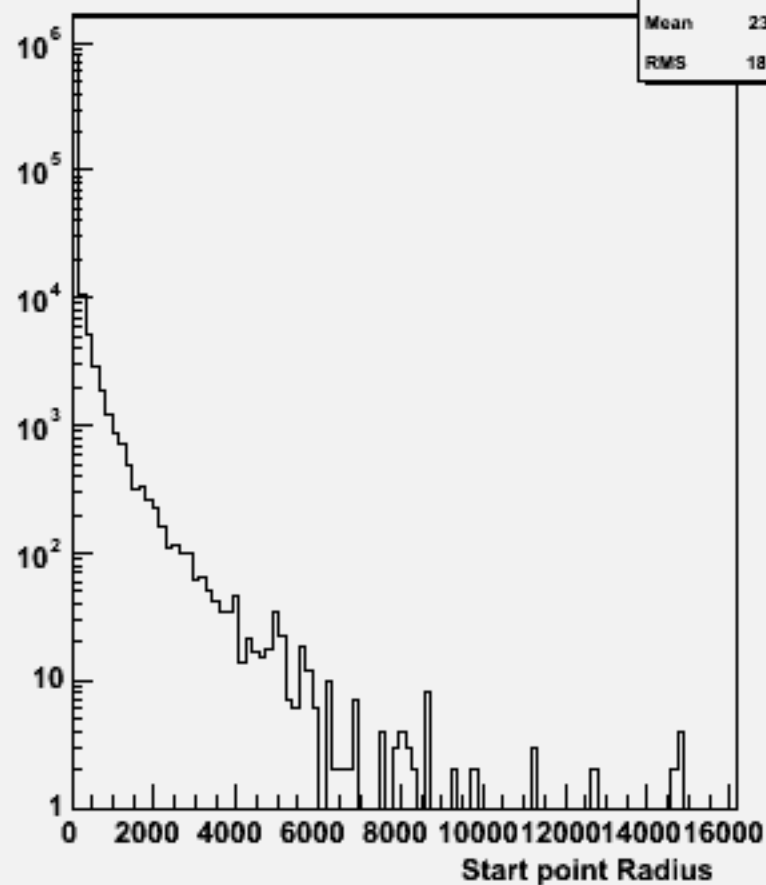
Start point R : w102092 n3n3ccdd_o
