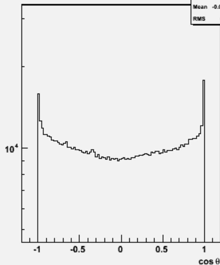
Particle cos \theta : w102092 n3n3ccdd_o
