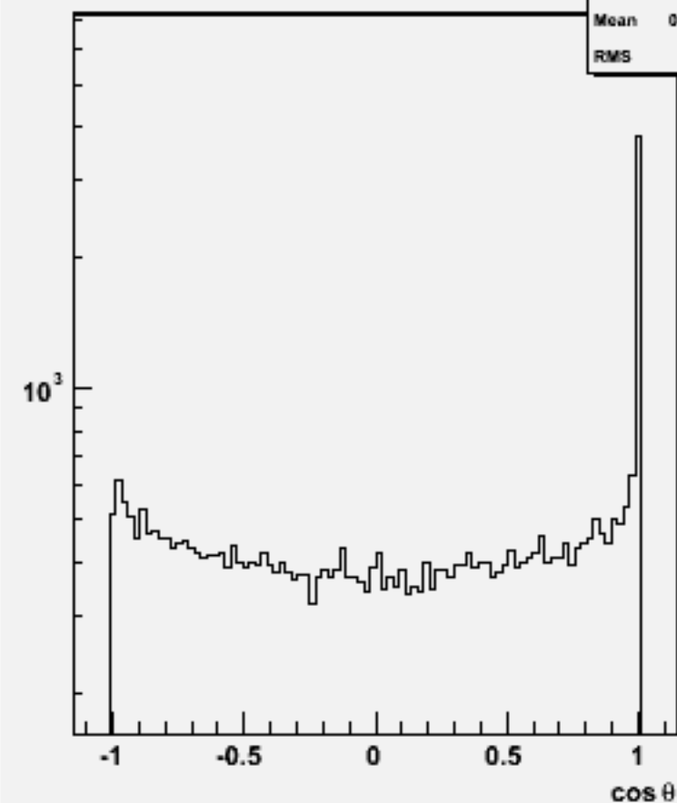
Jet cos \theta (All jets)w102092 n3n3ccdd_o
