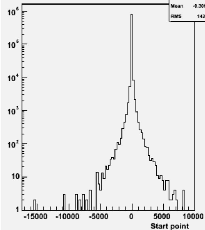
Start point Z : w102092 n3n3ccdd_o
