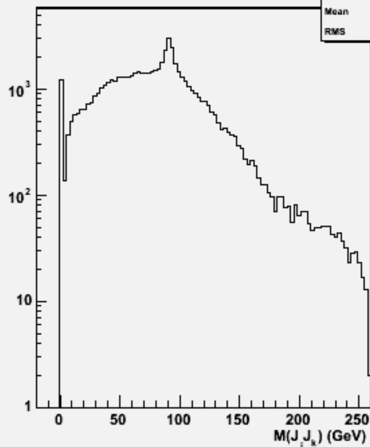
2jets mass(All comb)w102092 n3n3ccdd_o
