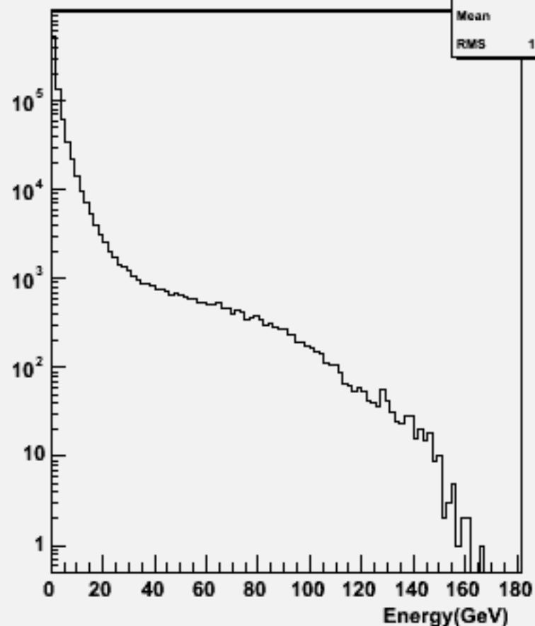
Particle Energy : w102092 n3n3ccdd_o
