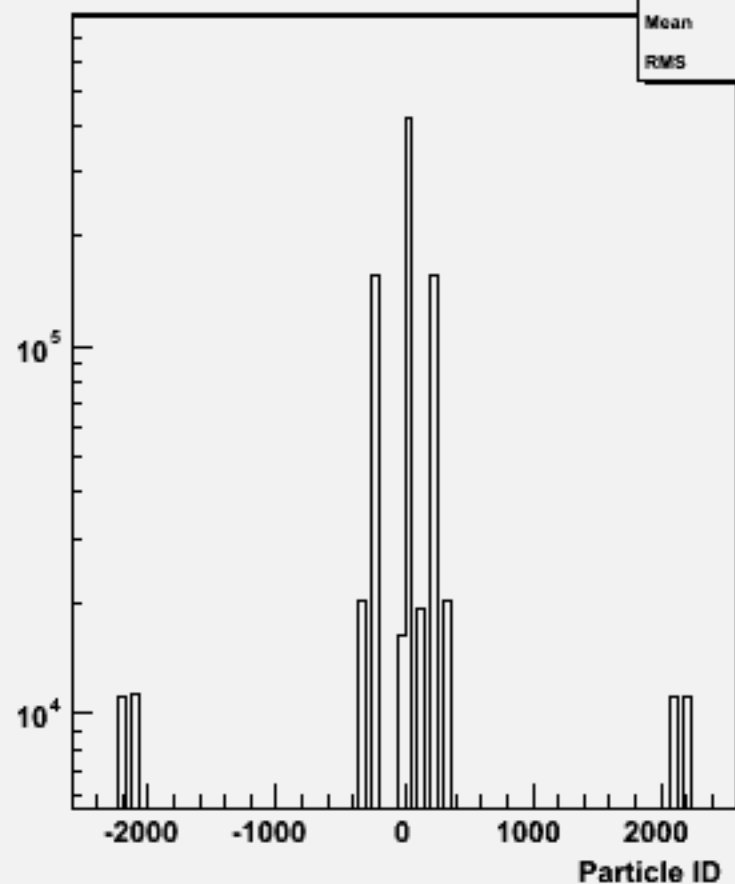
Particle ID : w102092 n3n3ccdd_o
