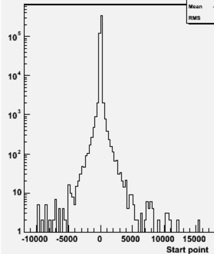
Start point Z : w102089 n3n3cce2e2_o
