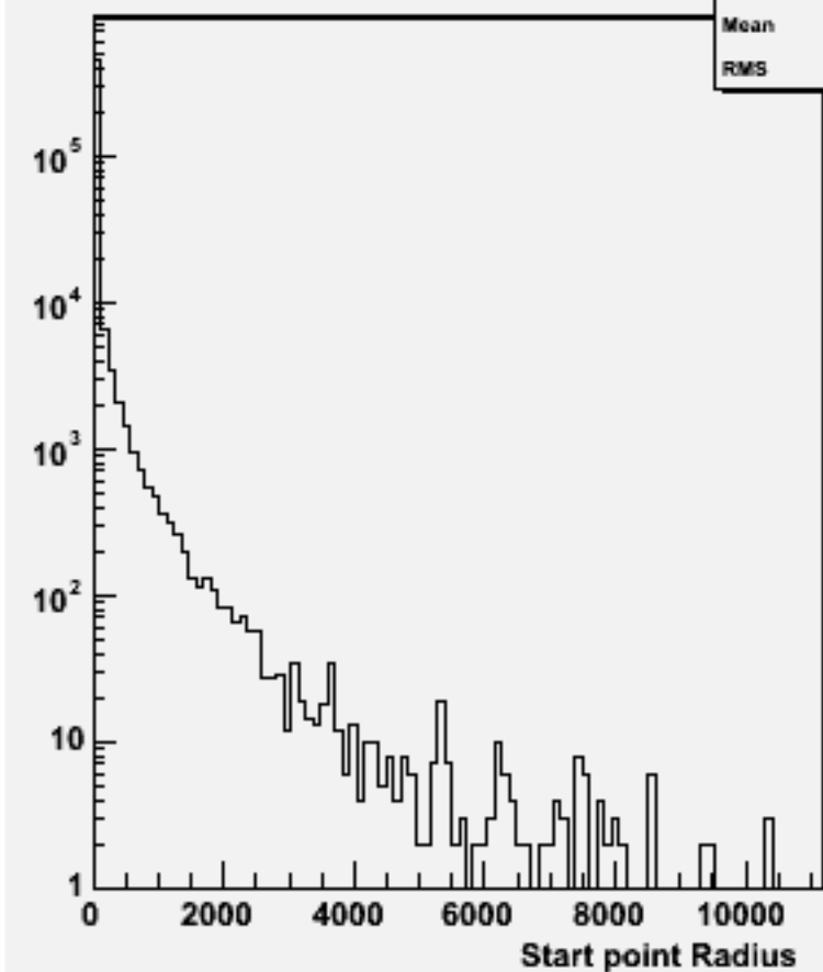
Start point R : w102089 n3n3cce2e2_o
