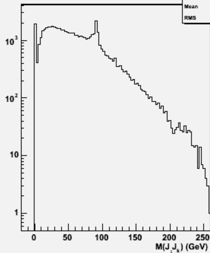
2jets mass(All comb)w102089 n3n3cce2e2_o
