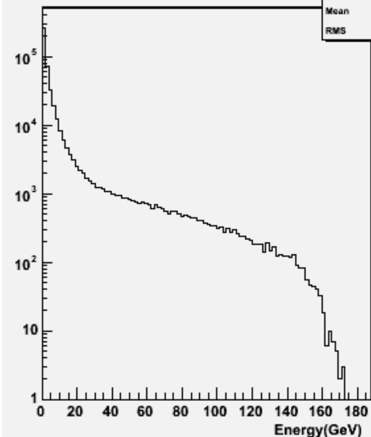
Particle Energy : w102089 n3n3cce2e2_o
