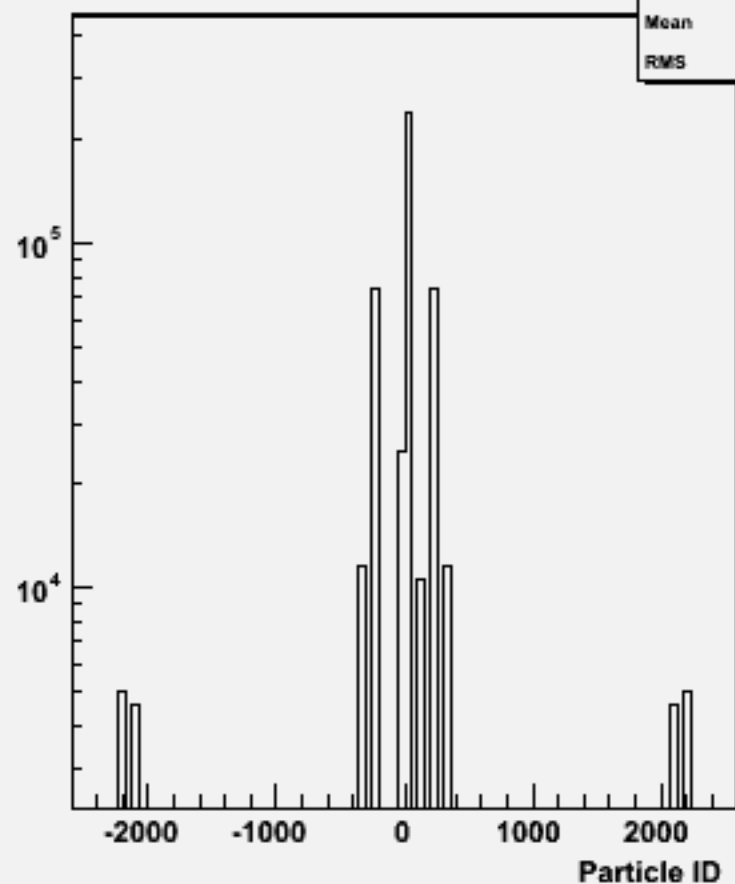
Particle ID : w102089 n3n3cce2e2_o
