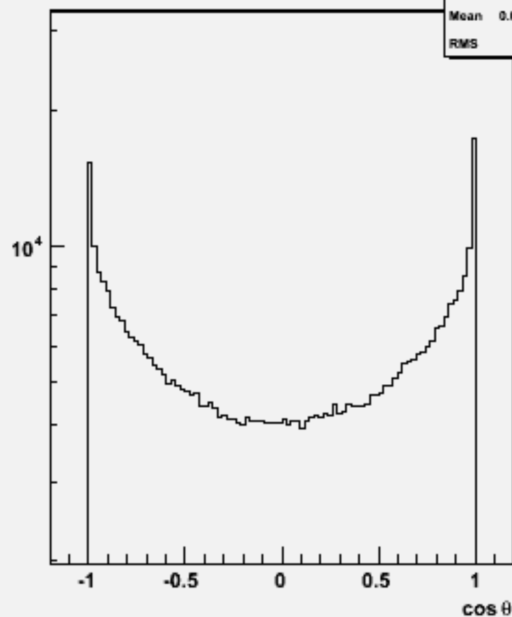
Particle cos θ : w102089 n3n3cce2e2_o
