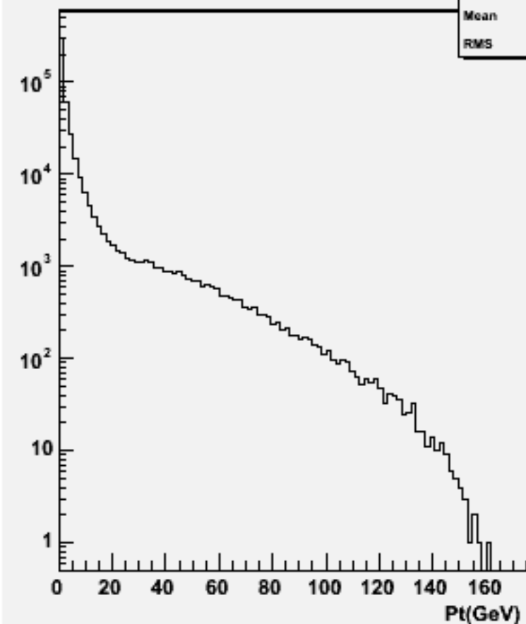
Particle Pt : w102089 n3n3cce2e2_o
