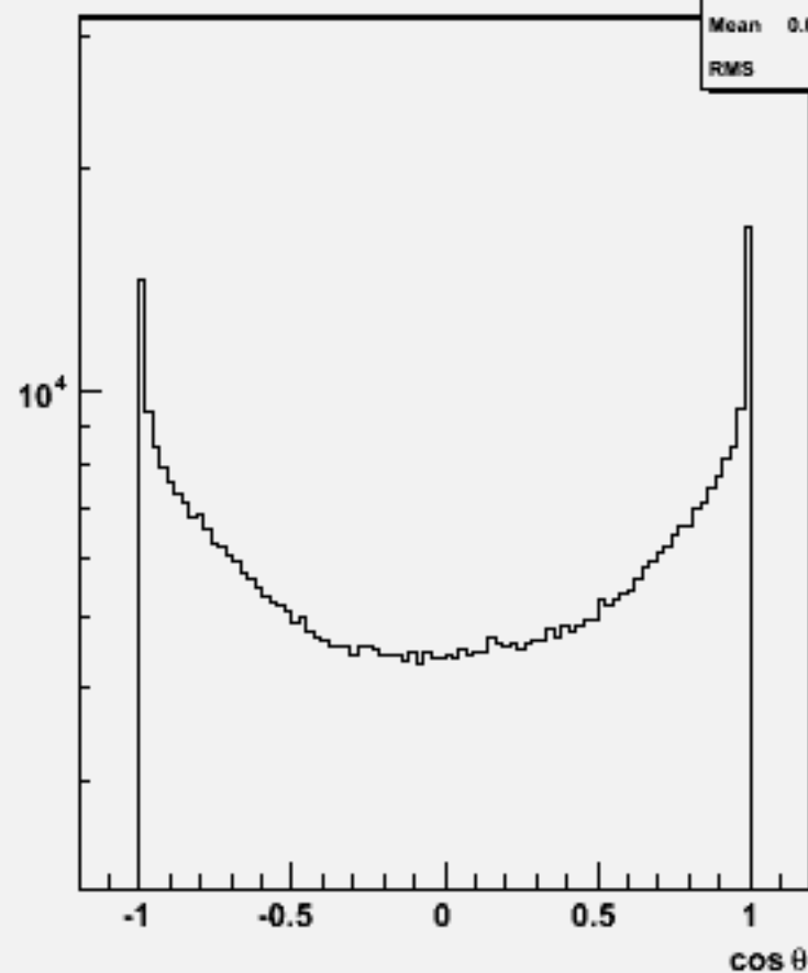
Particle \cos\theta : w102088 n3n3cce2e2_o
