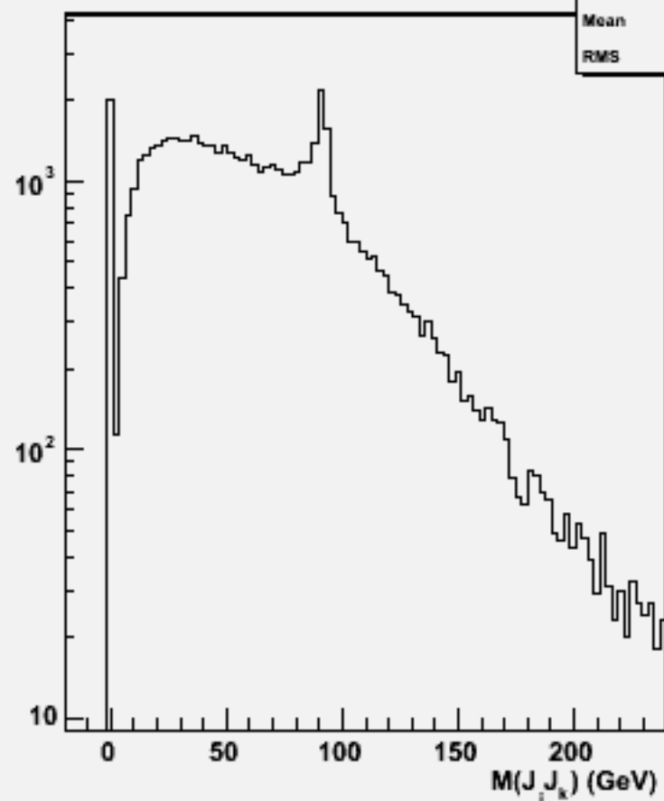
2jets mass(All comb)w102088 n3n3cce2e2_o
