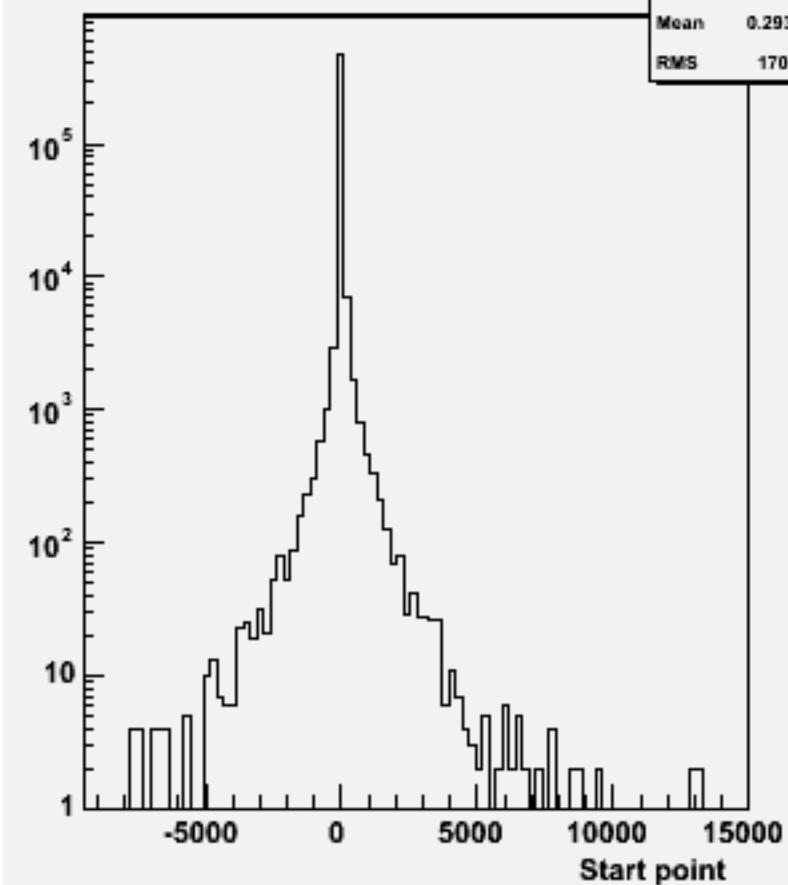
Start point Z : w102088 n3n3cce2e2_o
