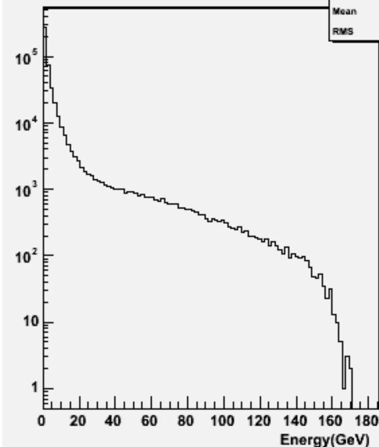
Start point R : w102088 n3n3cce2e2_o
