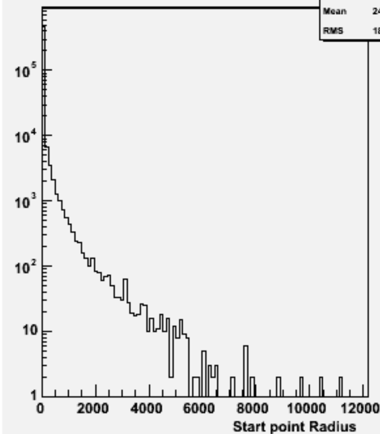
Start point R : w102088 n3n3cce2e2_o
