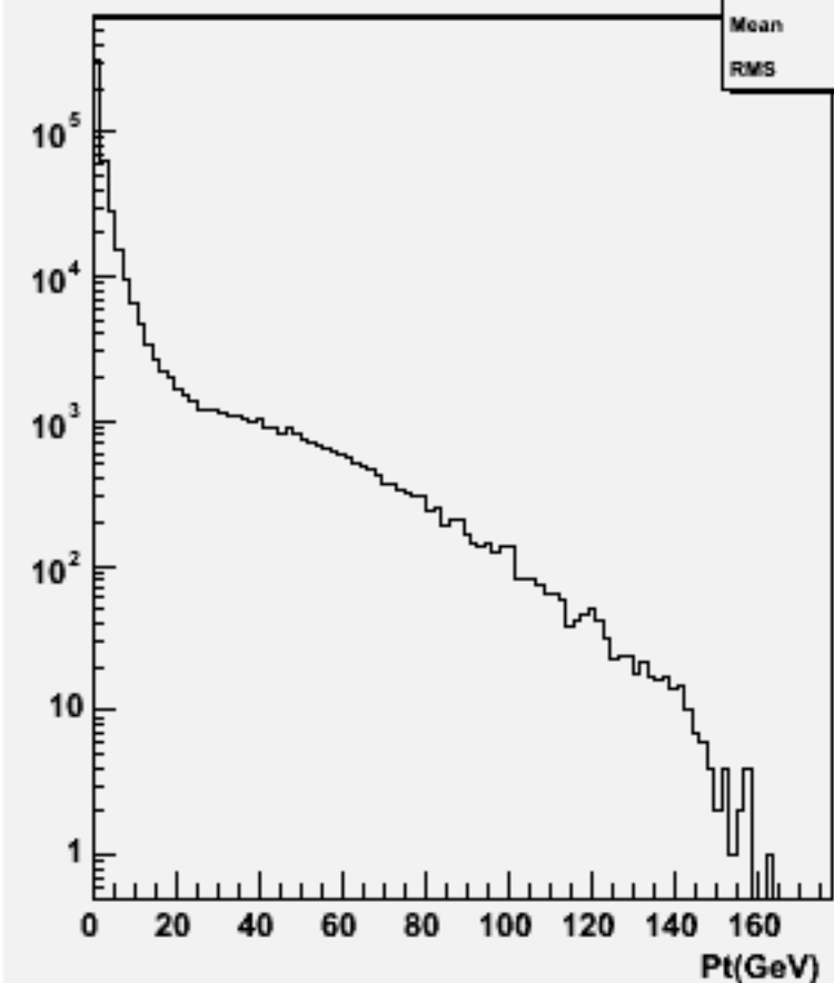
Start point Z : w102088 n3n3cce2e2_o
