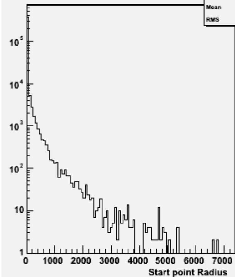
Start point R : w102086 n3n3cce1e1_o
