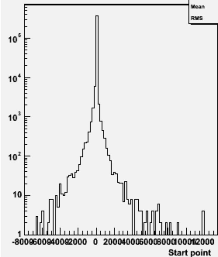
Start point Z : w102086 n3n3cce1e1_o
