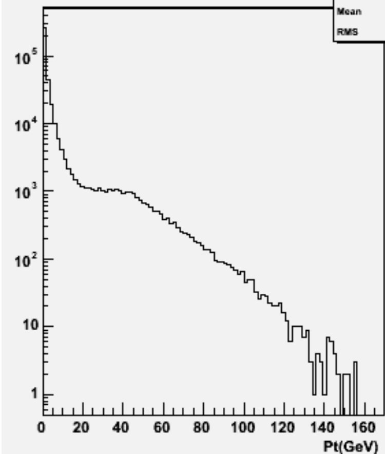
Particle Pt : w102086 n3n3cce1e1_o
