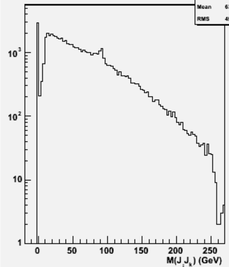
2jets mass(All comb)w102086 n3n3cce1e1_o
