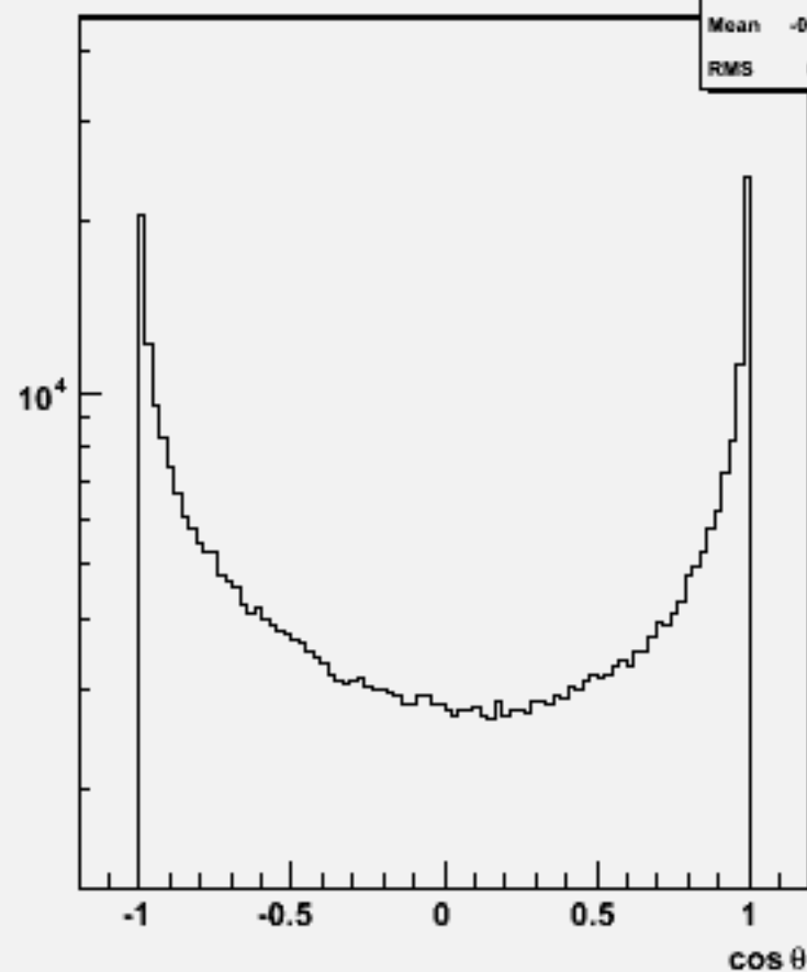
Particle \cos\theta : w102086 n3n3cce1e1_o
