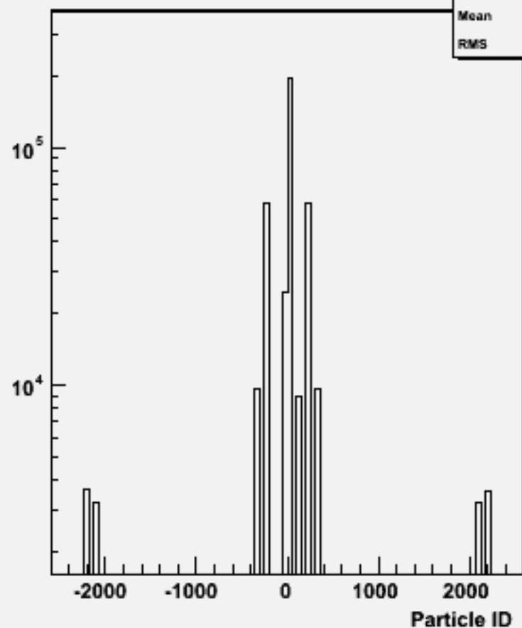
Particle ID : w102086 n3n3cce1e1_o
