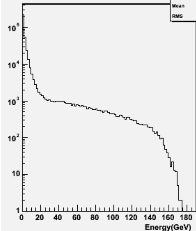
Particle Energy : w102086 n3n3cce1e1_o
