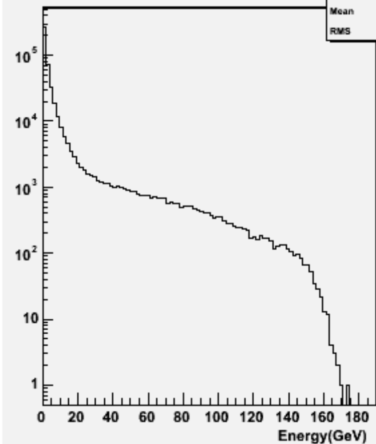
Particle Energy : w102084 n3n3cce1e1_o
