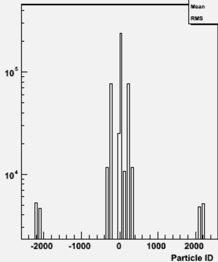
Particle ID : w102084 n3n3cce1e1_o
