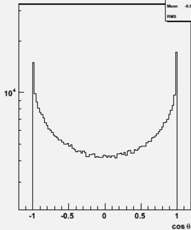
Particle cos \theta : w102084 n3n3cce1e1_o
