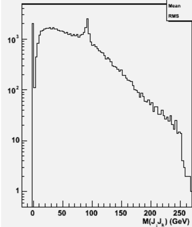
2jets mass(All comb)w102084 n3n3cce1e1_o
