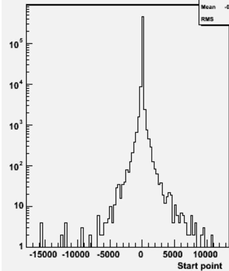
Start point Z : w102084 n3n3cce1e1_o
