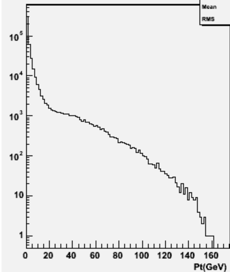
Particle Pt : w102084 n3n3cce1e1_o
