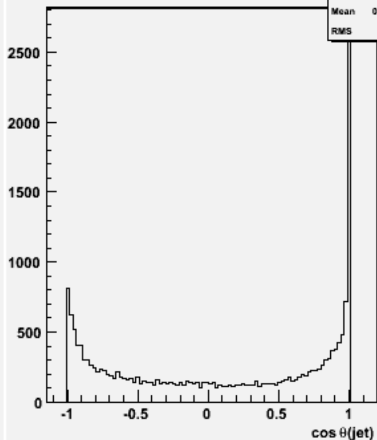
cos \theta for 2-jets :w102084 n3n3cce1e1_o
