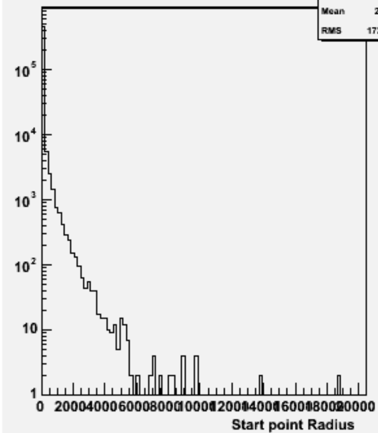
Start point R : w102084 n3n3cce1e1_o
